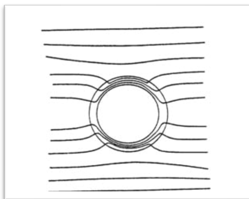
Figura 9: andamento qualitativo della deformazione delle linee di forza di un campo magnetico uniforme per effetto di un nucleo in materiale ferromagnetico
