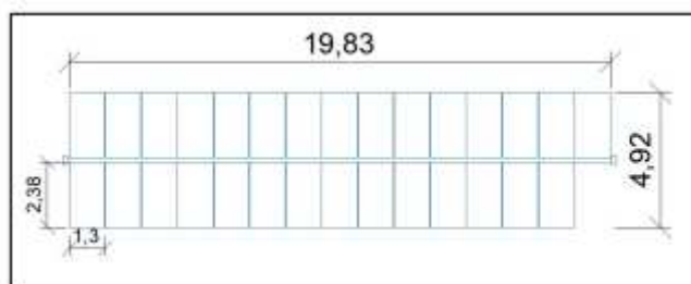
Figura 11 Dimensione "tracker" 1x29 con moduli VERTEX 670W – TSM-DEG21C.20
