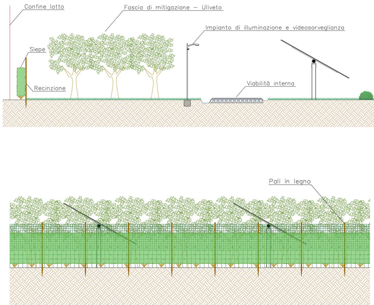
Figura 74 - Fascia di mitigazione tipo -sezione viabilità interna e prospetto recinzione
