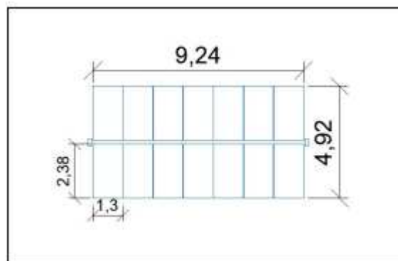
Figura 13 Dimensione "tracker" 1x14 con moduli VERTEX 670W – TSM-DEG21C.20
