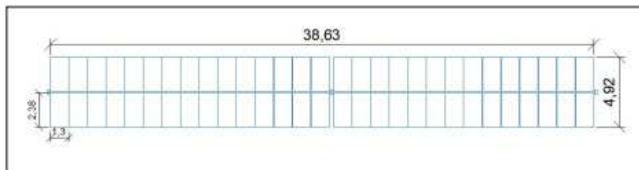
Figura 10 - Dimensione "tracker" 2x29 con moduli VERTEX 670W – TSM-DEG21C.20
