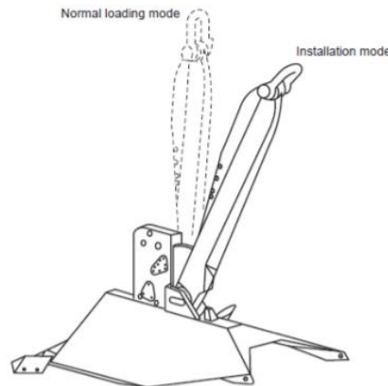
Figura 5.7: Variazione Angolo 'Shank-Fluke' Installazione/Esercizio per Ancora Bruce Dennla VLA [4]
