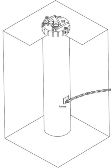
Figura 5.2: Tipica Connessione tra 'Suction Pile' e Linea di Ormeggio a Catenaria [7]
