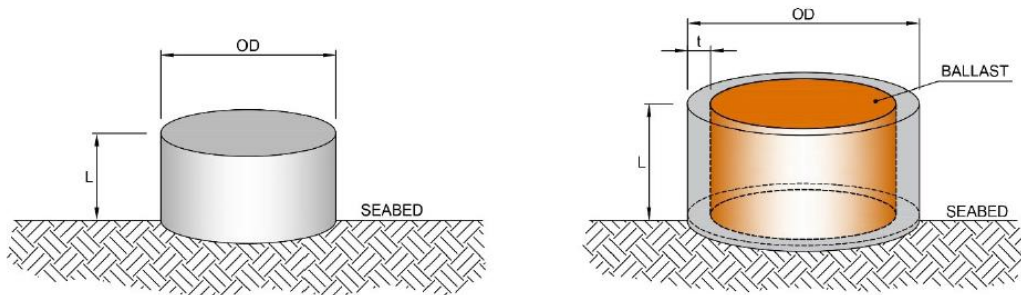
Figura 5.1: Schema Semplificato di Ancore a Gravità Piene (Sinistra) o Cave con Zavorra (Destra)
