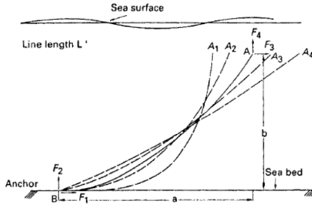
Figura 4.2: Sistema di Ormeggio con Catenaria [2]
