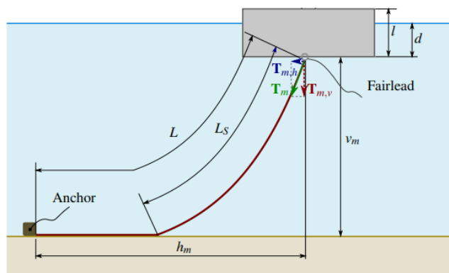
Figura 4.3: Catenaria
