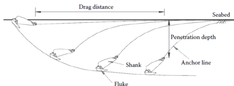
Figura 5.5: Schema di Installazione di Ancore a Trascinamento DEA [23]
