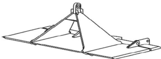
Figura 5.8: Esempio Schematico di Ancora a Piastra [3]
