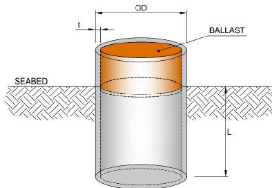
Figura 5.3: Schema Semplificato di Ancore Ibride
