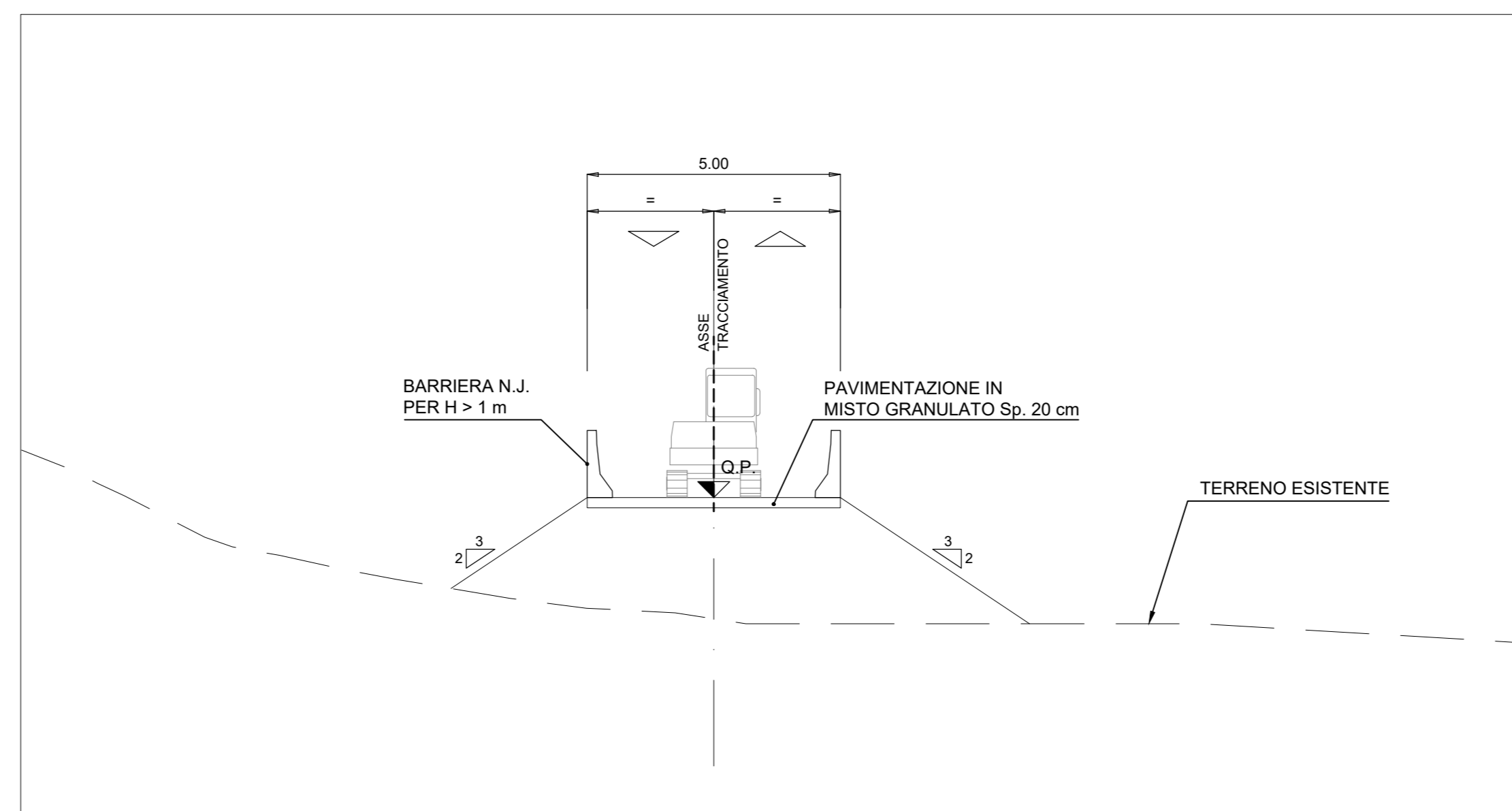
SEZIONE TPO scala 1:100
