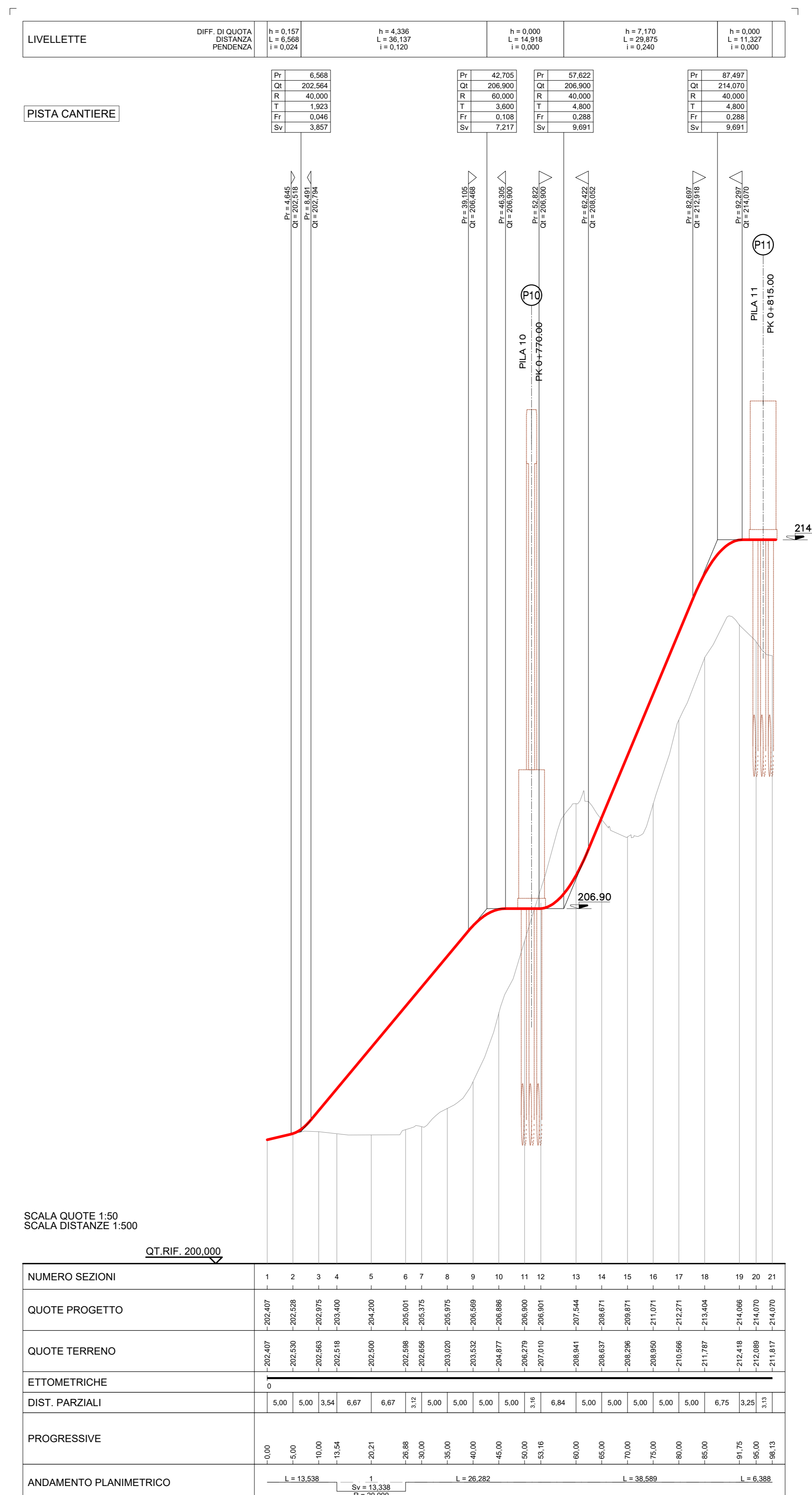
PROFILO LONGITUDINALE scala 1:500/50
