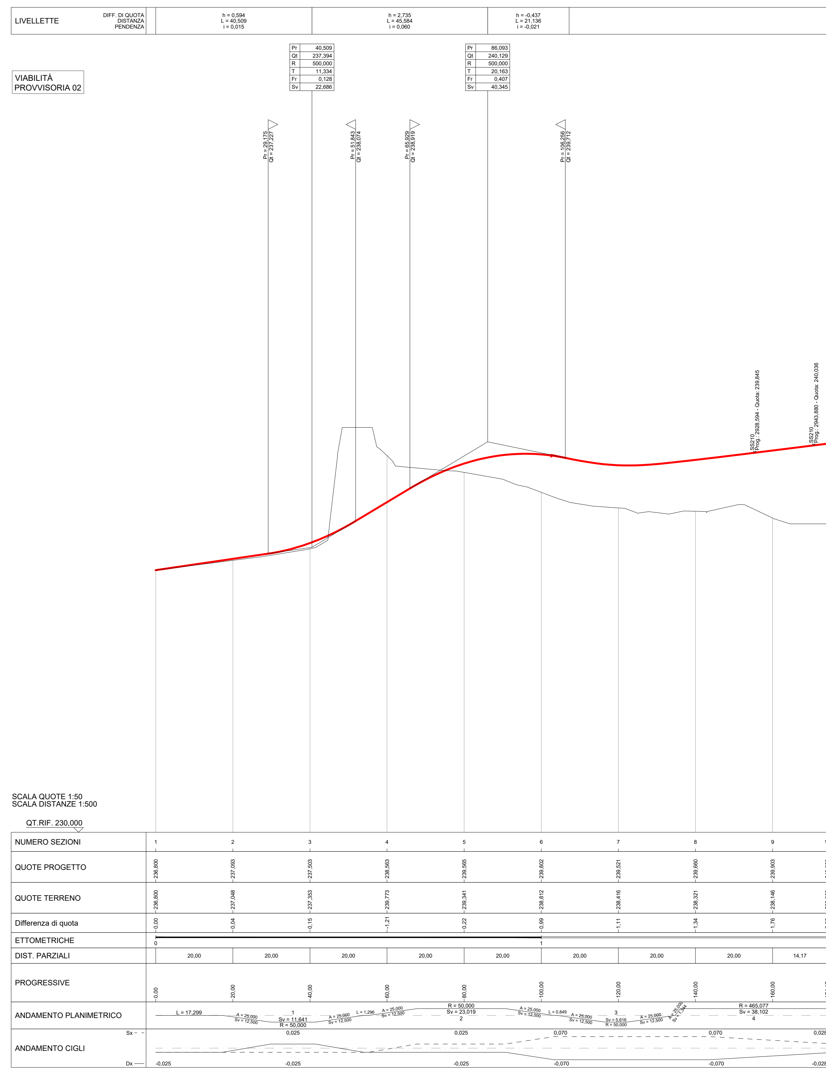
PROFILO LONGITUDINALE scala 1:500/50
