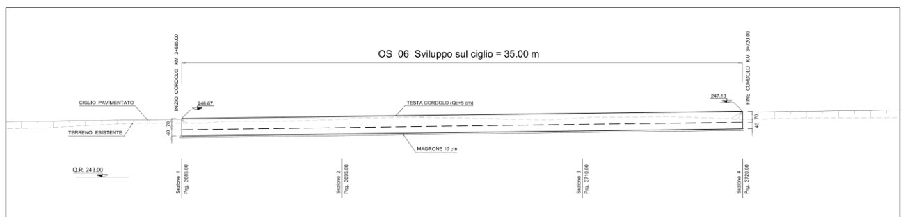
Figura 2 – Prospetto
