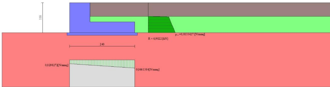
Diagramma delle pressioni (combinazione statica) (Combinazione n° 2)
