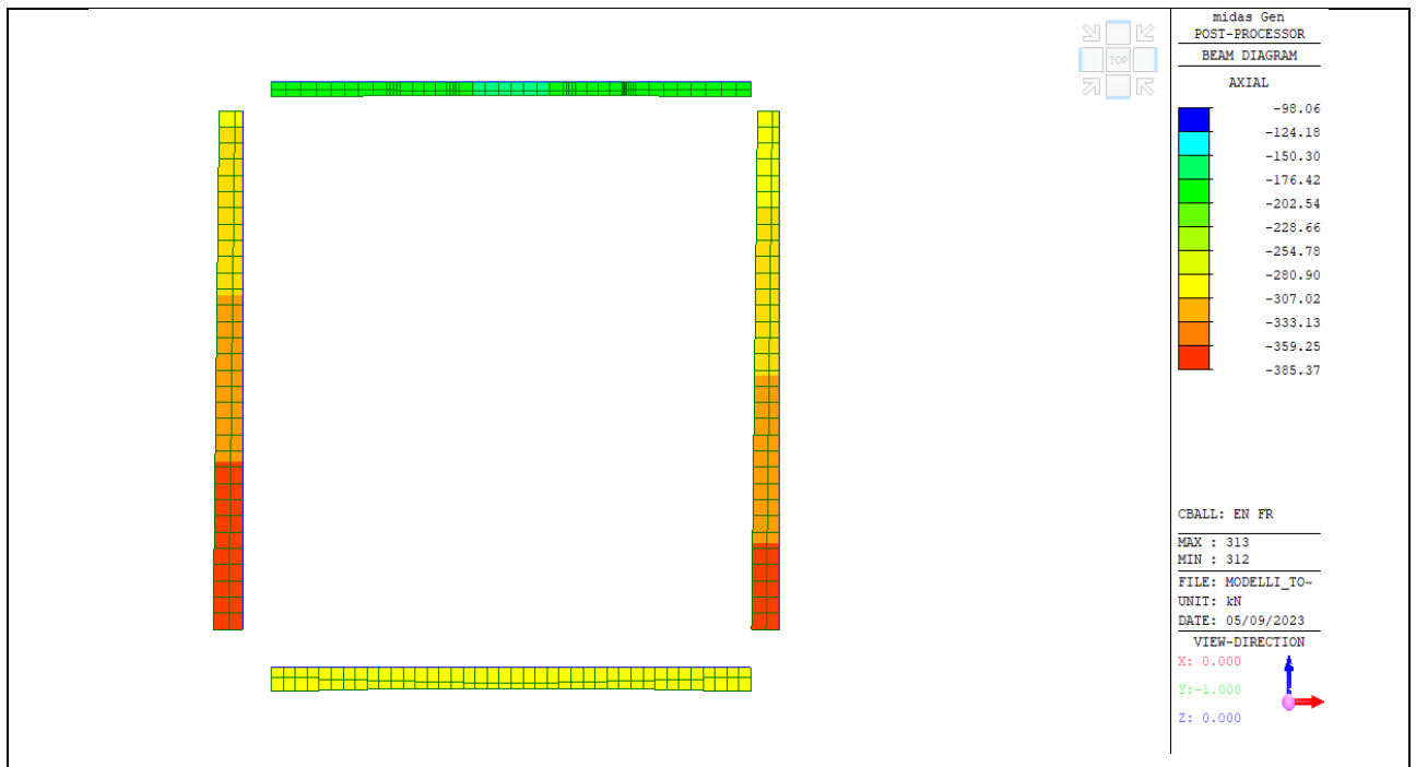
Figura 18: Azione assiale (kN) – Inviluppo FREQUENTE
