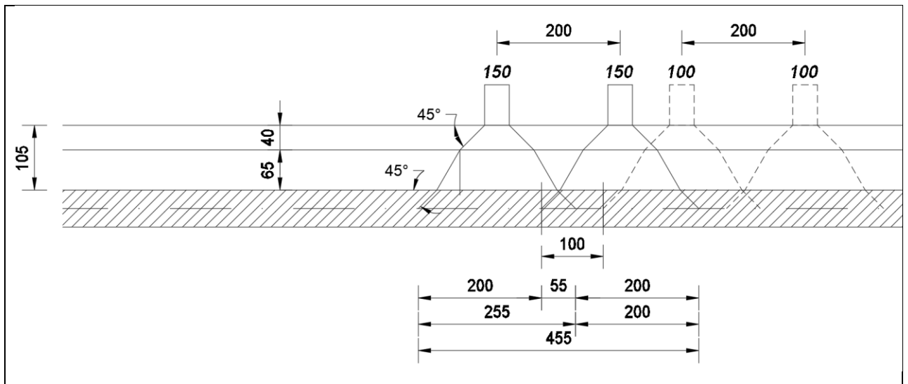
Figura 9: Diffusione longitudinale
