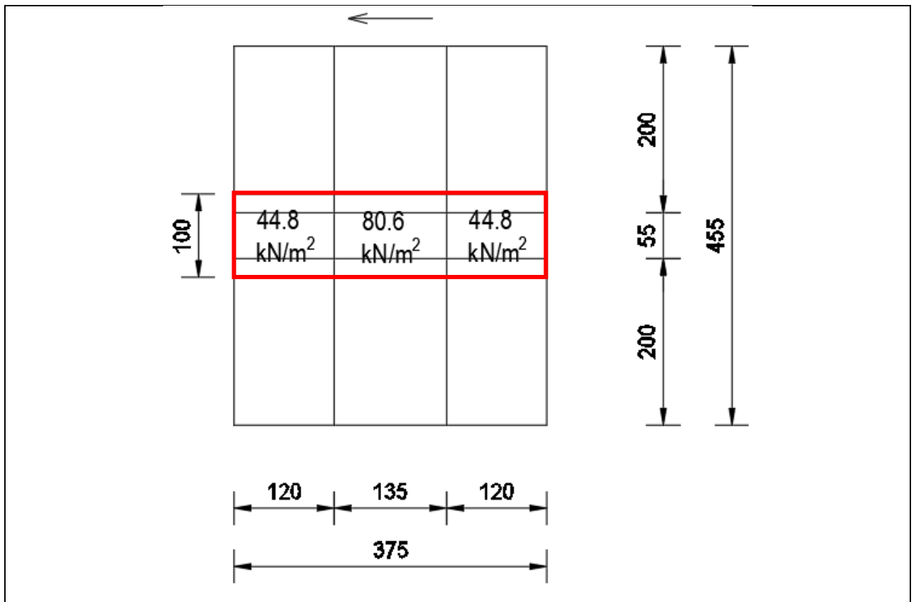
Figura 10: Valore del carico
