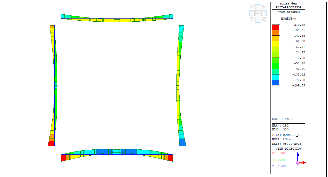
Figura 19: Momento flettente (kNm) – Inviluppo QUASI PERMANENTE
