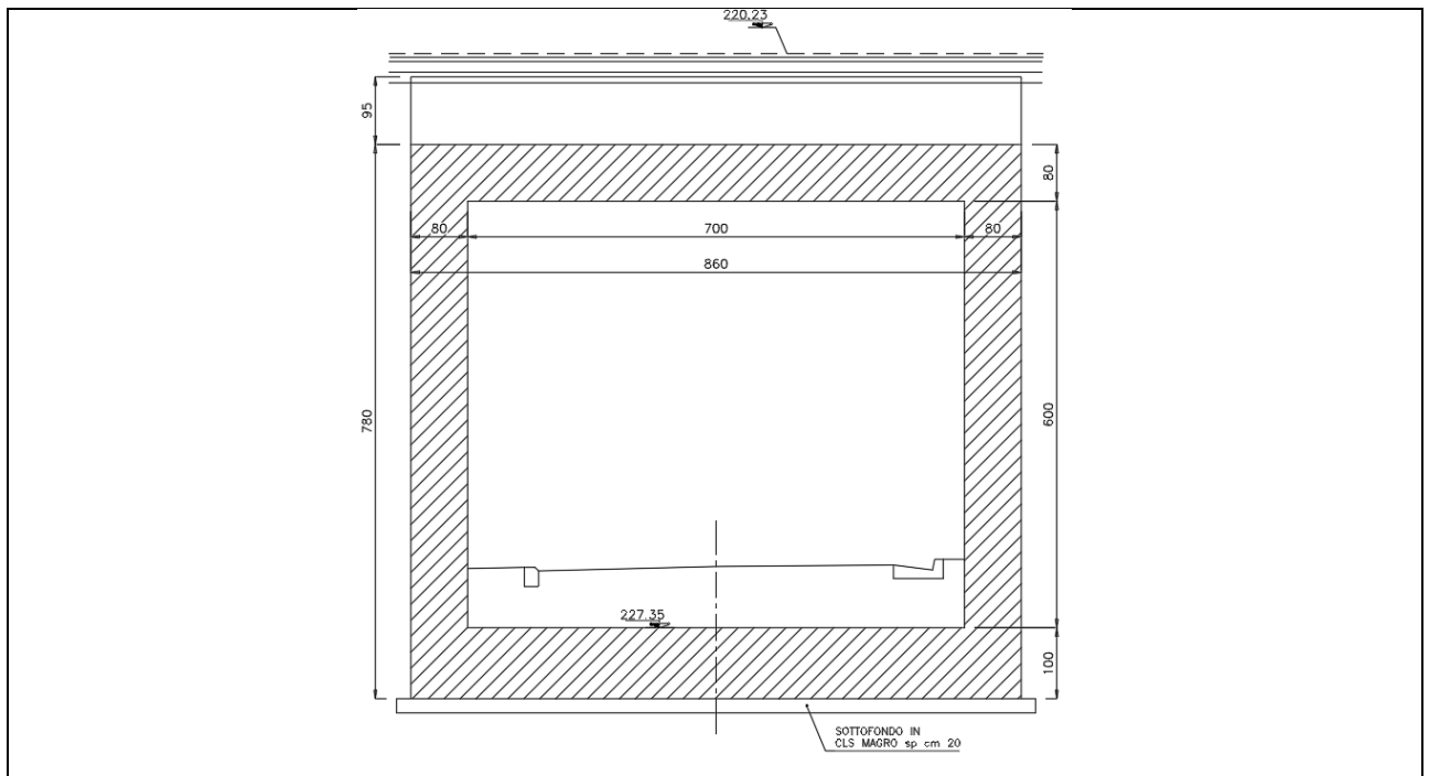
Figura 3: Sezione trasversale
