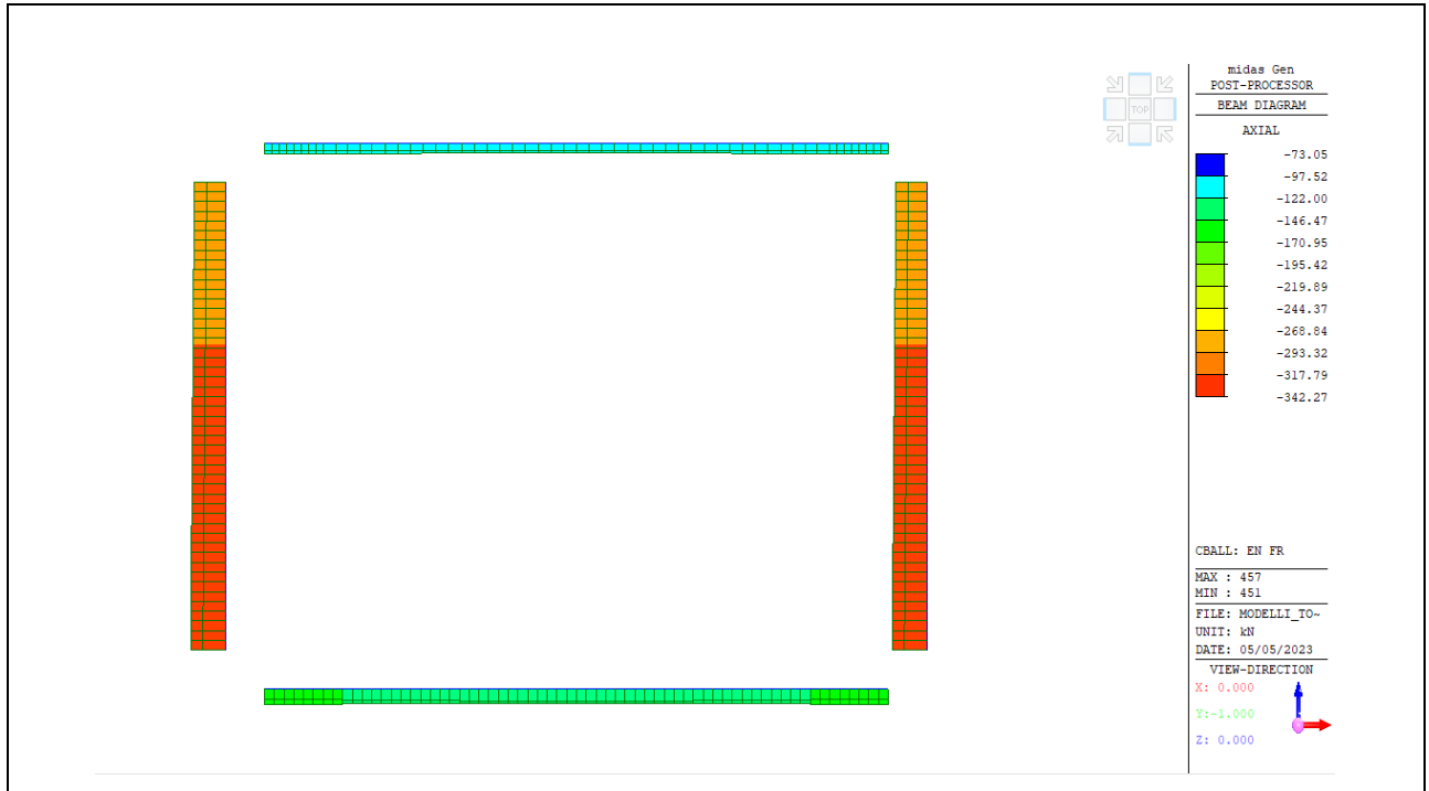
Figura 20: Azione assiale (kN) – Involuppo FREQUENTE
