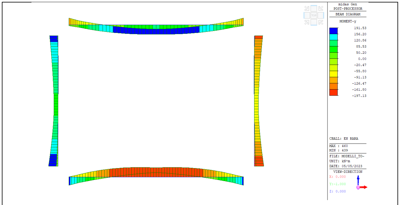
Figura 17: Momento flettente (kNm) – Involuppo RARA
