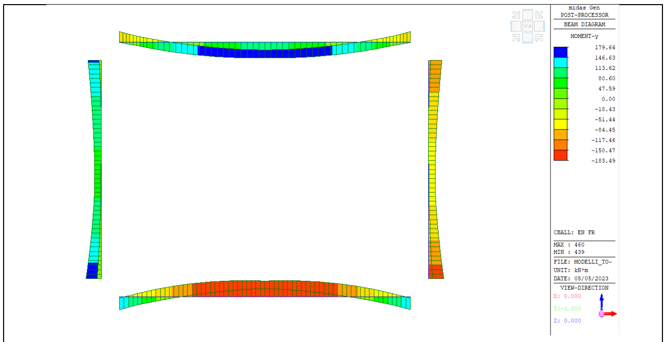
Figura 19: Momento flettente (kNm) – Involuppo FREQUENTE
