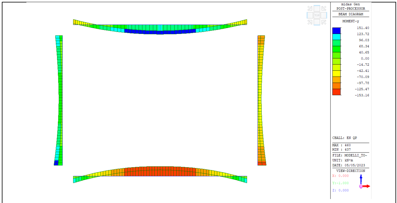
Figura 21: Momento flettente (kNm) – Involuppo QUASI PERMANENTE
