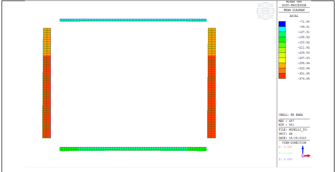
Figura 18: Azione assiale (kN) – Involuppo RARA
