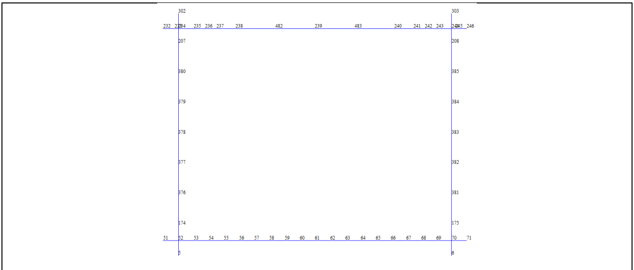
Figura 5: Numerazione nodi
