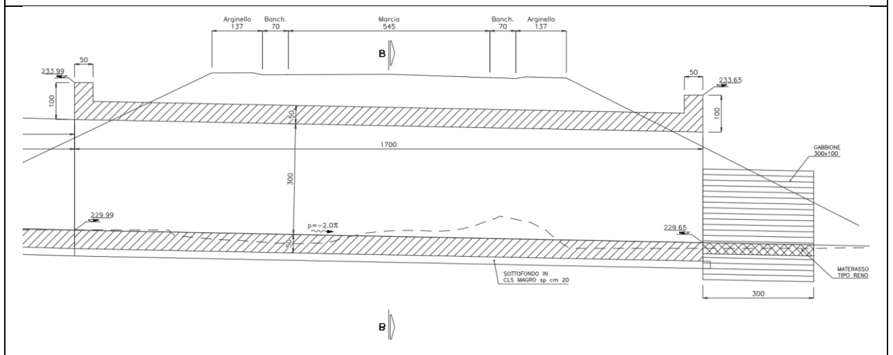
Figura 2: Sezione longitudinale
