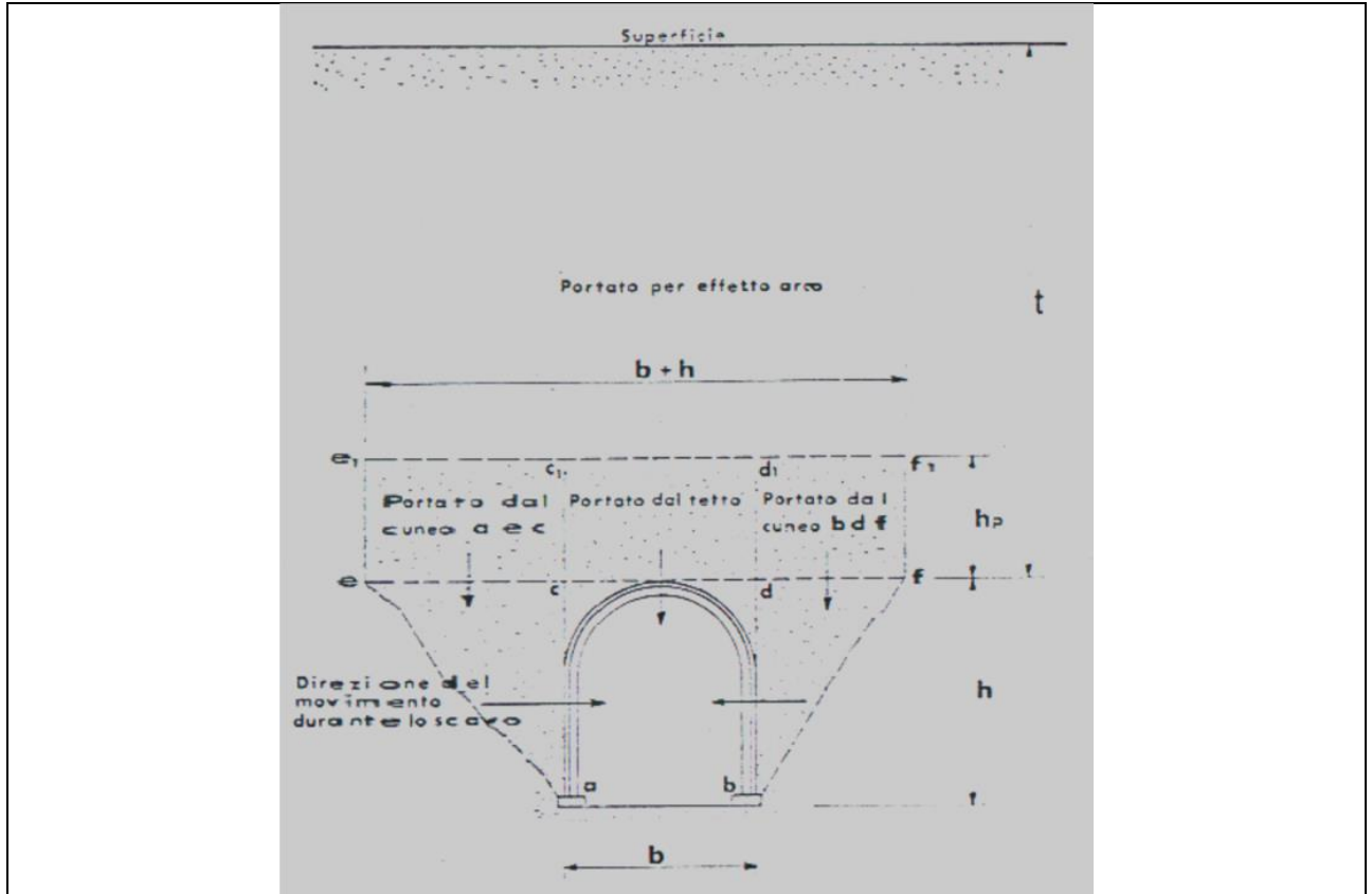
Figura 9: Modello di calcolo di Terzaghi
