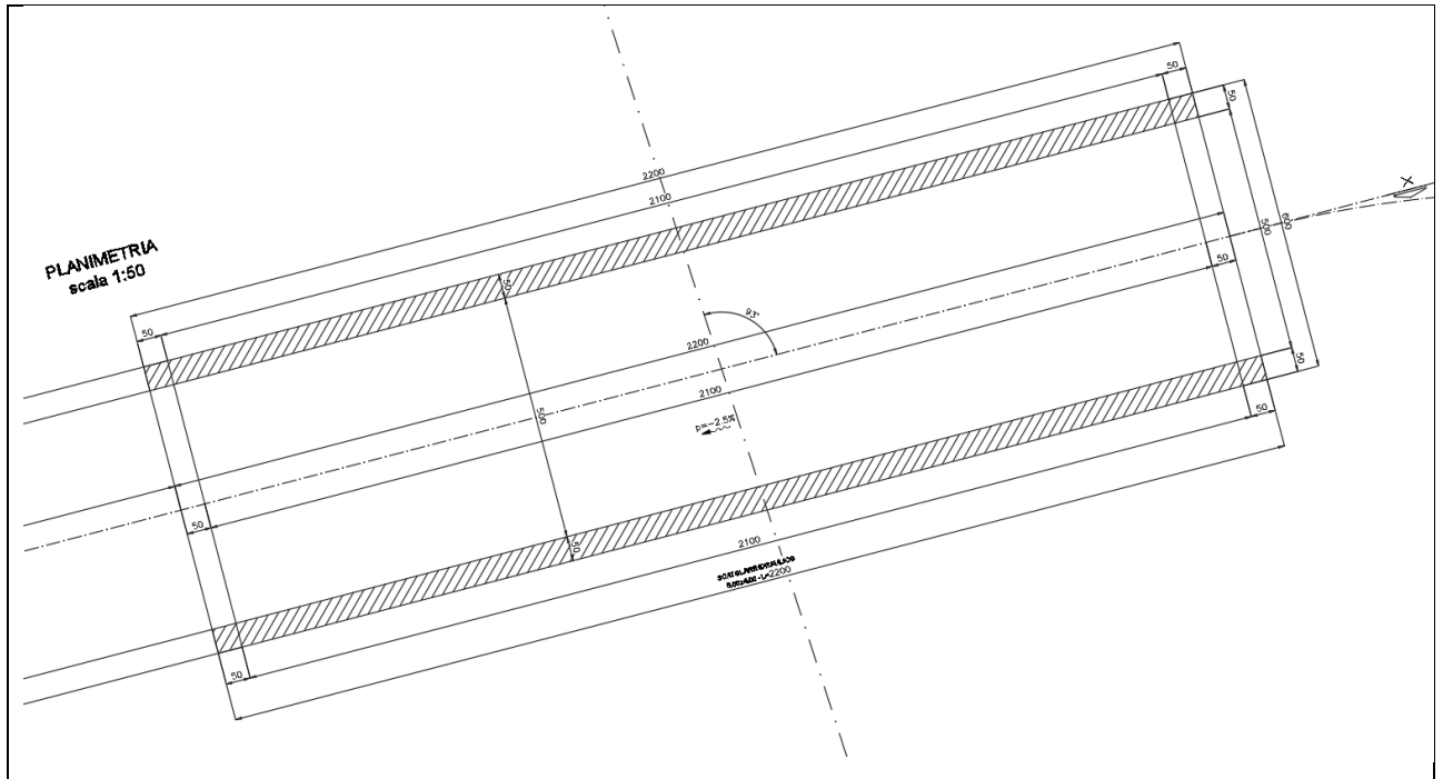
Figura 1: Stralcio planimetrico
