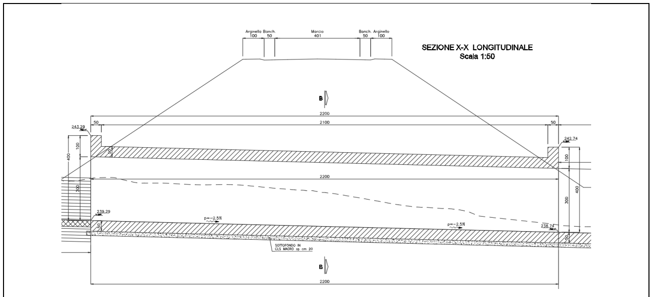
Figura 2: Sezione longitudinale
