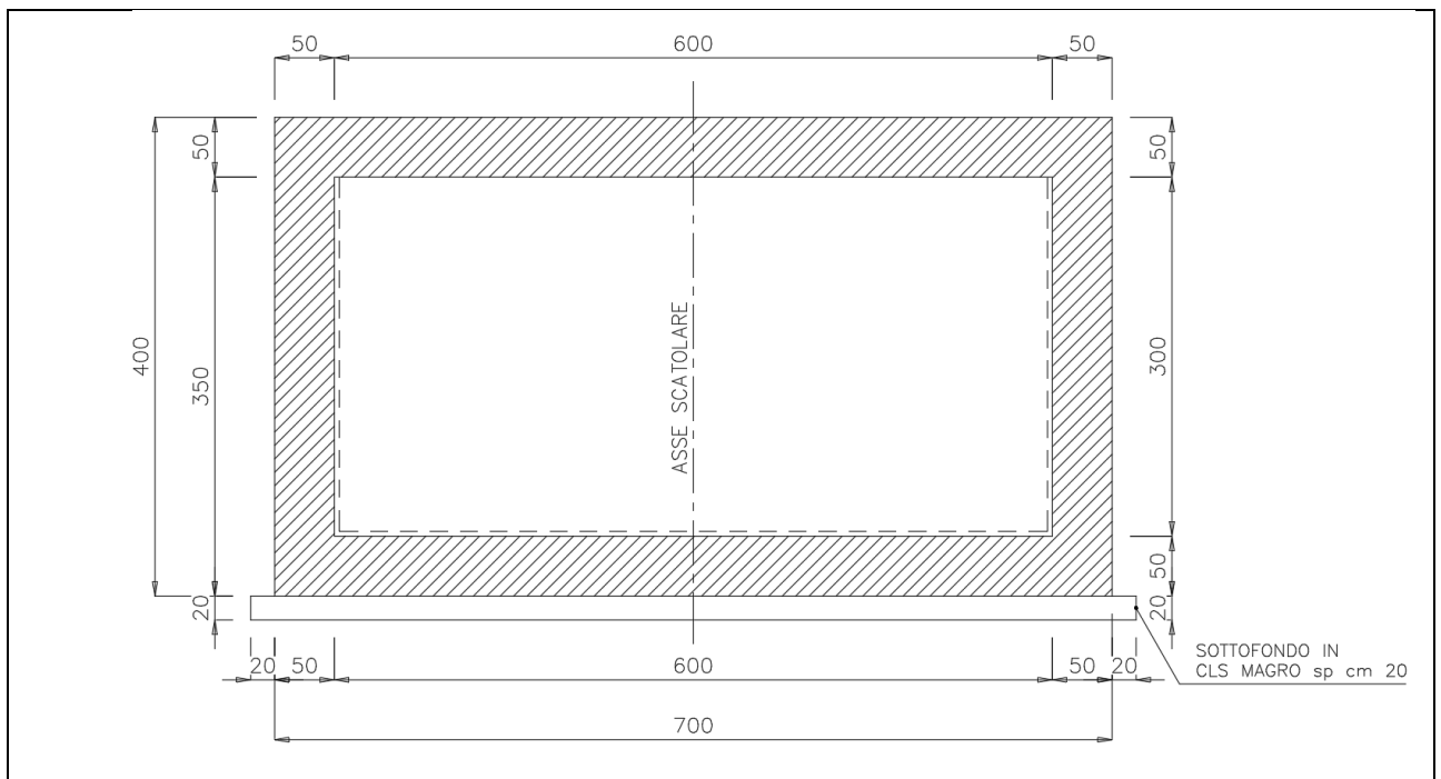
Figura 3: Sezione trasversale
