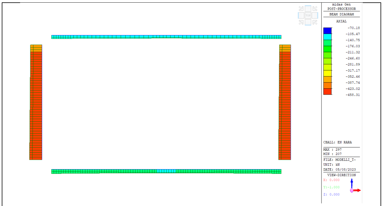
Figura 16: Azione assiale (kN) – Involuppo RARA
