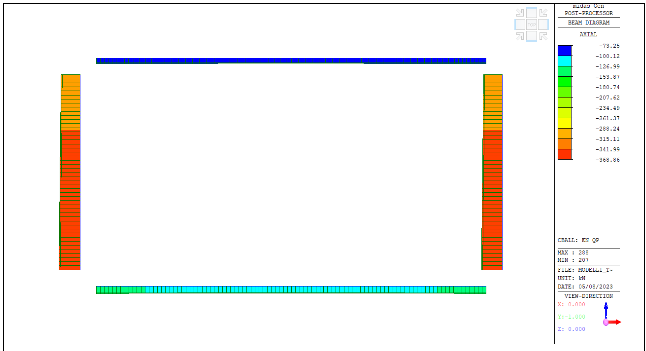
Figura 20: Azione assiale (kN) – Involuppo QUASI PERMANENTE
