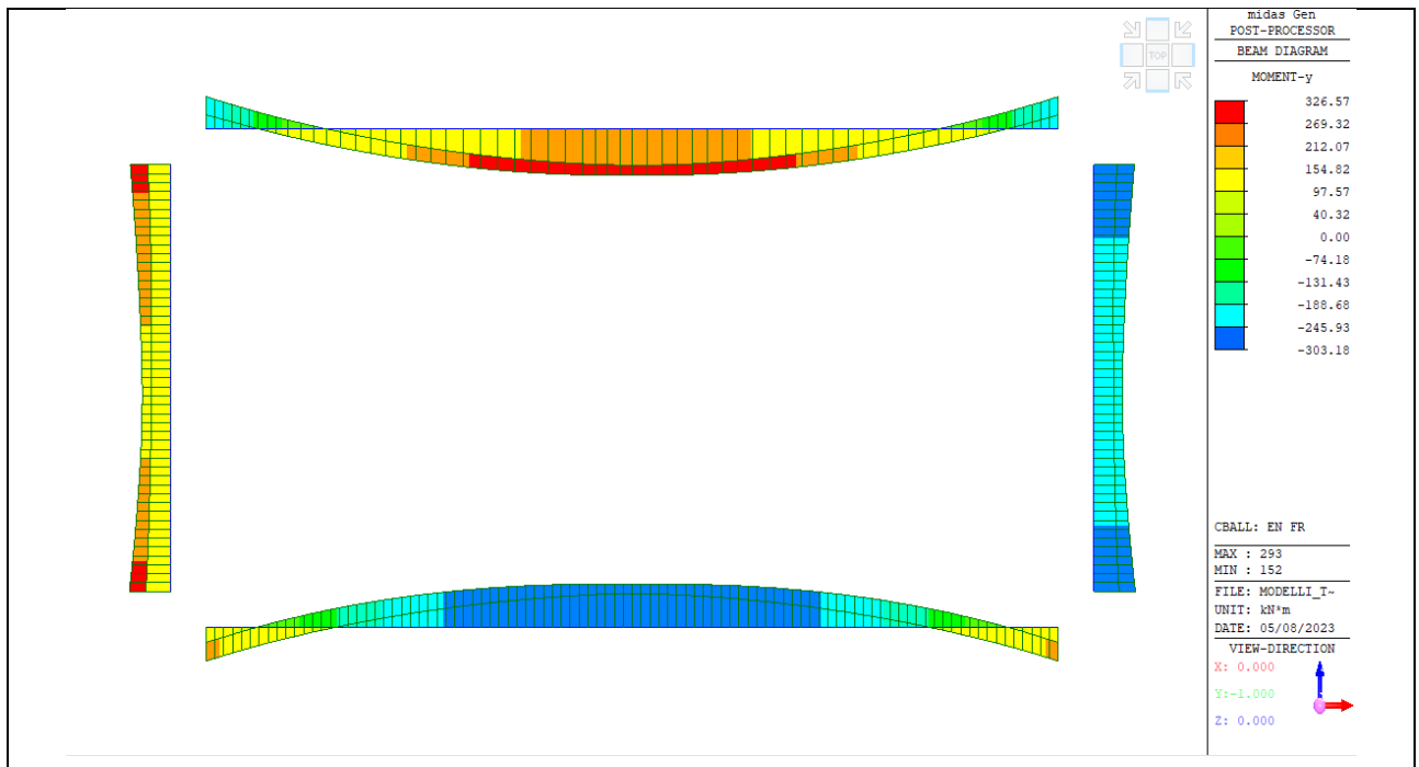
Figura 17: Momento flettente (kNm) – Involuppo FREQUENTE
