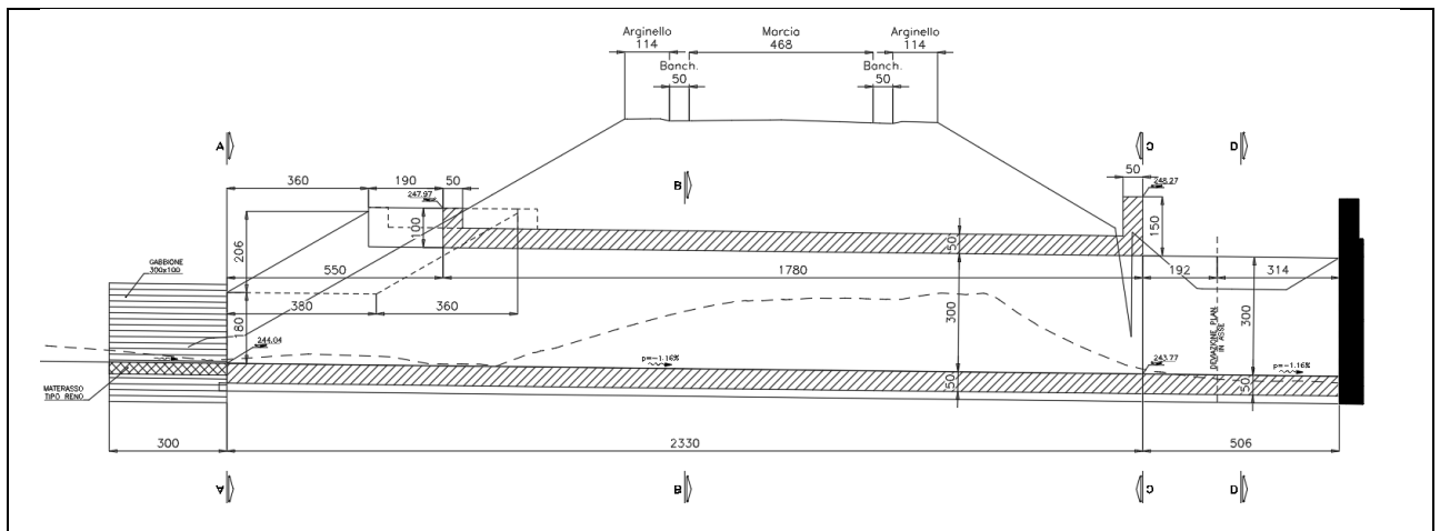
Figura 2: Sezione longitudinale
