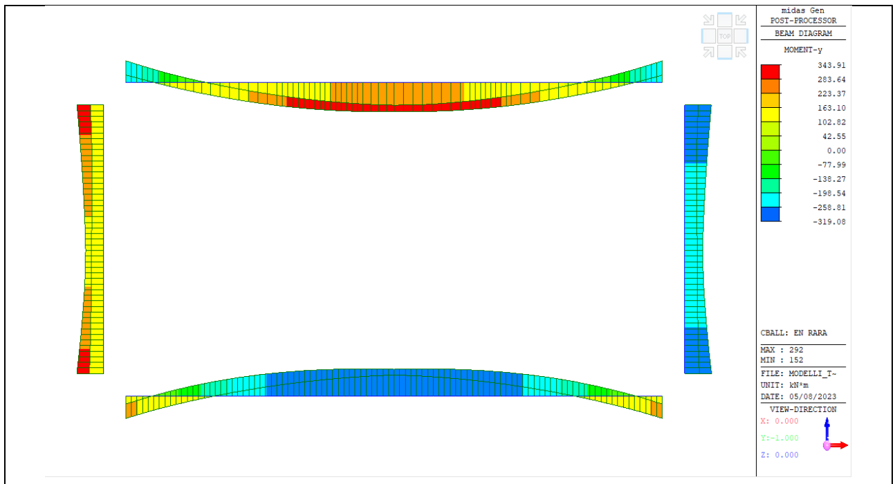
Figura 15: Momento flettente (kNm) – Involuppo RARA
