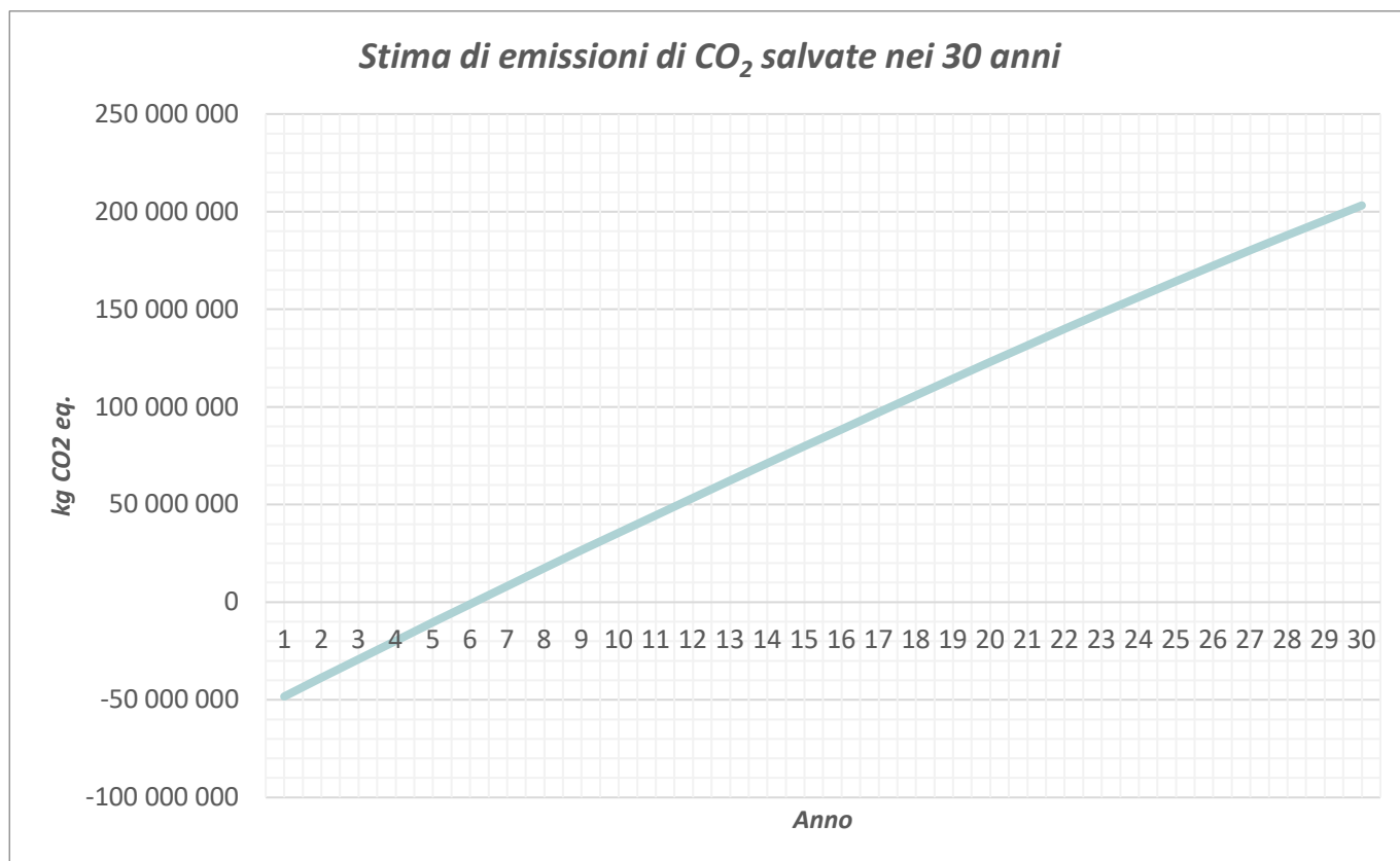
Figura 11 – Stima di risparmi di CO 2 nei 30 anni di vita dell'impianto fotovoltaico.
