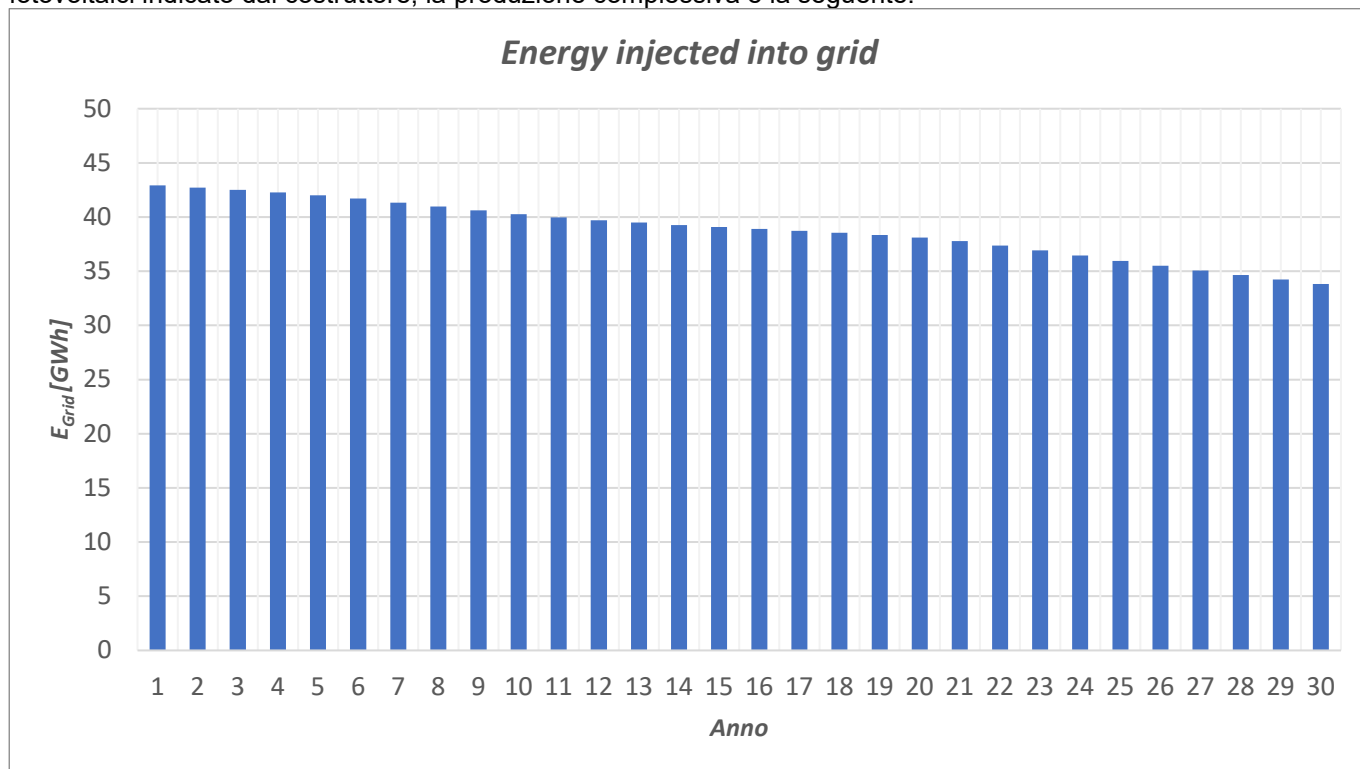
Figura 6 - Energia immessa in rete nei 30 anni di vita dell’impianto
