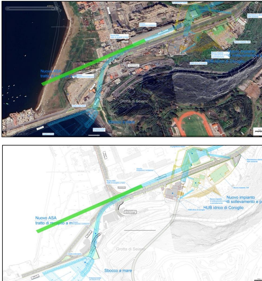
Fig.1 Foce del Collettore ASA seguendo percorso rettilineo
