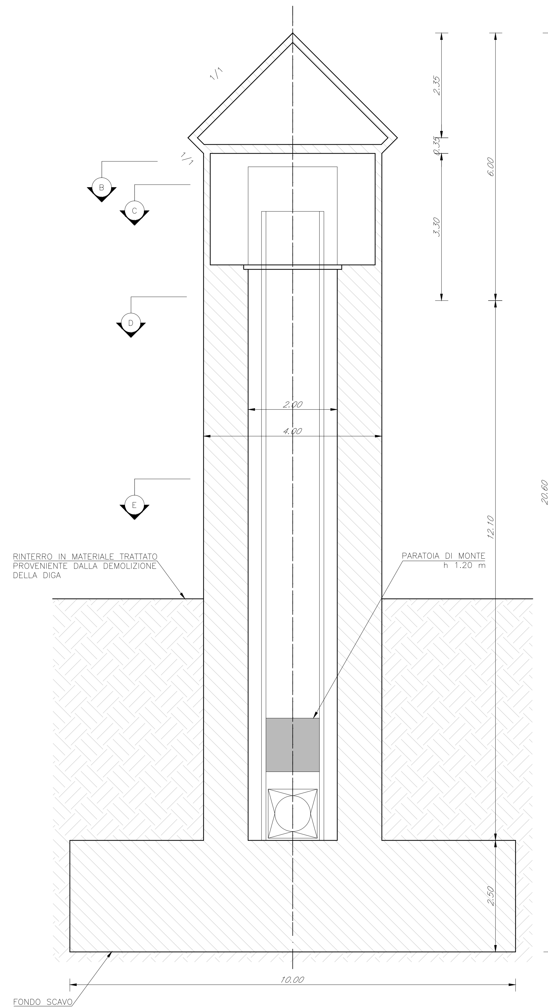
SEZIONE A
