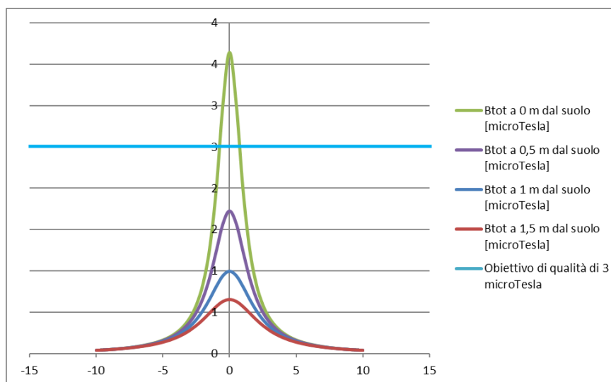
Andamento del campo magnetico generato dal cavidotto, composto da una terna da 630 mm 2
