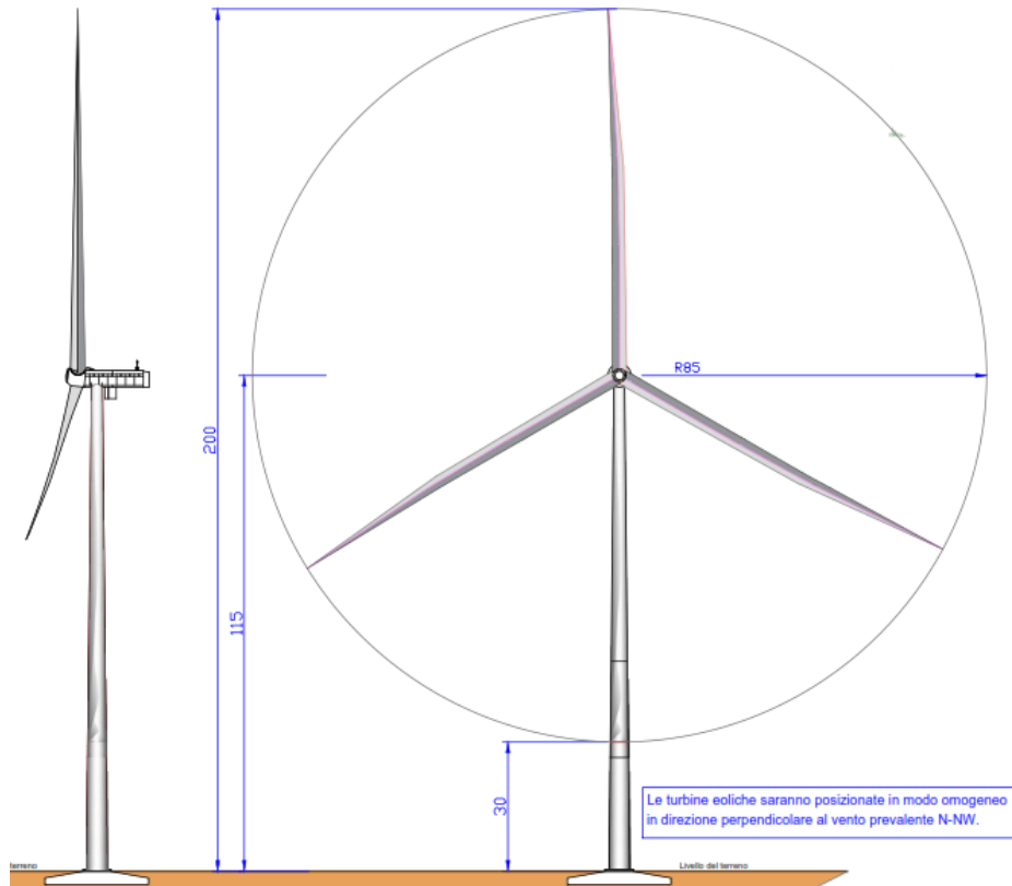
Figura 6 - Struttura aerogeneratore.
