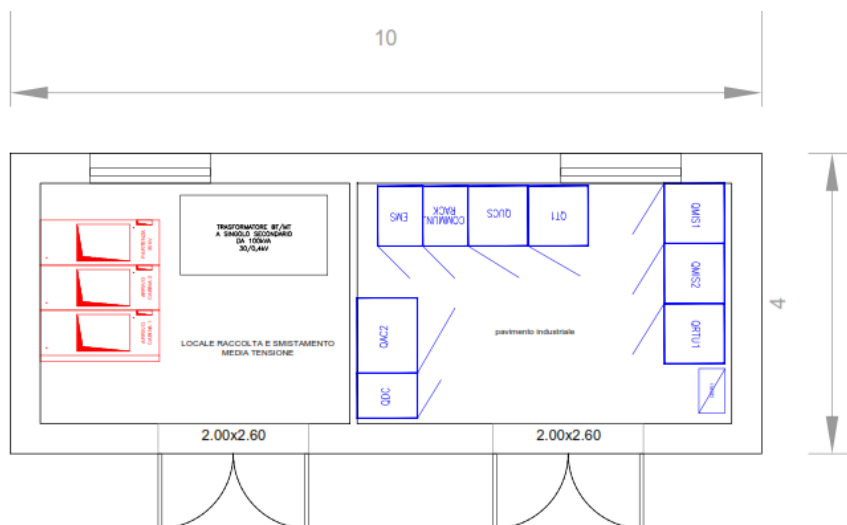
Figura 9 - Pianta della Cabina di Raccolta e smistamento
