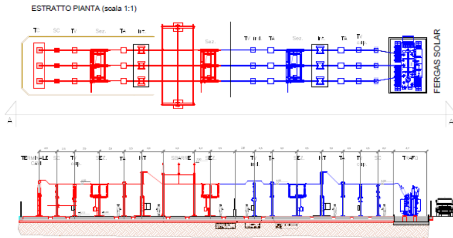
Figura 10 – Pianta della SSE utente
