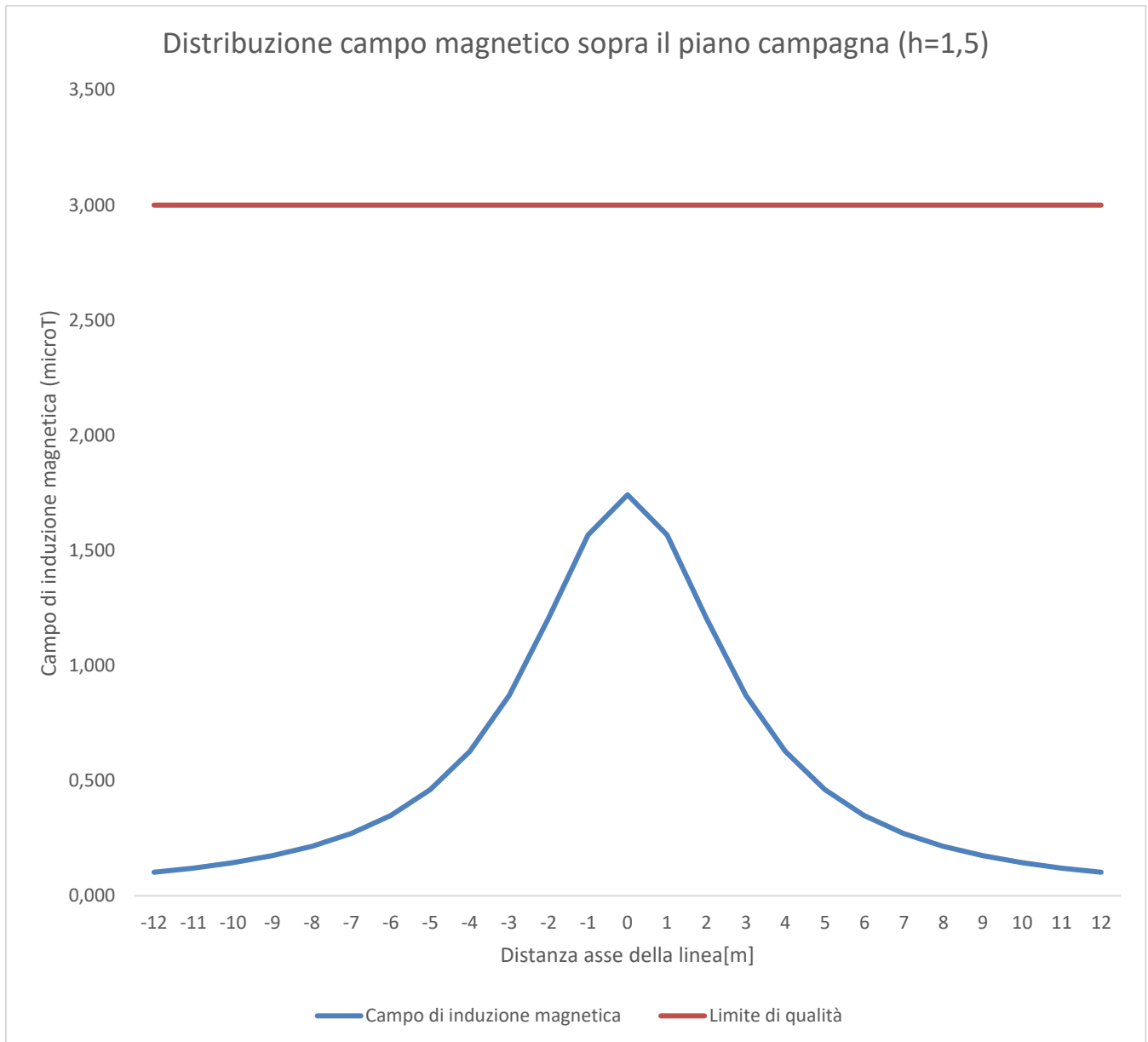
Figura 13 – Andamento dell'induzione magnetica per il caso AT
