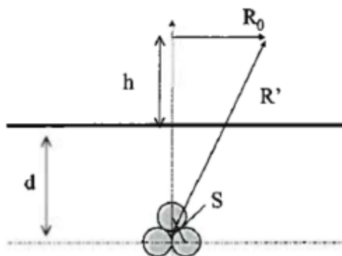
Figura 11 – Schema di principio per il calcolo delle distanze da terne di cavi interrati con poa a trifoglio oltre le quali l'induzione magnetica è inferiore all'obiettivo di qualità
