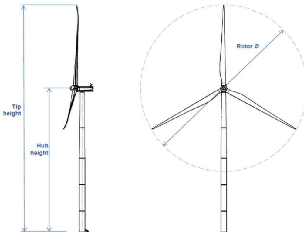
Figura 6 – Esempio Aerogeneratore
