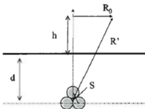
Figura 13 – Schema di principio per il calcolo delle distanze da terne di cavi interrati con poa a trifoglio oltre le quali l'induzione magnetica è inferiore all'obiettivo di qualità
