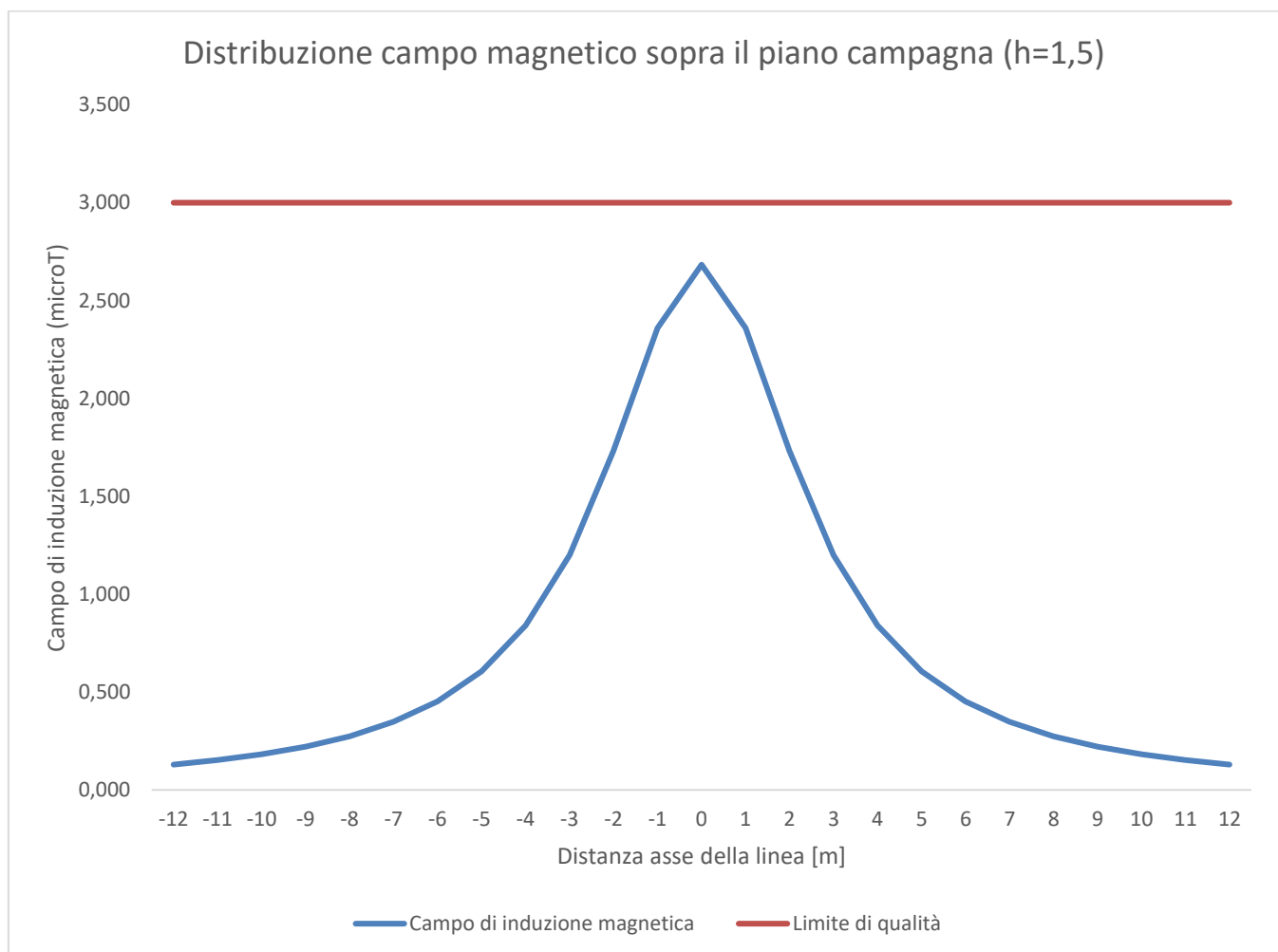
Figura 12 – Andamento dell'induzione magnetica per il caso MT
