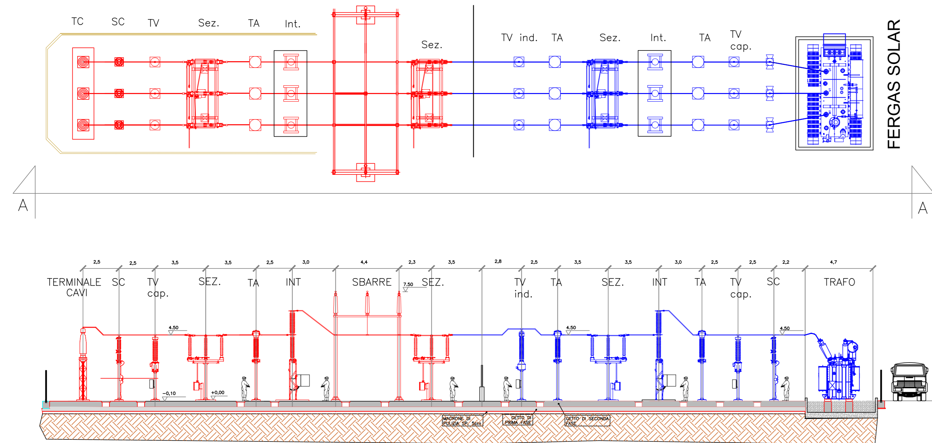
ESTRATTO PIANTA (scala 1:1)
