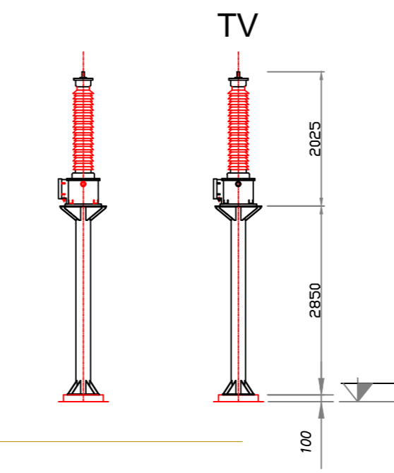
SOSTEGNO CON TV
