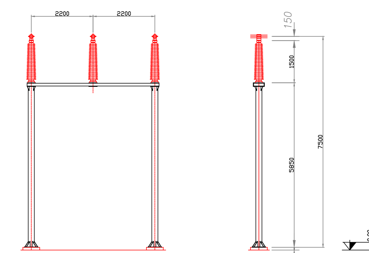
SOSTEGNO PORTALE SBARRE
