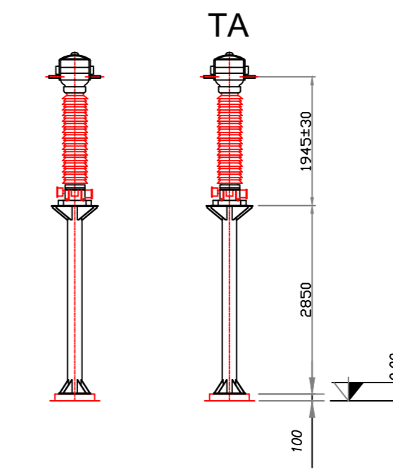
SOSTEGNO CON TA
