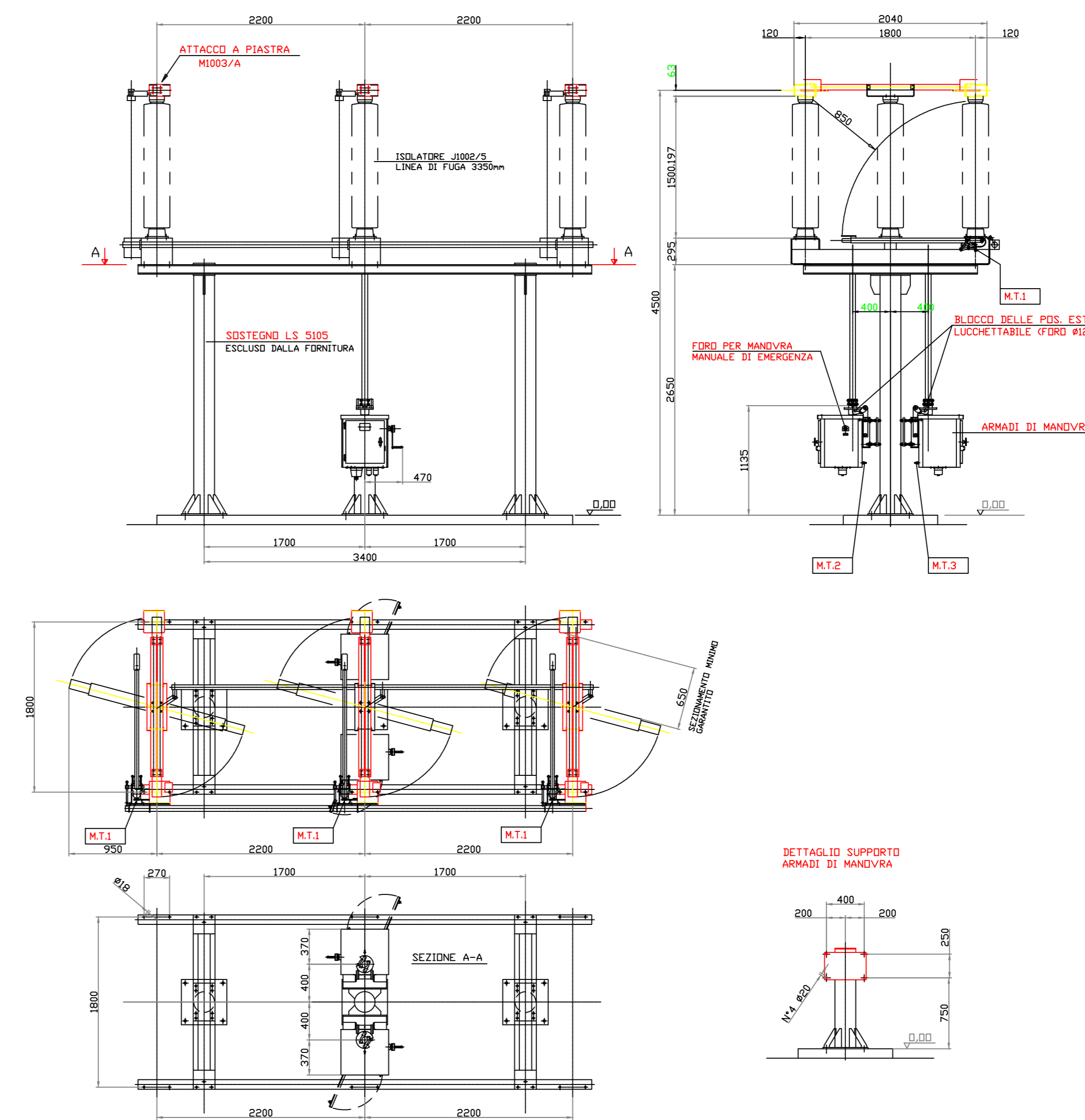
PIANTA (scala 1:200)
