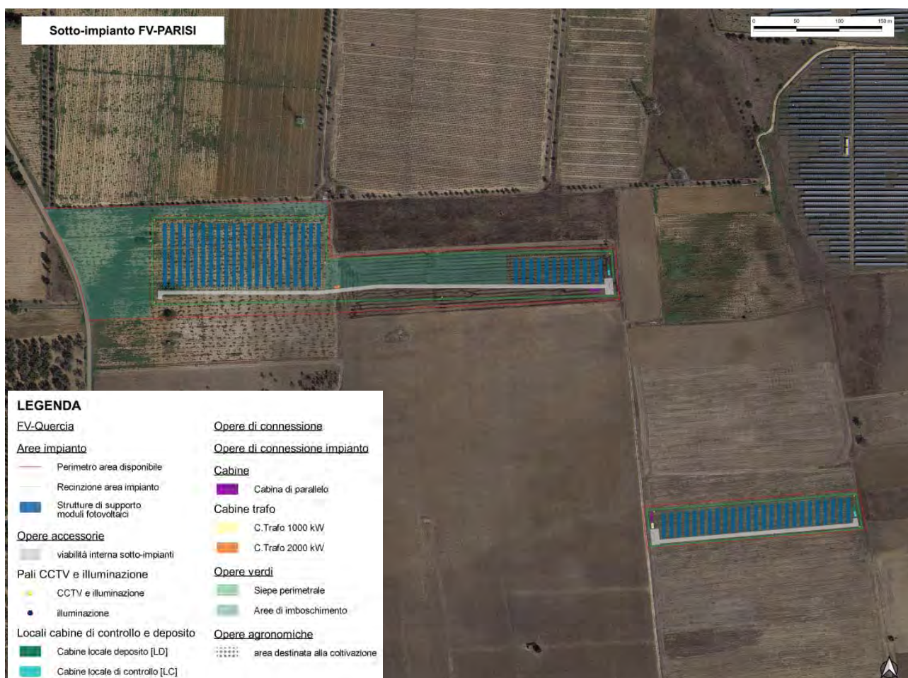
Figura 9-11 - Layout agrovoltaico sotto-impianto FV-Parisi
