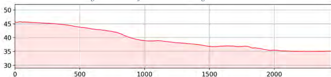
Figura 6-86 Profilo altimetrico lungo la LoS17
