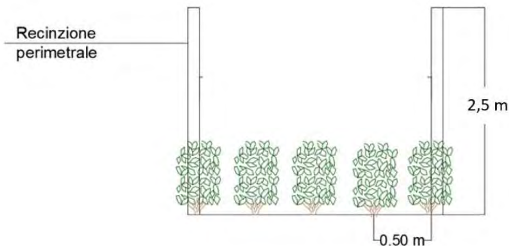
Figura 10-1 - Dettaglio siepe perimetrale
