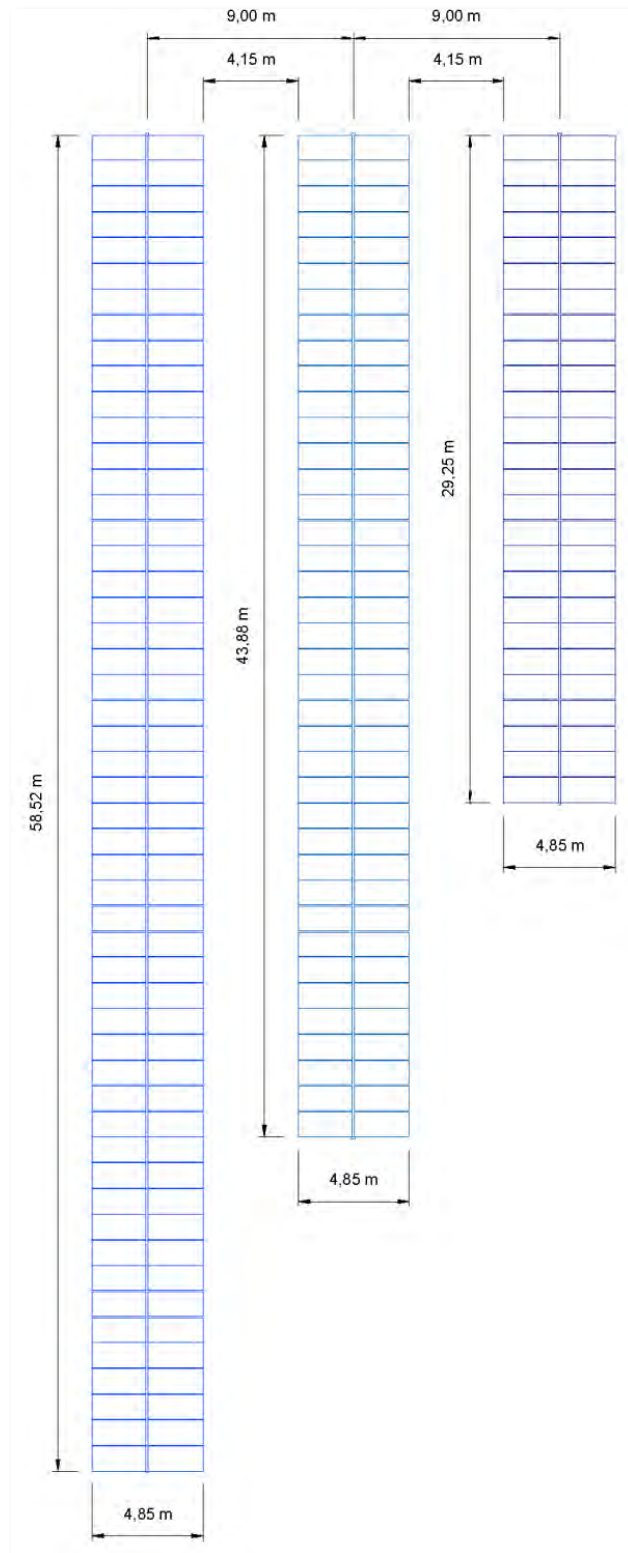
Figura 4-37 - Tipologie di strutture per l'alloggiamento dei moduli fotovoltaici
