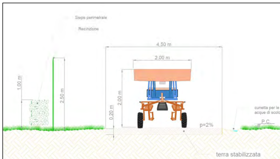
Figura 6-2 - Dettaglio costruttivo delle strade per la viabilità interna al sito di installazione dell'impianto agro-fotovoltaico
