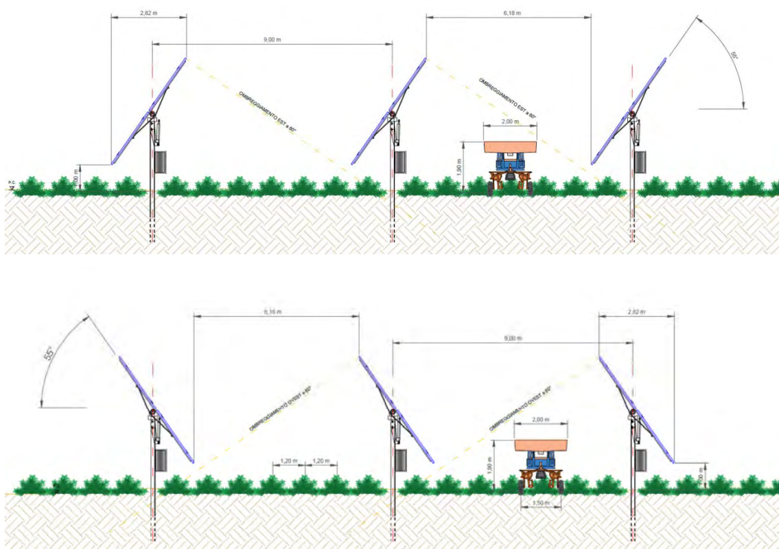
Figura 9-8 - Dettaglio sezione trasversale delle strutture di sostegno dei moduli fotovoltaici con rotazione +/-55°
