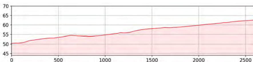
Figura 6-66 Profilo altimetrico lungo la LoS5
