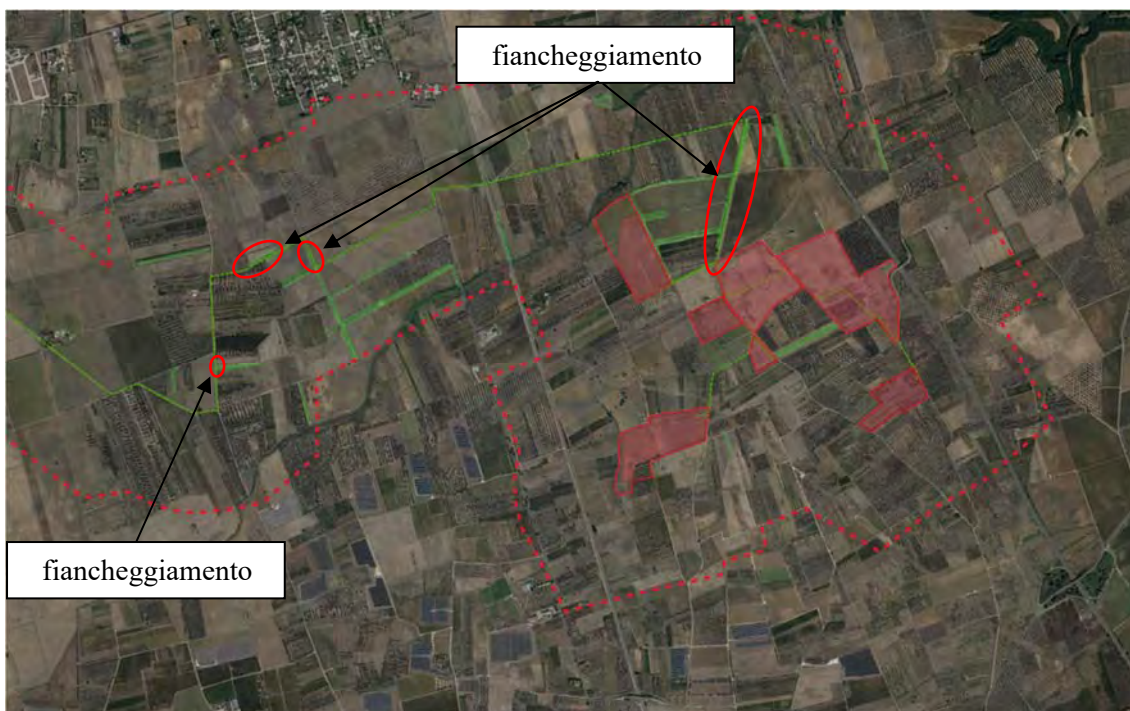
Figura 6-41 - Ortofoto del parco agro-fotovoltaico FV-Quercia con rilievo elementi del paesaggio agrario - Dettaglio opere di connessione - Cavidotto MT di parallelo interrato (in rosso le interferenze riscontrate)
