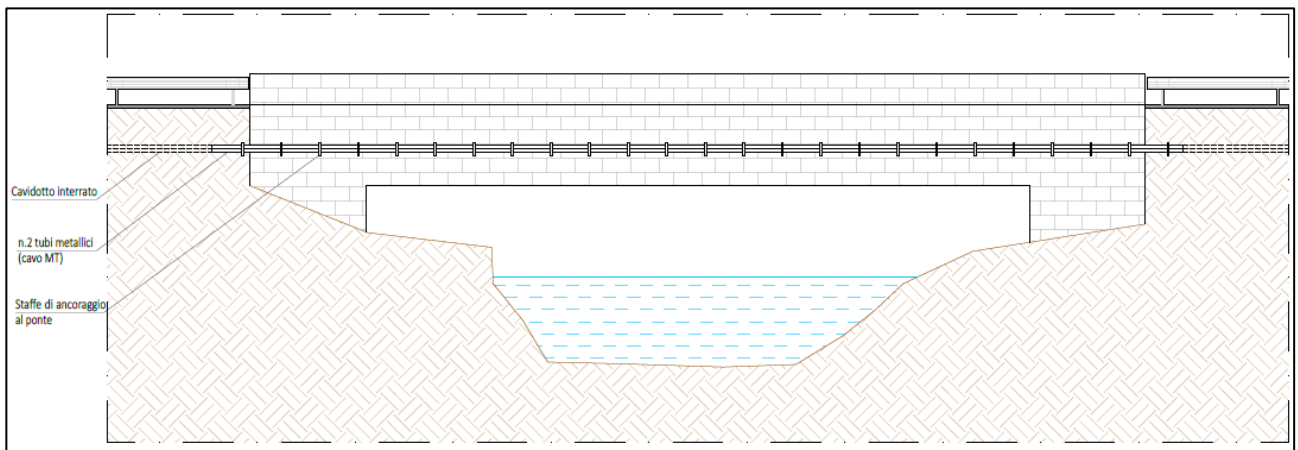
Figura 7-22 - Esempio di dettaglio tecnico risoluzione interferenza mediante staffe laterali.
