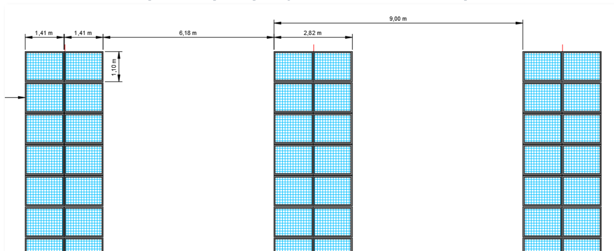
Figura 4-40 - Particolare costruttivo indicante l'interasse tra le strutture e la distanza tra le file di moduli - Inclinazione pannelli 0° (per le opere agricole si rimanda alla relazione specialistica)
