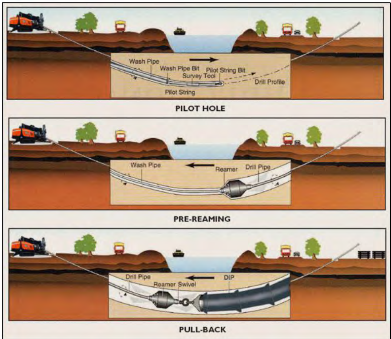
Figura 7-20 - Schema esemplificativo di risoluzione interferenza mediante T.O.C. (Trivellazione Orizzontale Controllata)
