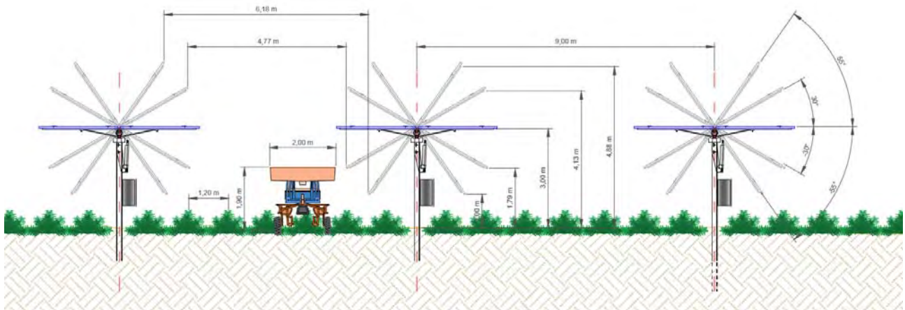
Figura 9-9 - Dettaglio sezione trasversale delle strutture di sostegno dei moduli fotovoltaici
