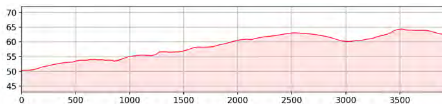
Figura 6-65 Profilo altimetrico lungo la LoS4
