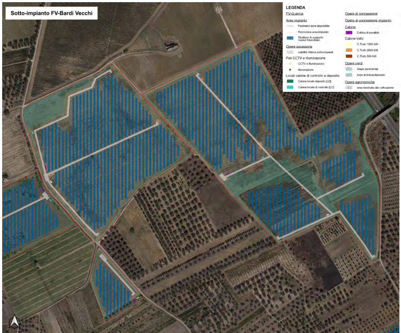
Figura 9-13 - Layout agro-fotovoltaico sotto-impianto FV-Bardi Vecchi
