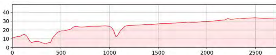
Figura 6-77 Profilo altimetrico lungo la LoS11
