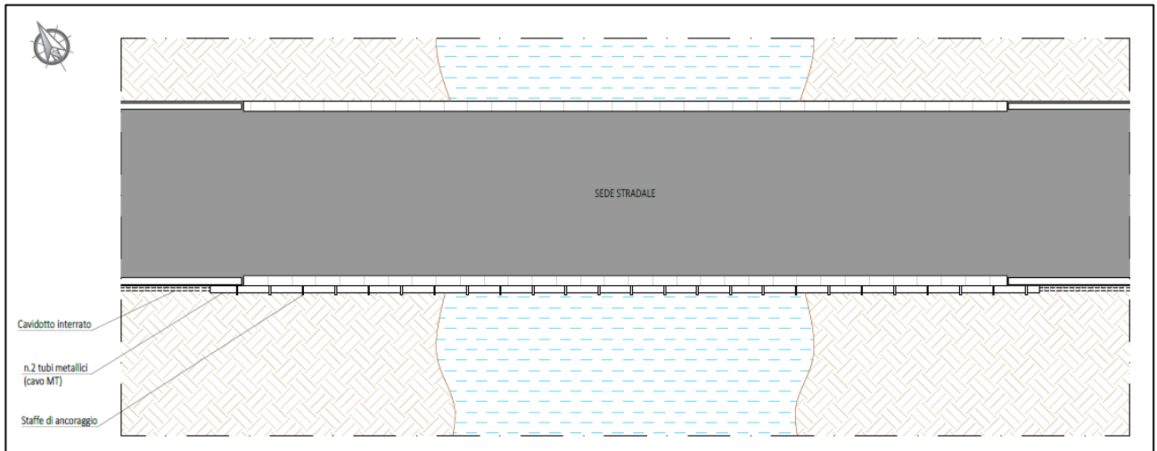
Figura 7-21 - Esempio di dettaglio tecnico risoluzione interferenza mediante staffe laterali.
