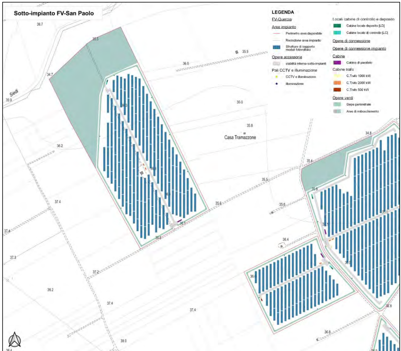
Figura 4-20 - Inquadramento su CTR del sotto-impianto FV-San Paolo
