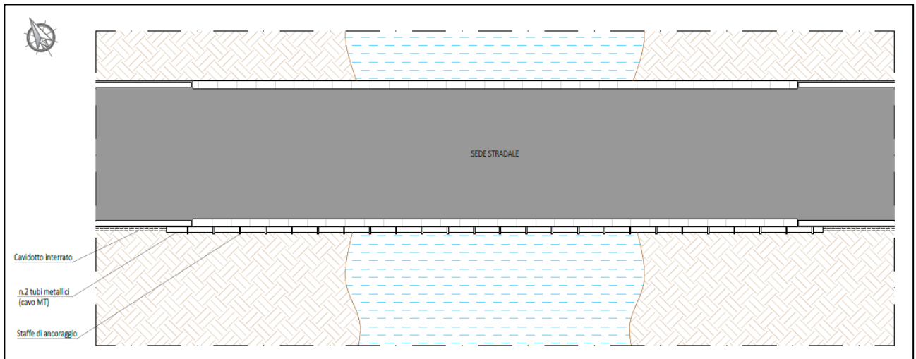
Figura 6-17 - Esempio di dettaglio tecnico risoluzione interferenza mediante staffe laterali. Dettaglio pianta
