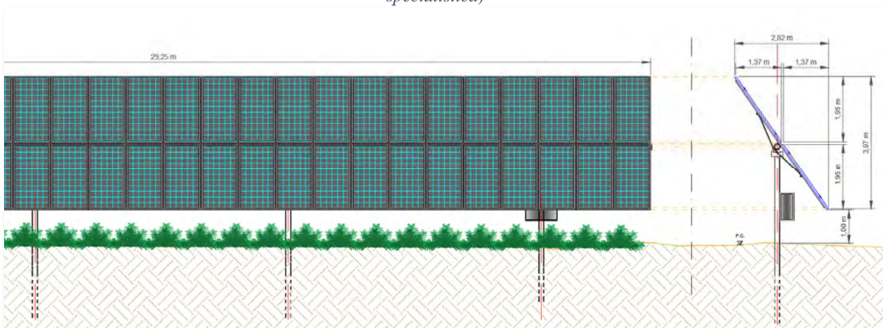
Figura 4-39 - Vista frontale e vista in sezione con rotazione di 55^\circ , (per le opere agricole si rimanda alla relazione specialistica)
