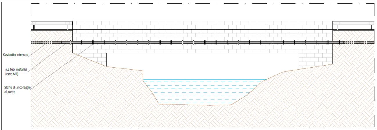
Figura 6-18 - Esempio di dettaglio tecnico risoluzione interferenza mediante staffe laterali. Dettaglio prospetto
