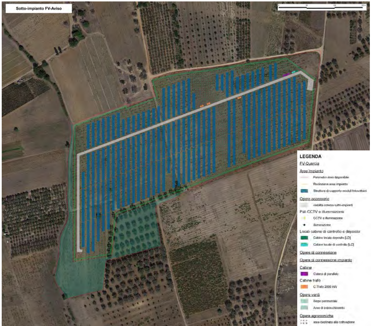
Figura 9-15 - Layout agro-fotovoltaico sotto-impianto FV-Aviso
