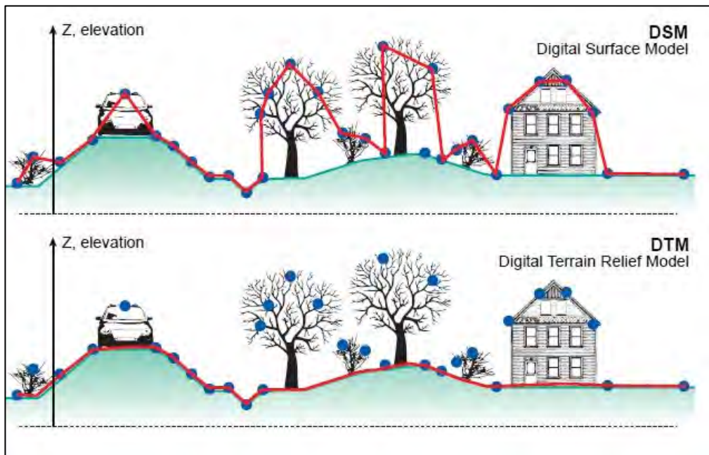
Figura 6-57 - Differenza tra un DEM di tipo DTM e uno di tipo DSM
