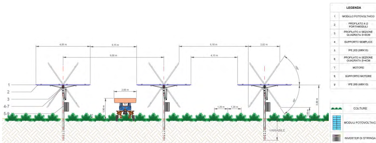
Figura 9-7 - Dettaglio sezione trasversale delle strutture di sostegno dei moduli fotovoltaici con relativa legenda esplicativa
