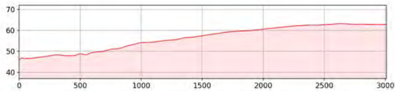
Figura 6-62 Profilo altimetrico lungo la LoS2
