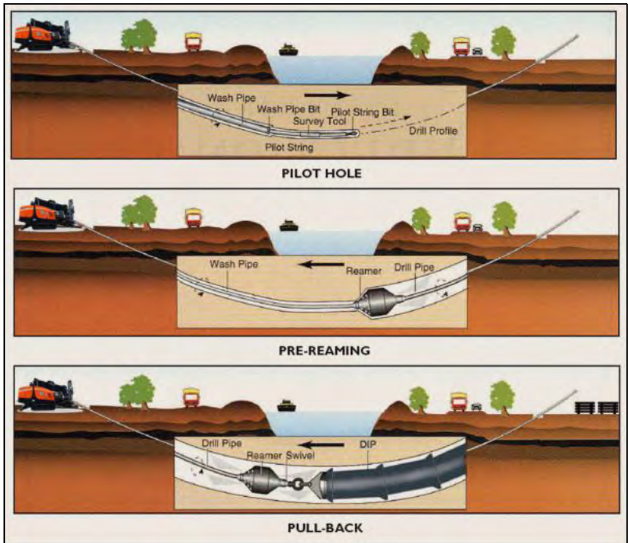
Figura 6-16 - Schema esemplificativo di risoluzione interferenza mediante T.O.C. (Trivellazione Orizzontale Controllata)
