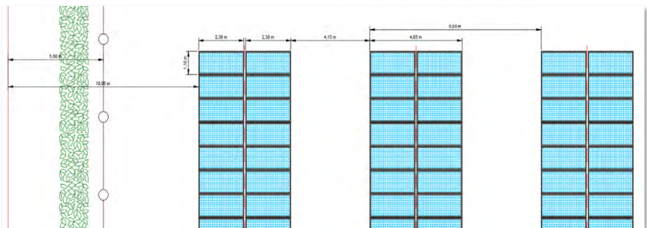
Figura 4-42 - Particolare costruttivo in pianta della recinzione e della barriera alberata, (per le opere agricole si rimanda alla relazione specialistica)
