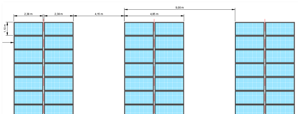
Figura 4-40 - Particolare costruttivo indicante l'interasse tra le strutture e la distanza tra le file di moduli - Inclinazione pannelli 0° (per le opere agricole si rimanda alla relazione specialistica)
