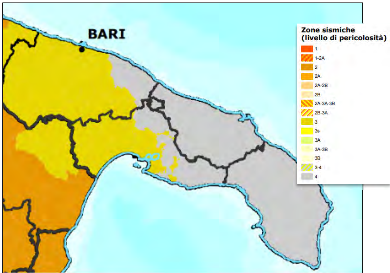
Figura 4-36 - Stralcio della carta della classificazione sismica del territorio italiano aggiornata al 2015 (fonte: " https://protezionecivile.puglia.it/ ")
