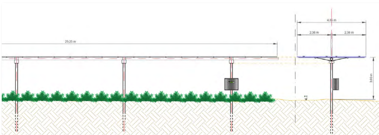
Figura 4-38 - Vista frontale e vista in sezione con rotazione di 0^\circ , (per le opere agricole si rimanda alla relazione specialistica)
