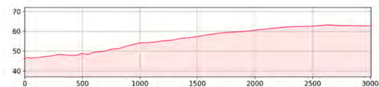
Figura 6-63 Profilo altimetrico lungo la LoS3
