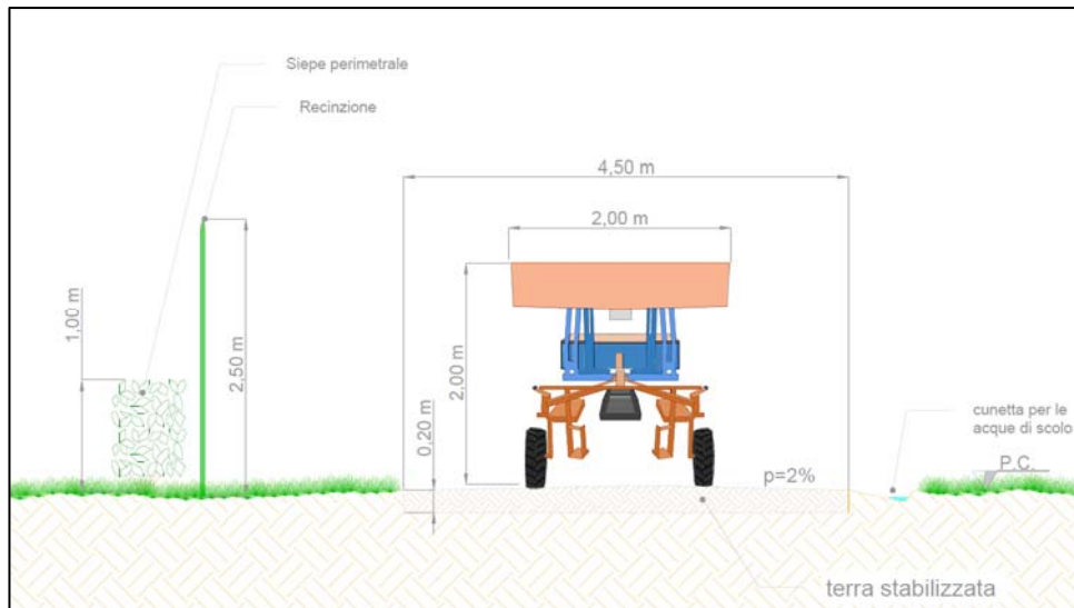
Figura 17-1 - Dettaglio costruttivo delle strade per la viabilità interna al sito di installazione dell'impianto fotovoltaico
