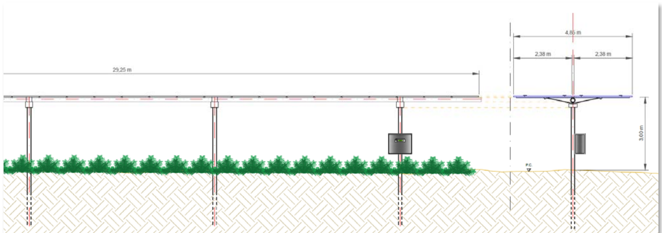
Figura 6-2 - Vista frontale e vista in sezione con rotazione di 0^\circ , (per le opere agricole si rimanda alla relazione specialistica)
