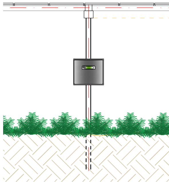
Figura 7-3 - Dettaglio alloggiamento dell'inverter sulle strutture dei moduli
