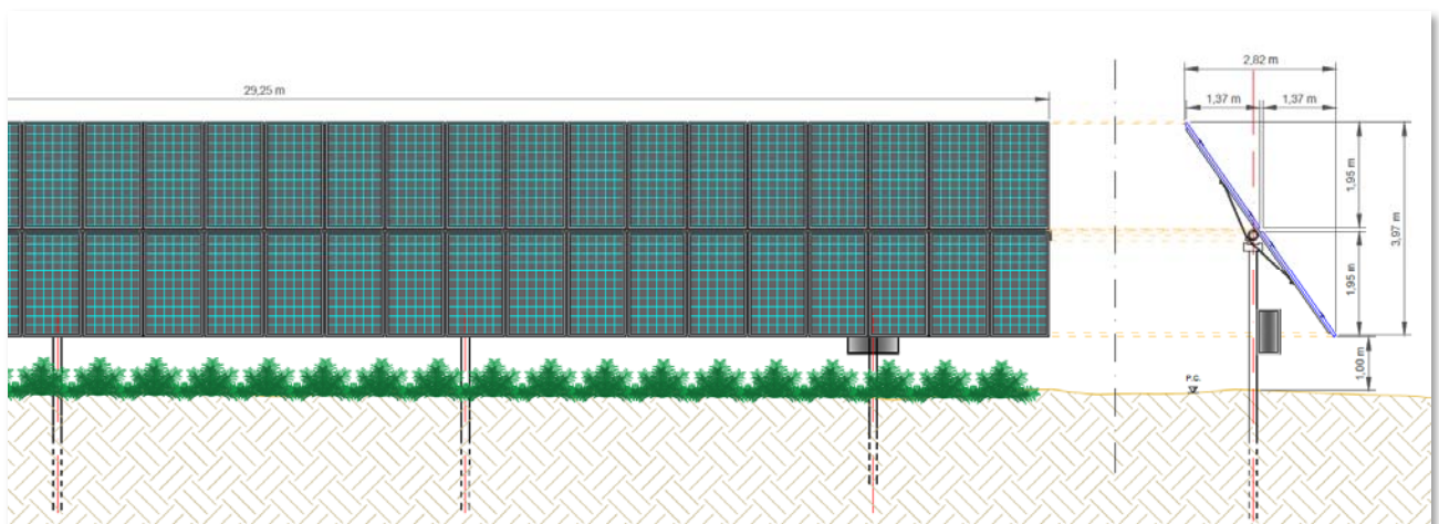
Figura 6-3 - Vista frontale e vista in sezione con rotazione di 55^\circ , (per le opere agricole si rimanda alla relazione specialistica)
