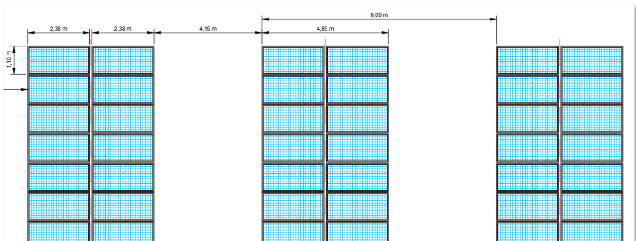
Figura 6-4 - Particolare costruttivo indicante l'interasse tra le strutture e la distanza tra le file di moduli - Inclinazione pannelli 0^\circ (per le opere agricole si rimanda alla relazione specialistica)
