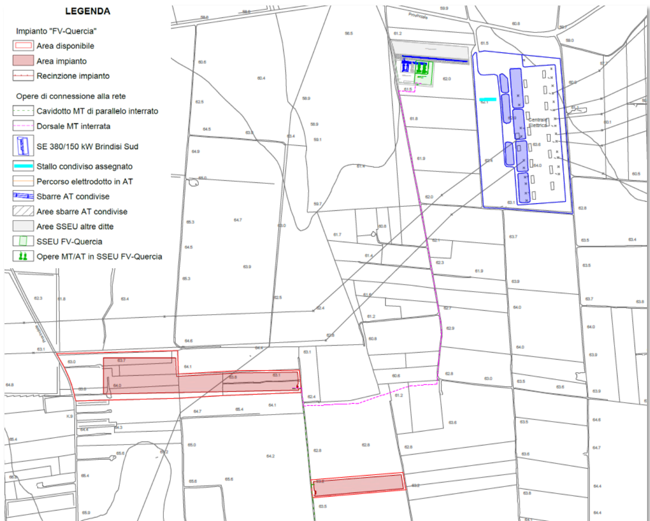
Figura 6-7 - Schema di convogliamento dell'energia dalla cabina di parallelo ubicata nel sotto-impianto FV-Parisi alla Stazione Elettrica di Trasformazione 380/150 kV "Brindisi Sud"
