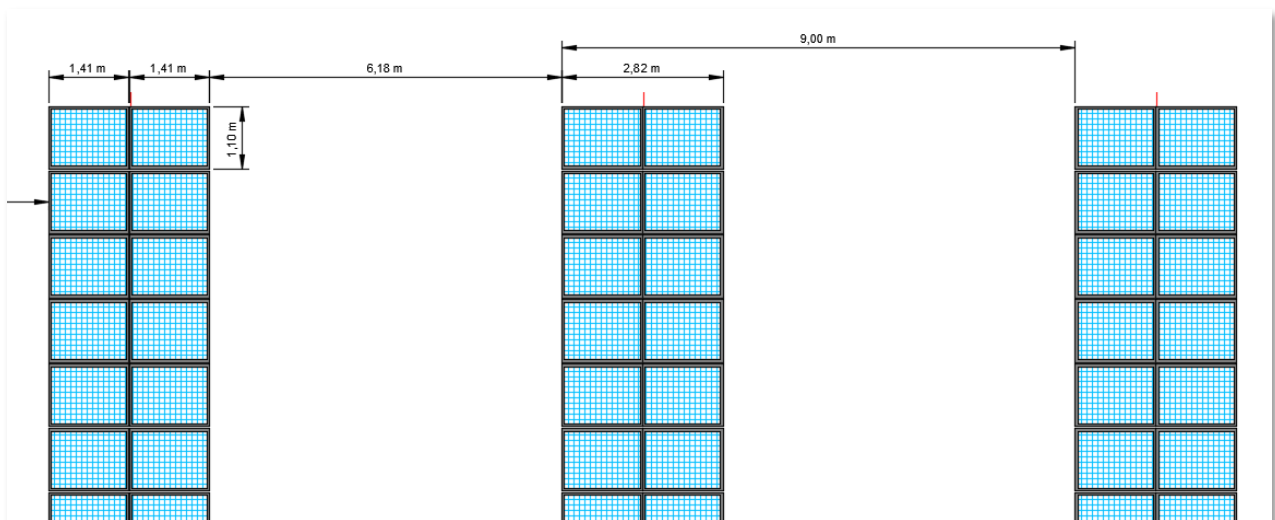
Figura 6-5 - Particolare costruttivo indicante l'interasse tra le strutture e la distanza tra le file di moduli - Inclinazione pannelli 55^\circ (per le opere agricole si rimanda alla relazione specialistica)
