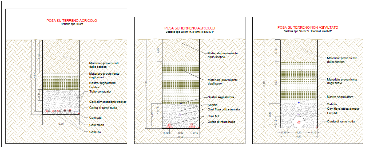
Figura 8-4 - Esempio di posa di cavi BT/MT su terreno agricolo e/o asfaltato
