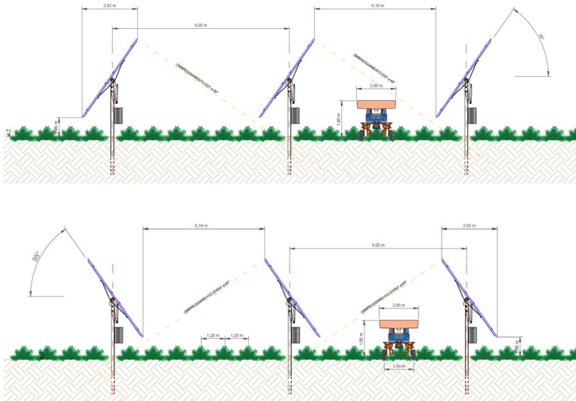
Figura 13-8 - Dettaglio sezione trasversale delle strutture di sostegno dei moduli fotovoltaici con rotazione \pm 55^\circ
