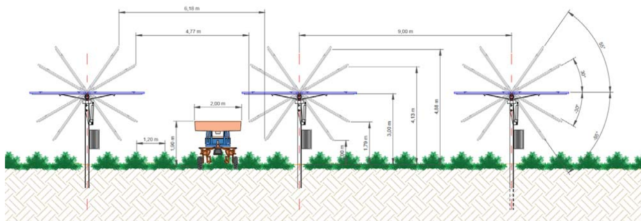
Figura 13-9 - Dettaglio sezione trasversale delle strutture di sostegno dei moduli fotovoltaici
