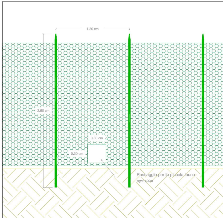
Figura 17-4 - Particolare recinzione passaggio piccola fauna
