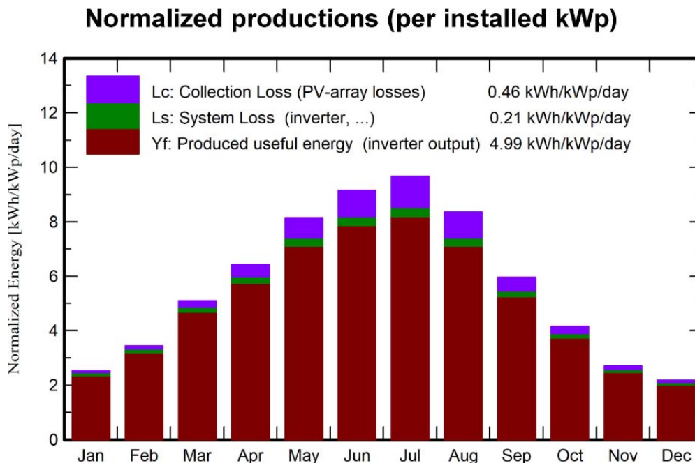
Figura 9-1 Producibilità per kWp installato
