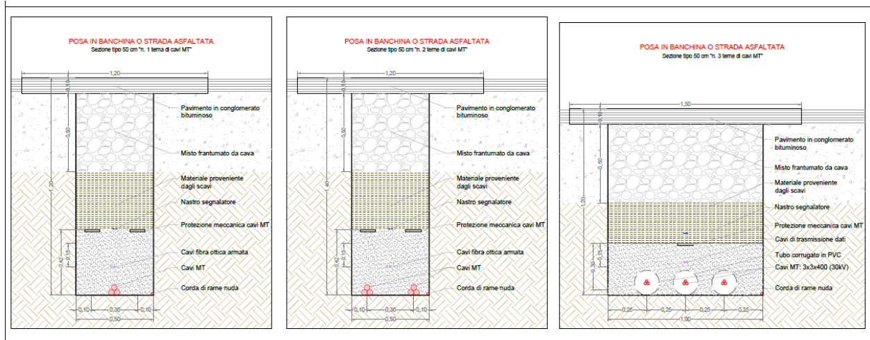
Figura 8-3 - Esempio di posa di cavi MT su banchina o strada asfaltata
