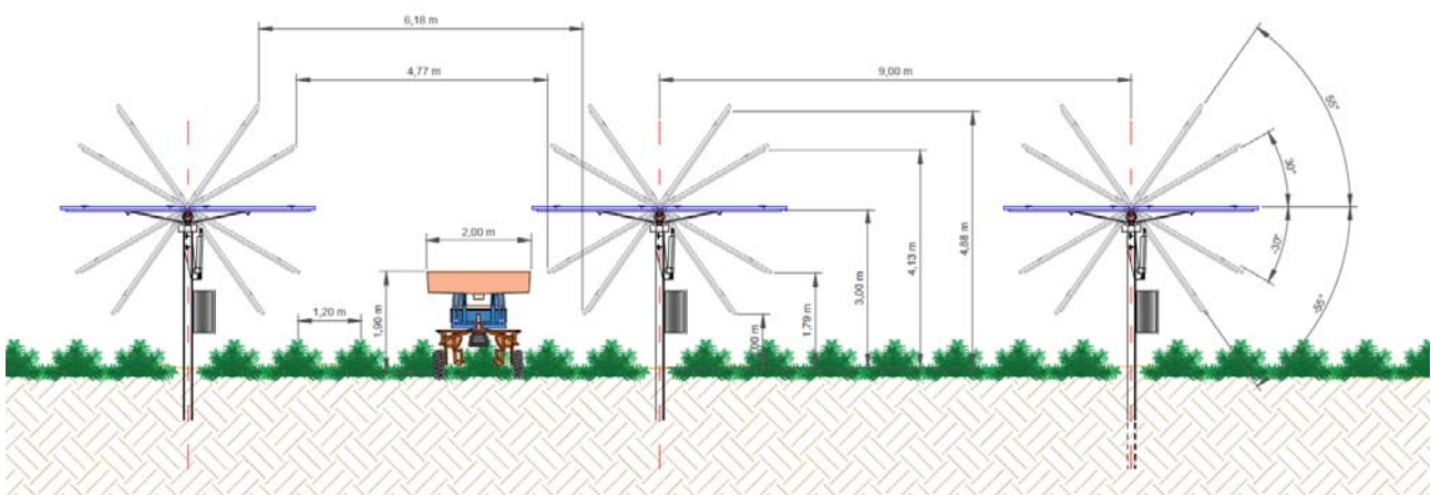
Figura 7-6 - Particolare costruttivo in sezione delle strutture di sostegno dei moduli fotovoltaici
