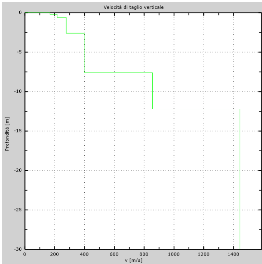
Fig. 12a: Profilo Vs numerico calcolato MASW 1
