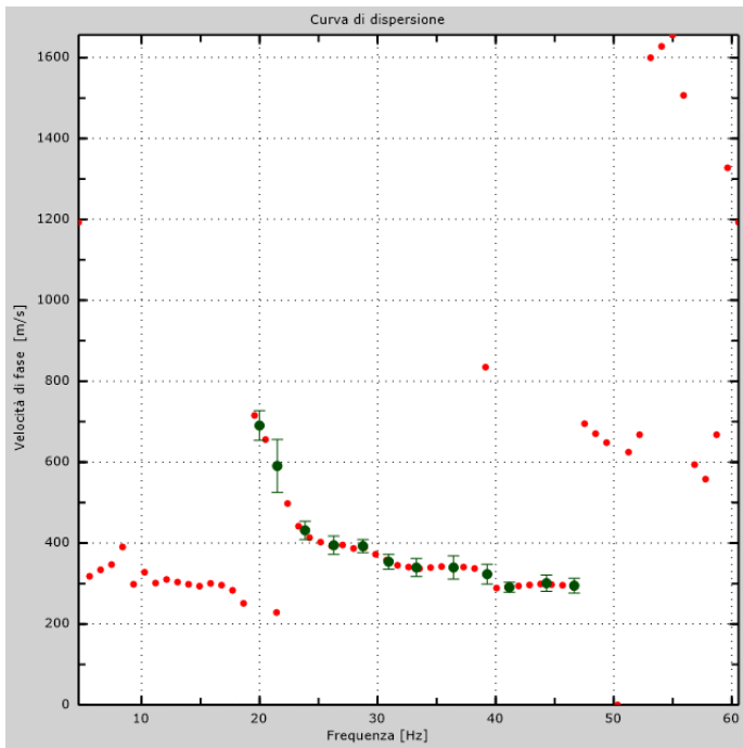
Fig. 10a: Curva di dispersione sperimentale MASW 1
