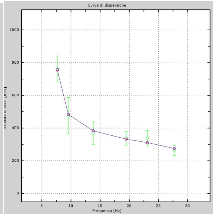
Fig. 11b: Punti sperimentali (verde), modi di Rayleigh (ciano), curva apparente (blu), curva numerica (rosso) MASW 2
