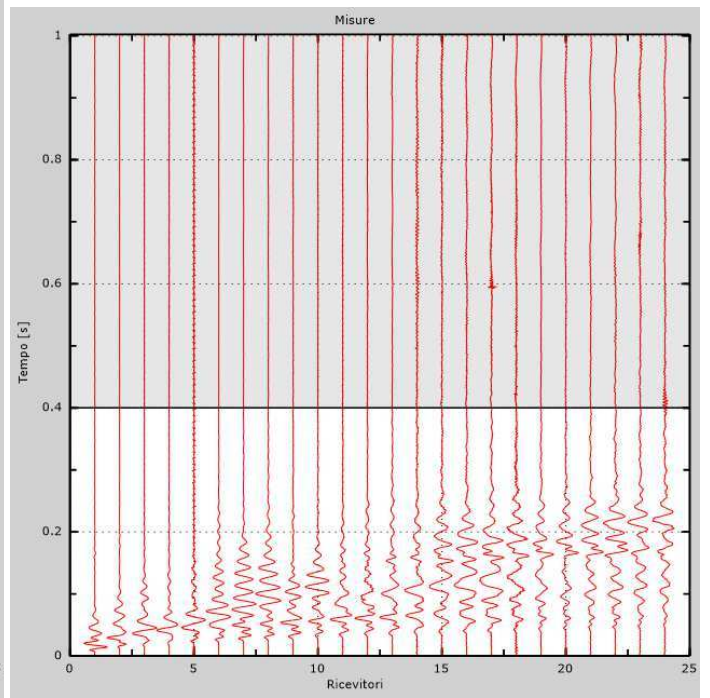
Fig. 8b: Sismogramma sperimentale MASW 2
