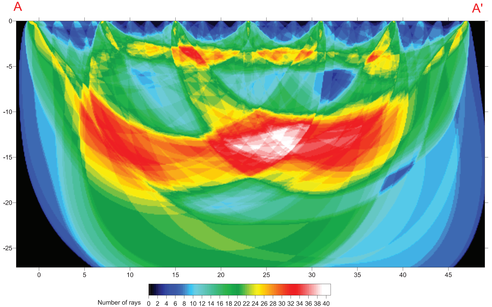
Fig.14 : Impianti Ovest (Parisi), 100 WET iterations, RMS error 1.8 %, Rays paths
