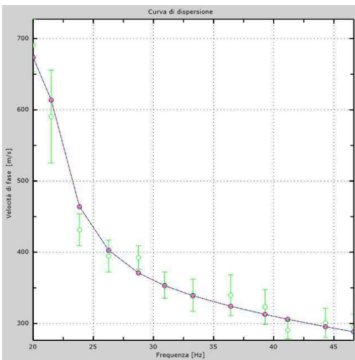
Fig. 11a: Punti sperimentali (verde), modi di Rayleigh (ciano), curva apparente (blu), curva numerica (rosso) MASW 1
