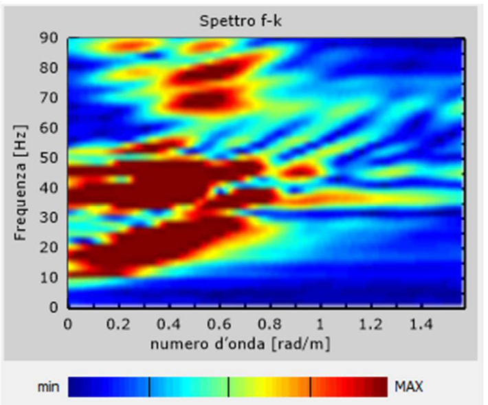
Fig. 9 b: Spettro F-K MASW 1
