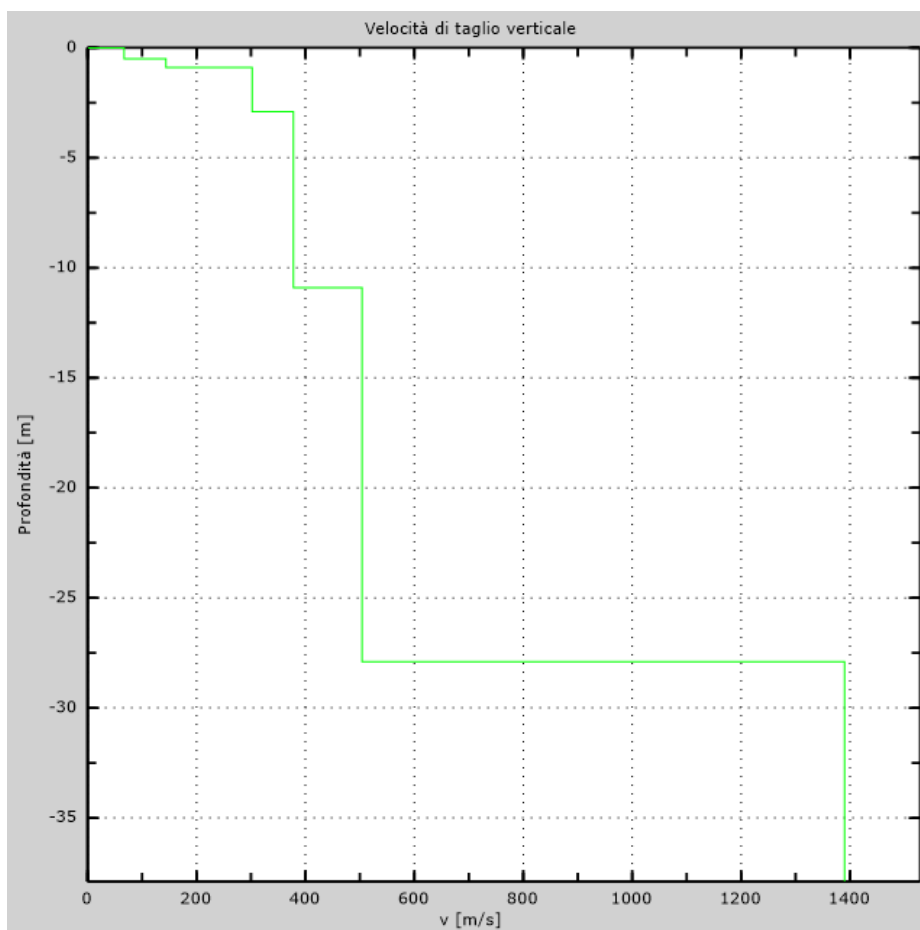
Fig. 12b: Profilo Vs numerico calcolato MASW 2
