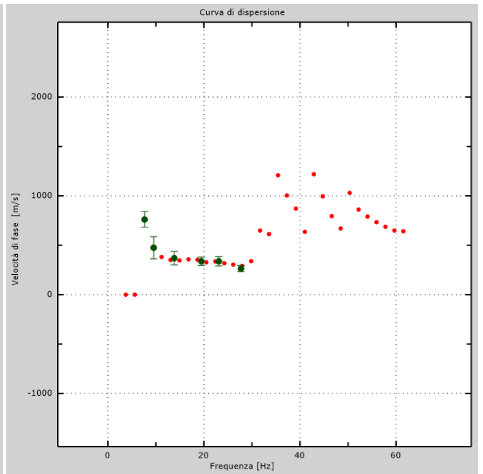
Fig. 10b: Curva di dispersione sperimentale MASW 2
