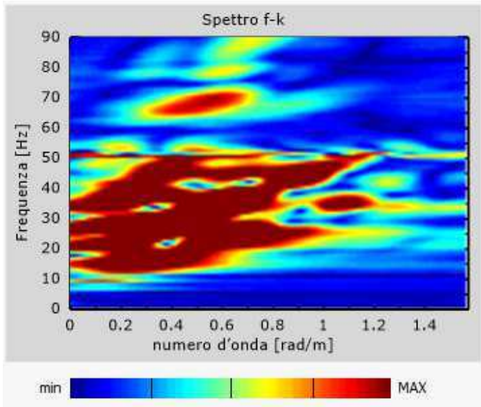
Fig. 9 a: Spettro F-K MASW 1
