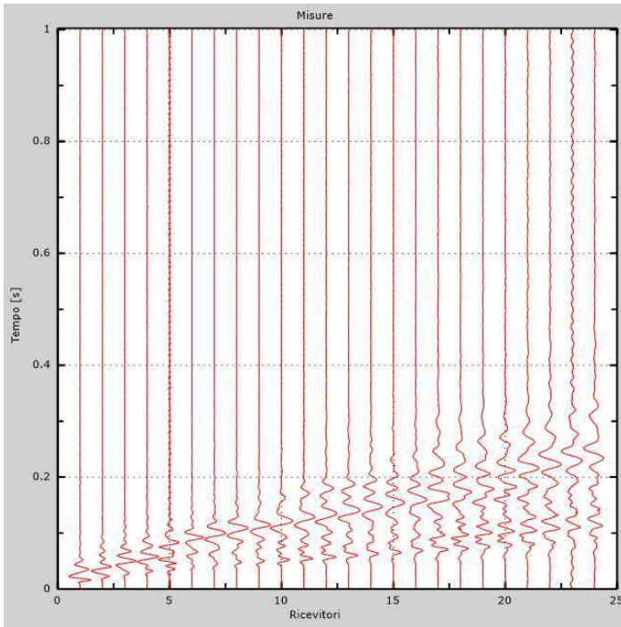
Fig. 8a: Sismogramma sperimentale MASW 1
