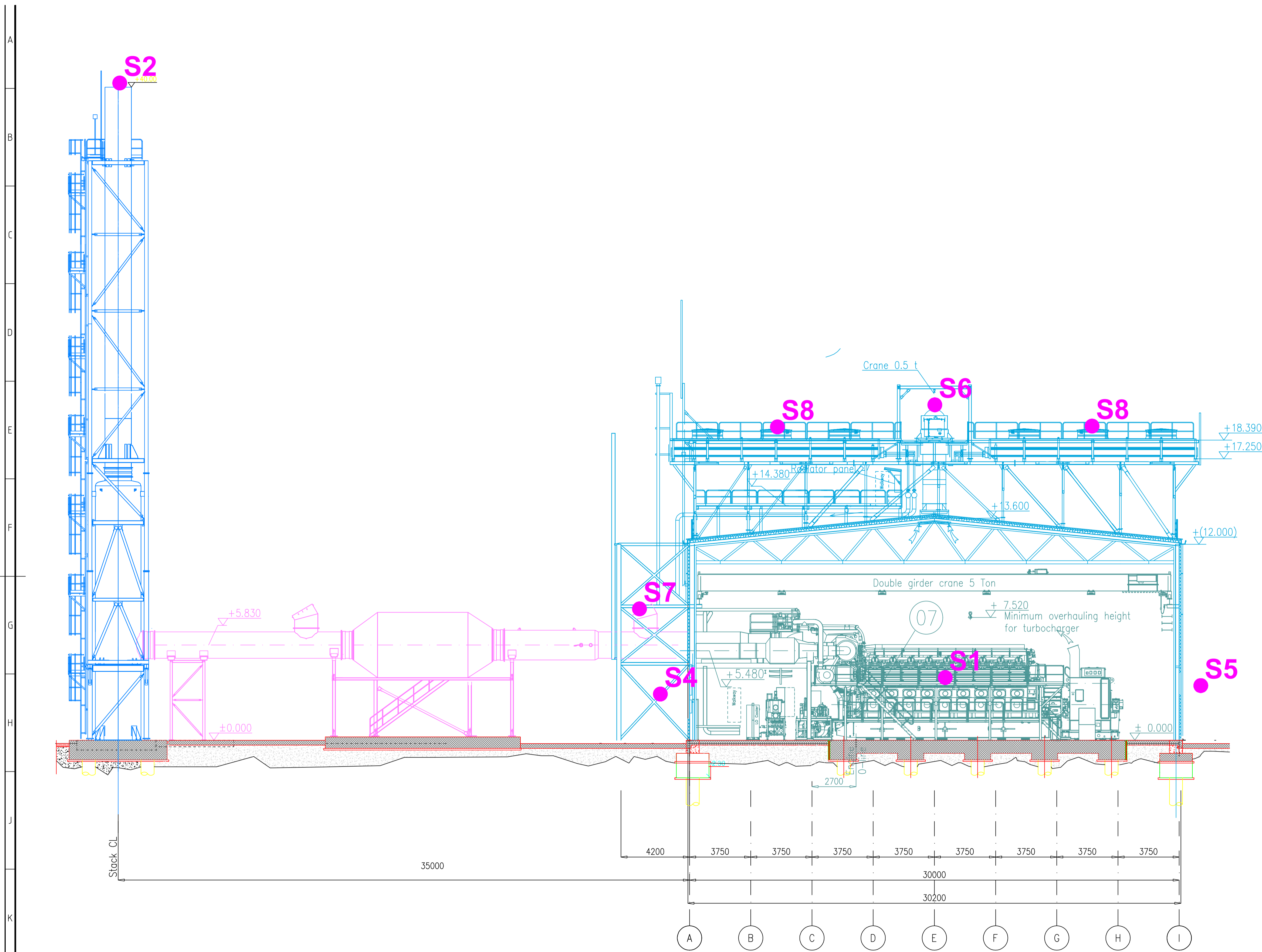
Section A-A
