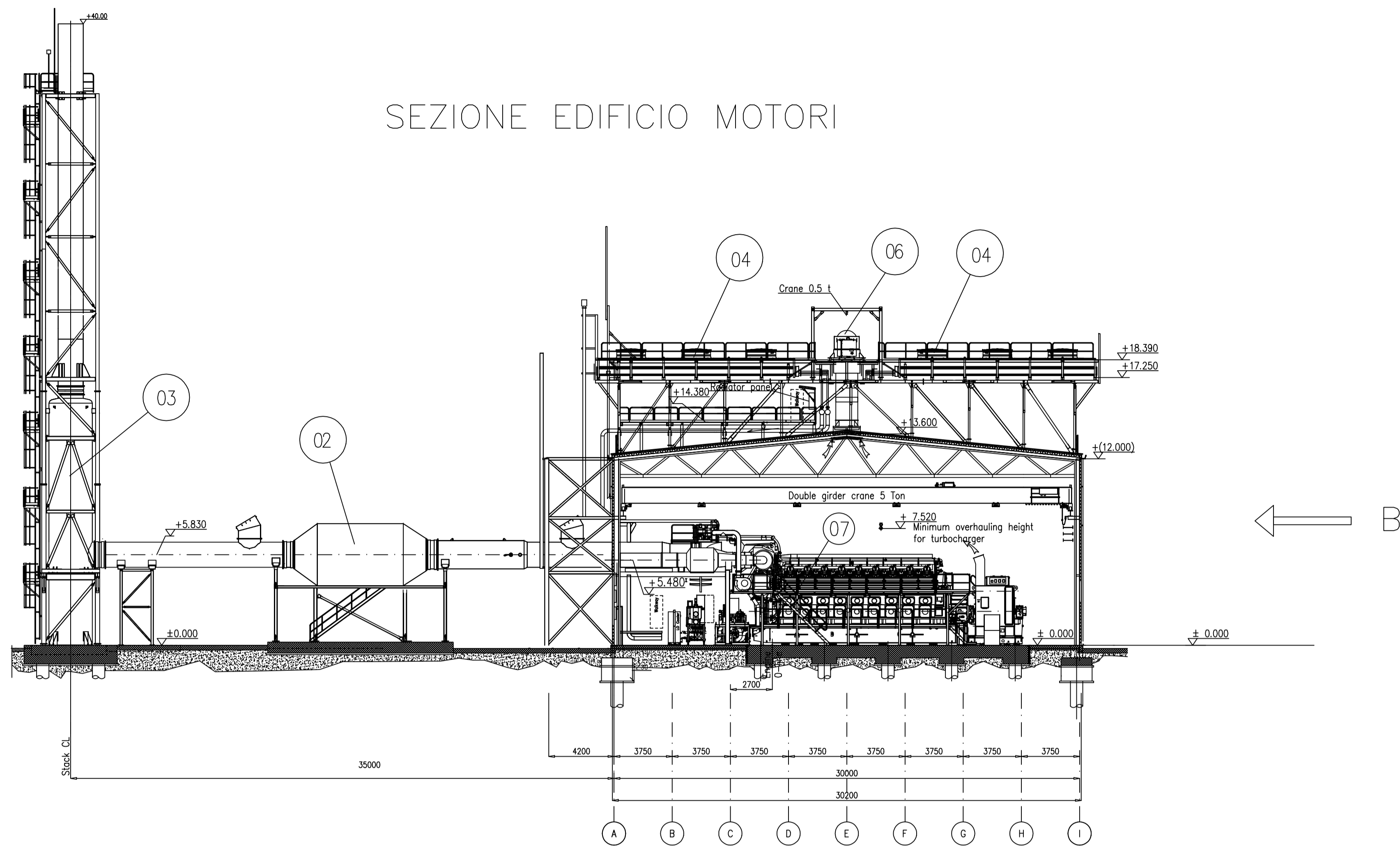
Section A-A
