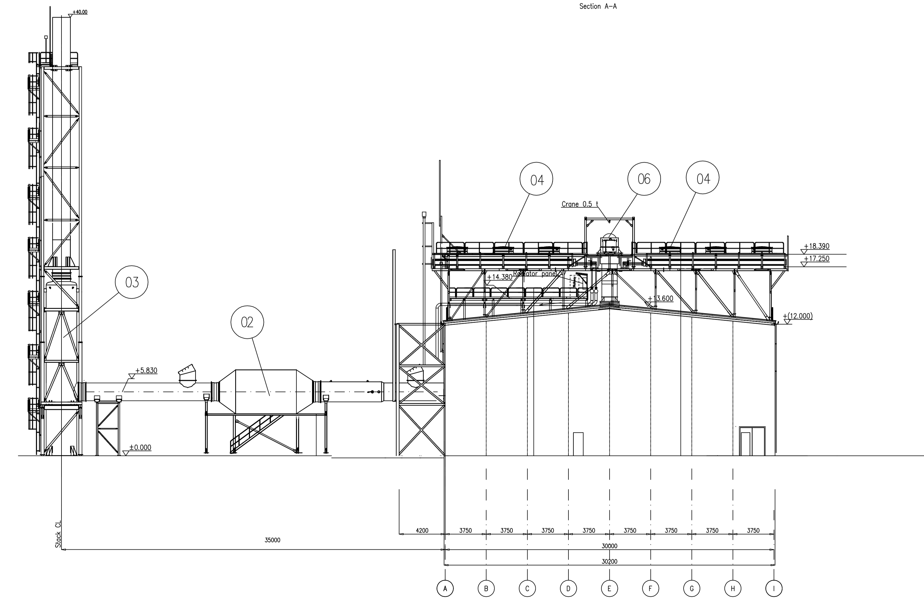
Section A-A
