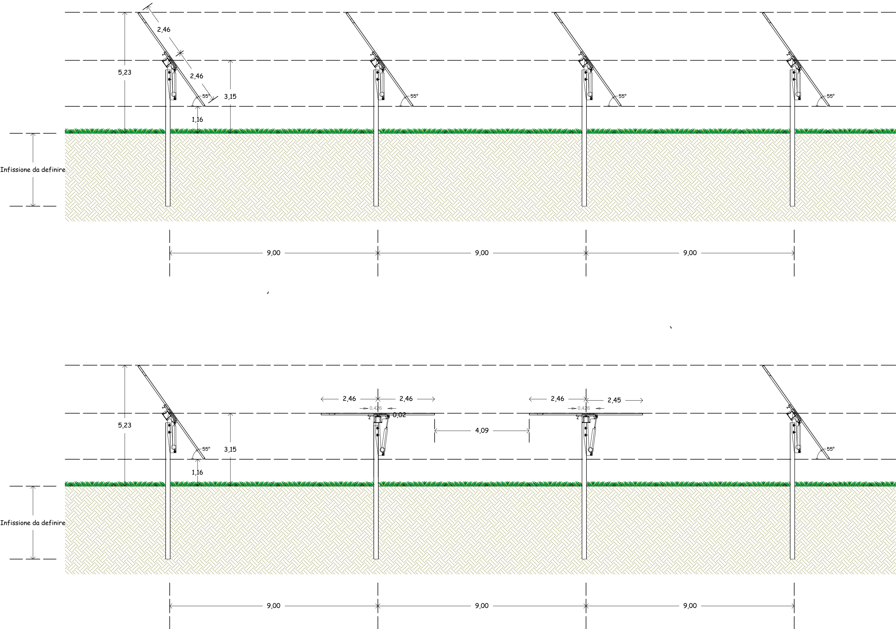
Sezioni trasversali tracker scala 1 : 100
