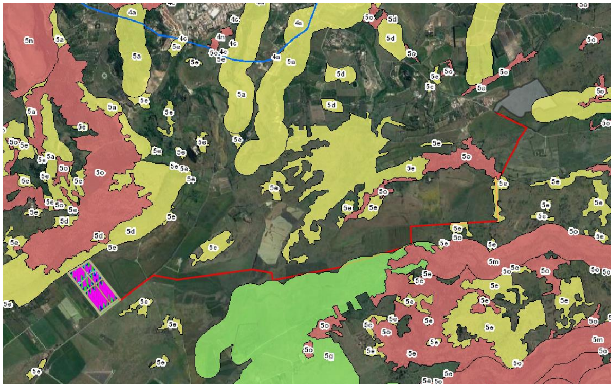
Figura 4 – Inquadramento impianto fotovoltaico e percorso cavidotto rispetto alle zone sottoposte a vincolo paesaggistico
