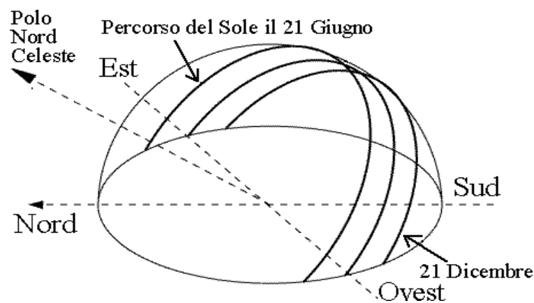
Figura 11 – Movimento apparente del disco solare per un osservatore situato ad una latitudine nord attorno ai 45°. Per tutte le località situate tra il Tropico del Cancro e il Polo Nord Geografico il disco solare non raggiunge mai lo zenit
