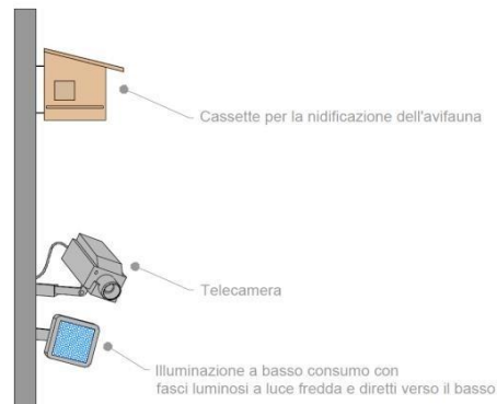
Figura 10 – Esempi di cassette realizzate sui pali dell'impianto per la nidificazione dell'avifauna
