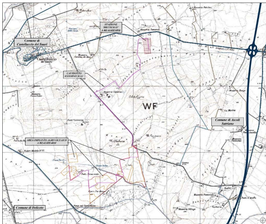
Figura 4 - Tracciato cavidotto AT a 36 kV su base IGM
