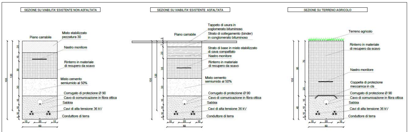
Figura 3 - Particolari sezioni cavidotto esterno AT da 36 kV su strada asfaltata, non asfaltata e terreno agricolo
