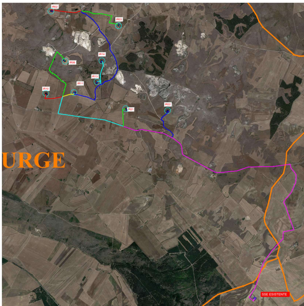
Figura 1 – Inquadramento di ampio raggio su ortofoto dell’area di intervento, situata nel comune di Minervino Murge. Nella figura in alto è rappresentato lo stato di fatto esistente con 16 aerogeneratori e in quella in basso è rappresentato lo stato di progetto con la collocazione dei 9 aerogeneratori
