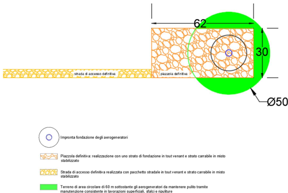
Fig. 3 – schema costruttivo della piazzola permanente dell'aerogeneratore
