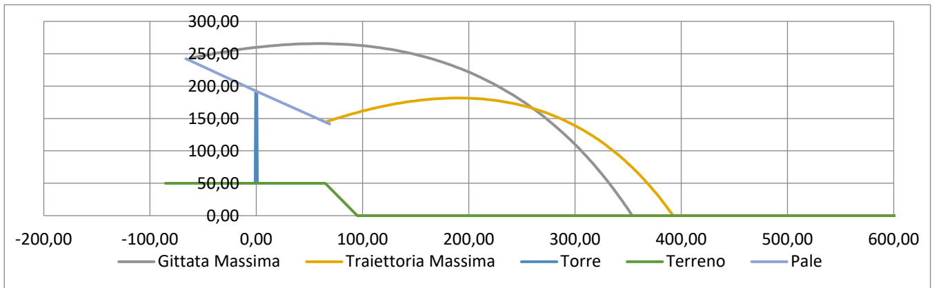
Figura 4 - Traiettoria del moto di un frammento di 10 m, a seguito di rottura
