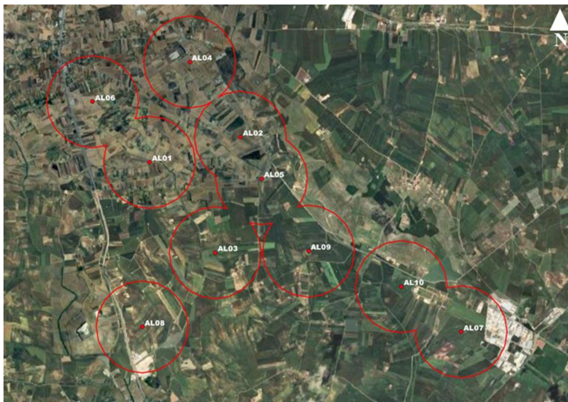
Figura 3-3 Ambito di studio (in rosso) e turbine di progetto
