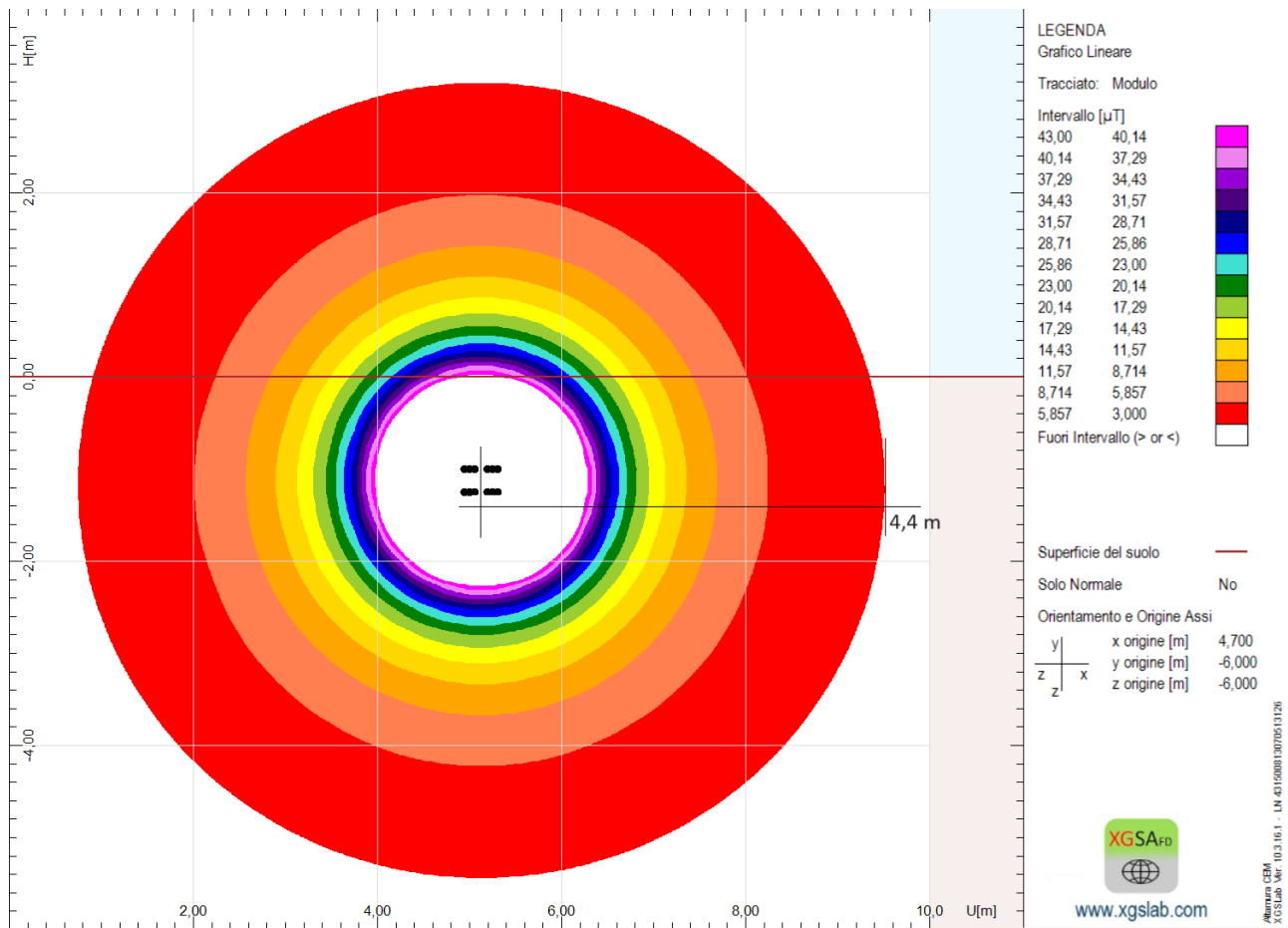
Fig. 1 : andamento del campo di induzione magnetica nel tratto a 4 terne
