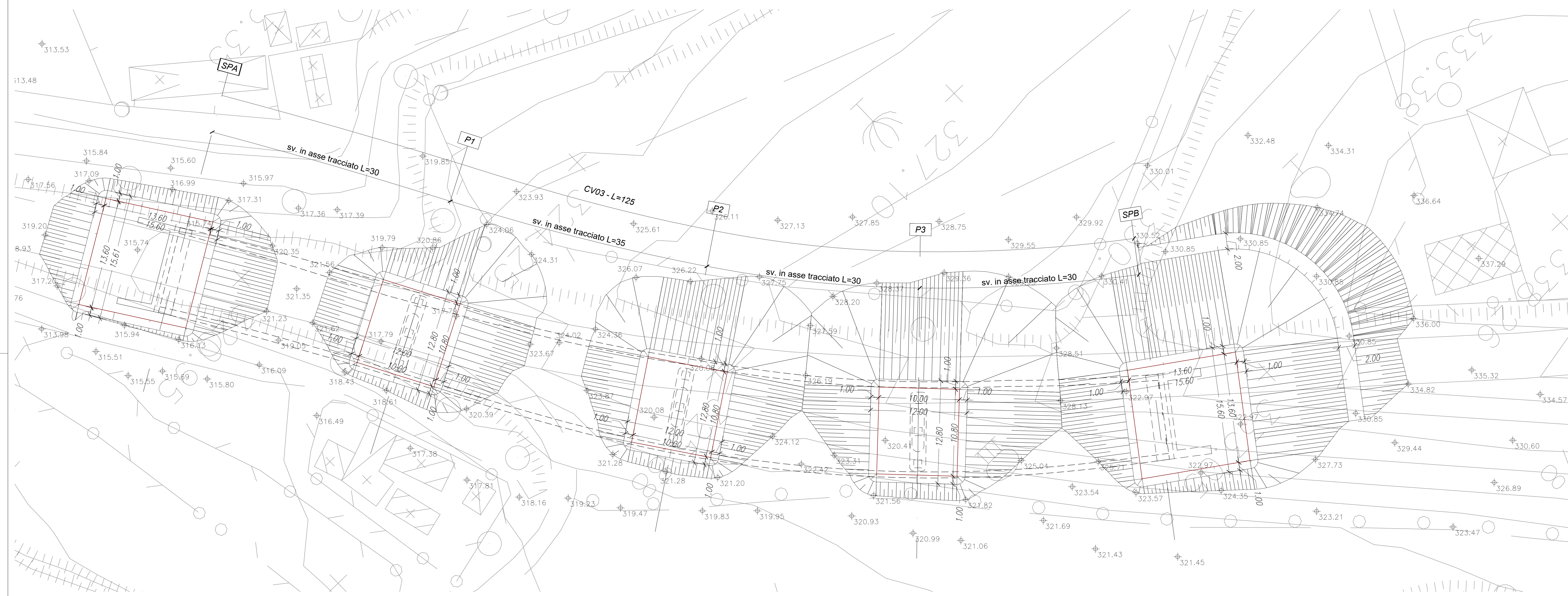
Pianta Scavi - CV03 - Scala 1:200
