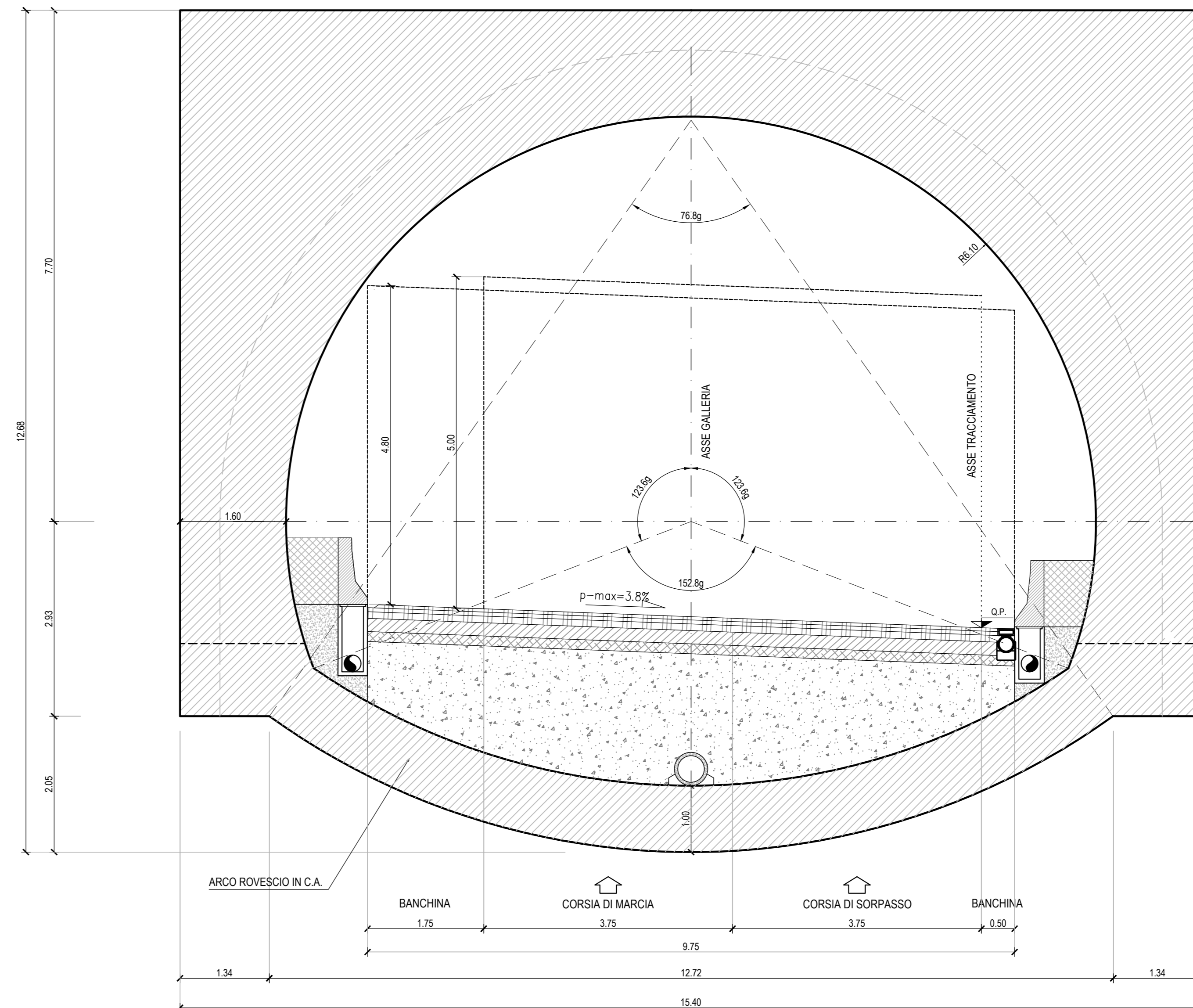
GA04 - MURO FRONTALE SCALA 1:50
