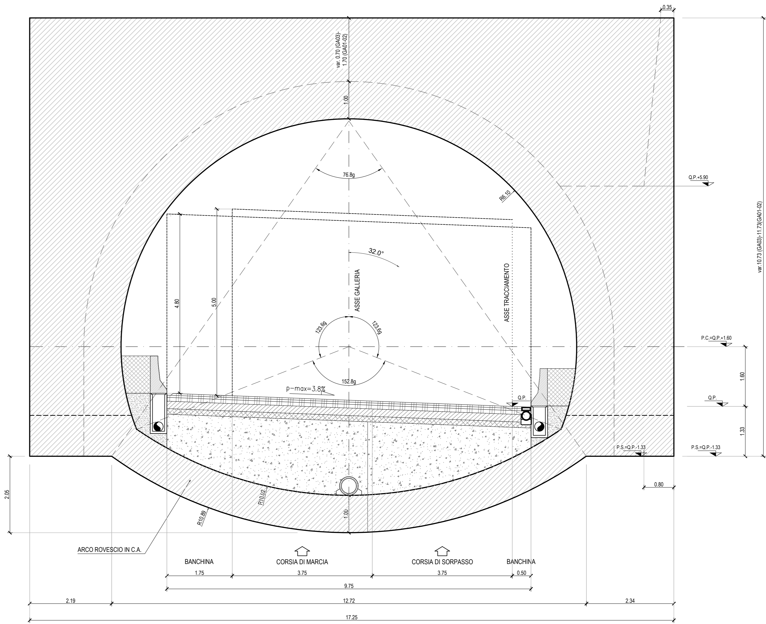
GA01-02-03 - MURO FRONTALE SCALA 1:50
