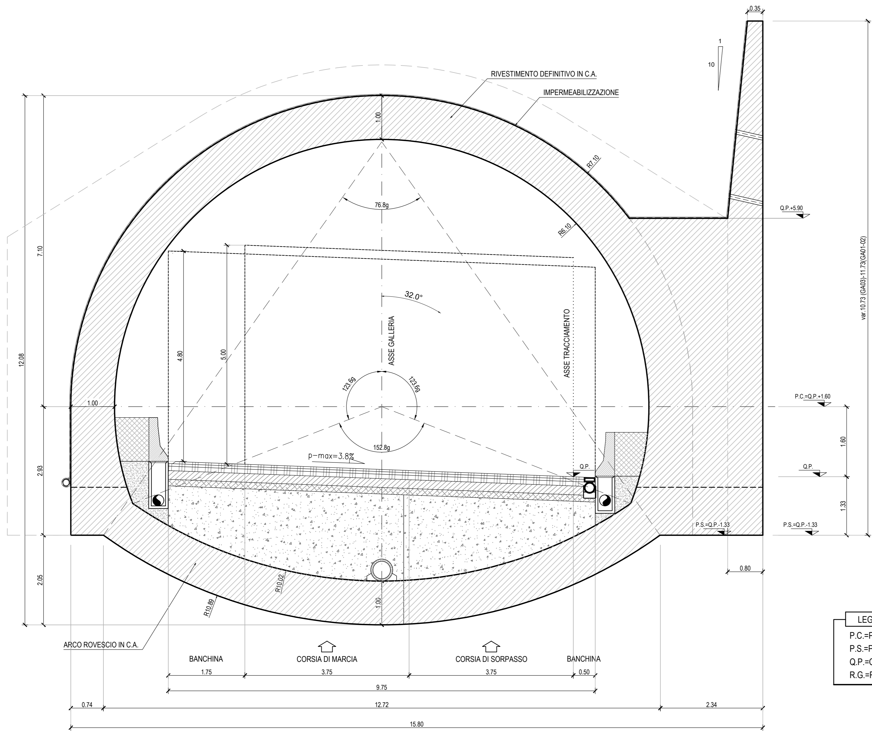
GA01-02-03 - SEZIONE CORRENTE SCALA 1:50
