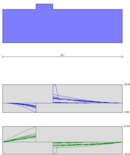
Fig. 10 - Fondazione (Inviluppo)
