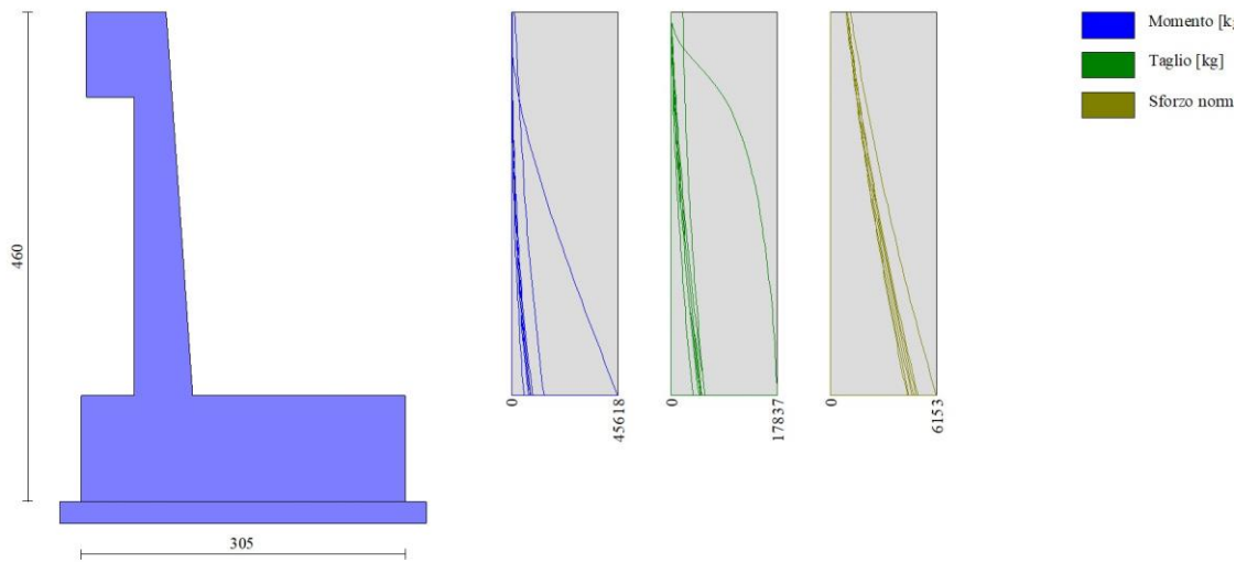
Fig. 8 - Paramento (Inviluppo)
