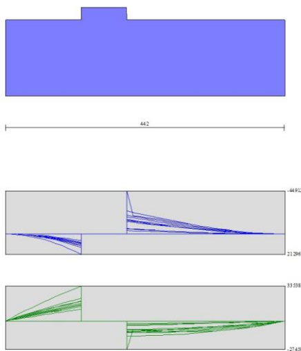
Fig. 10 - Fondazione (Inviluppo)
