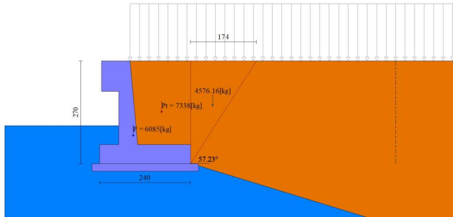
Fig. 6 - Cuneo di spinta (combinazione statica) (Combinazione n° 1)
