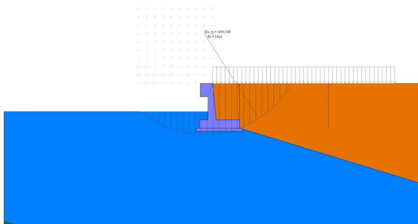
Fig. 18 - Stabilità fronte di scavo - Cerchio critico (Combinazione n° 9)
