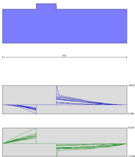
Fig. 16 - Fondazione
