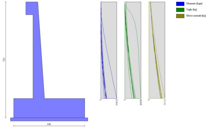
Fig. 8 - Paramento (Inviluppo)
