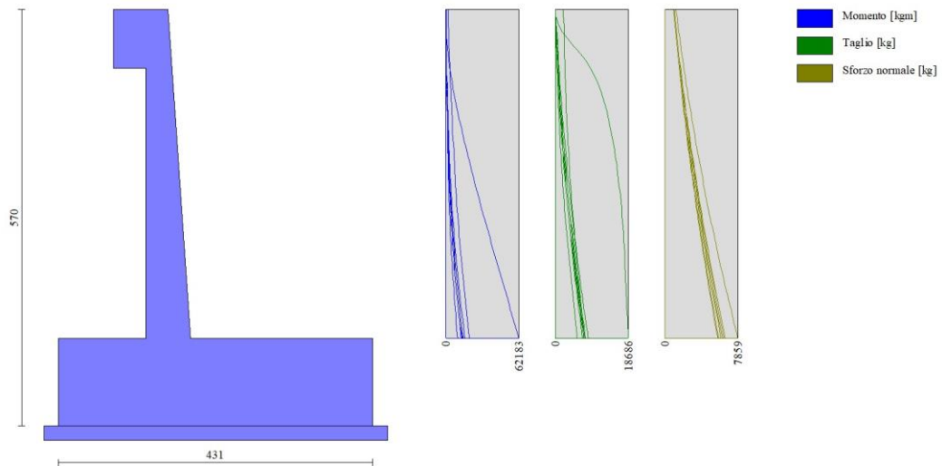
Fig. 8 - Paramento (Inviluppo)
