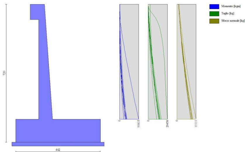
Fig. 14 - Paramento
