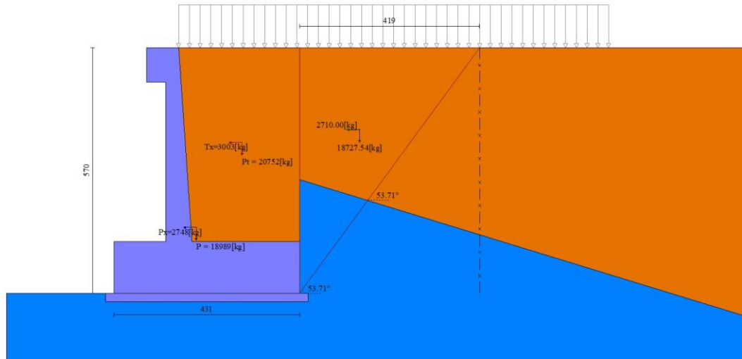
Fig. 11 - Cuneo di spinta (combinazione sismica) (Combinazione n° 2)
