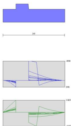
Fig. 13 - Fondazione (Inviluppo)
