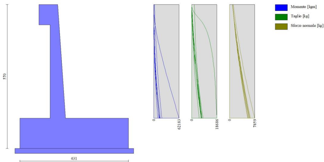
Fig. 14 - Paramento
