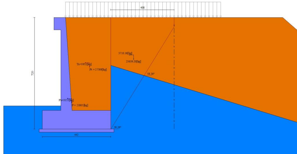
Fig. 11 - Cuneo di spinta (combinazione sismica) (Combinazione n° 2)
