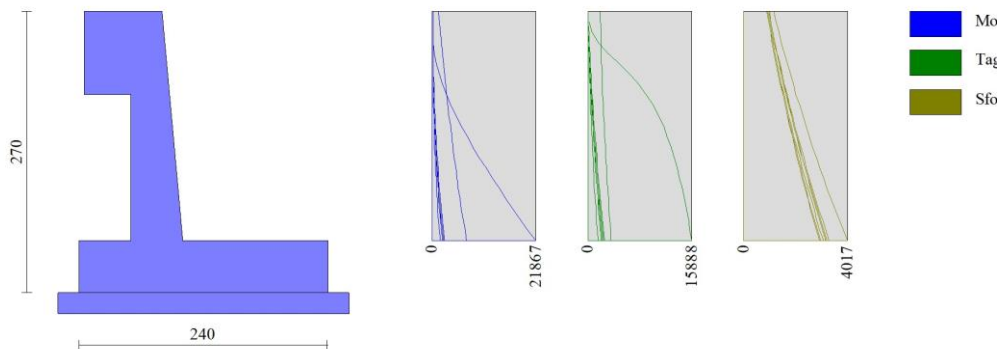
Fig. 19 - Paramento
