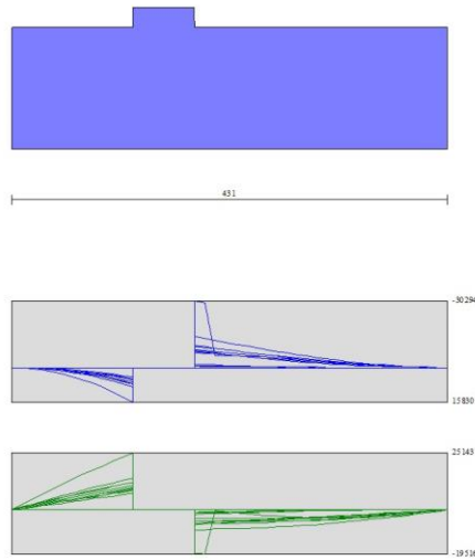
Fig. 16 - Fondazione
