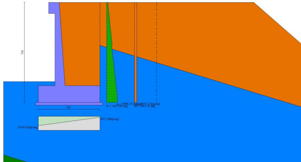
Fig. 12 - Diagramma delle pressioni (combinazione sismica) (Combinazione n° 2)
