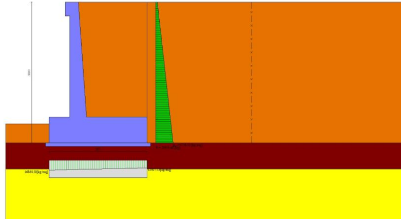
Fig. 12 - Diagramma delle pressioni (combinazione statica) (Combinazione n° 1)
