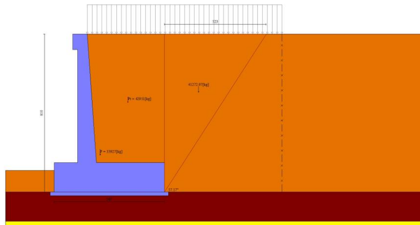
Fig. 11 - Cuneo di spinta (combinazione statica) (Combinazione n° 1)
