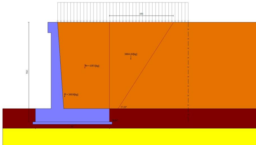
Fig. 6 - Cuneo di spinta (combinazione statica) (Combinazione n° 1)
