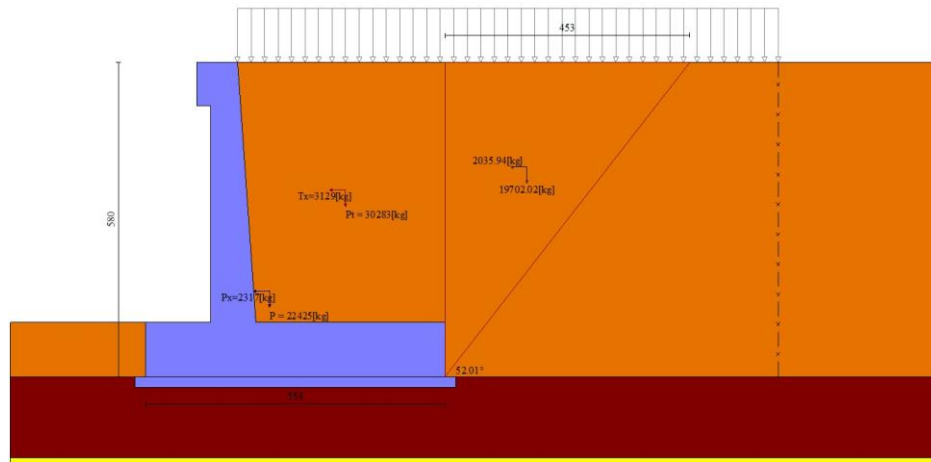
Fig. 8 - Cuneo di spinta (combinazione sismica) (Combinazione n° 2)
