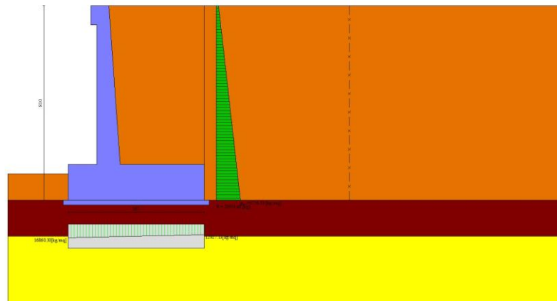
Fig. 4 - Diagramma delle pressioni (combinazione statica) (Combinazione n° 1)
