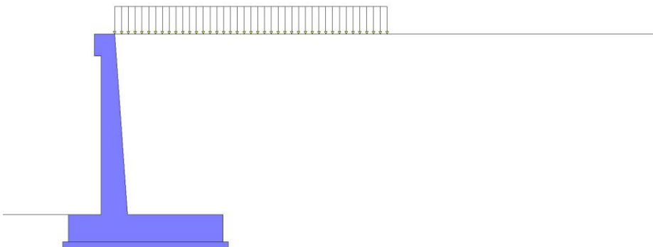
Fig. 5 - Carichi sul terreno
