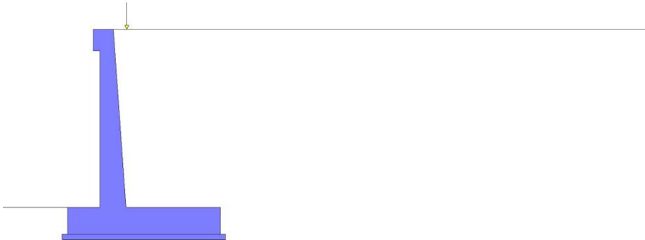
Fig. 4 - Carichi sul terreno
