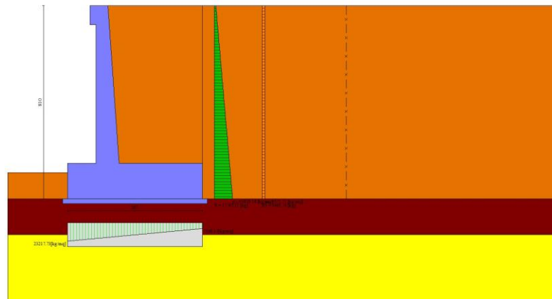
Fig. 6 - Diagramma delle pressioni (combinazione sismica) (Combinazione n° 2)
