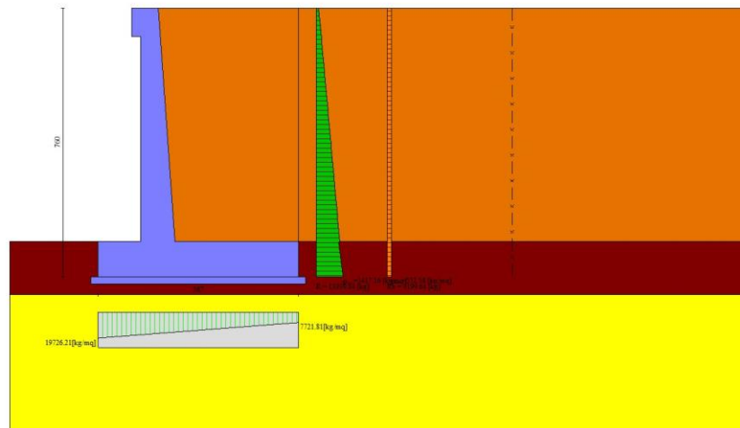
Fig. 9 - Diagramma delle pressioni (combinazione sismica) (Combinazione n° 2)
