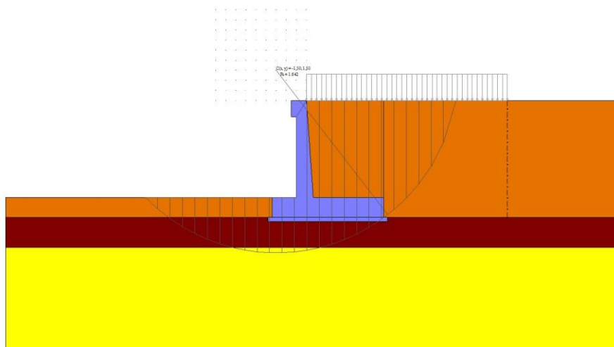
Fig. 10 - Stabilità fronte di scavo - Cerchio critico (Combinazione n° 7)
