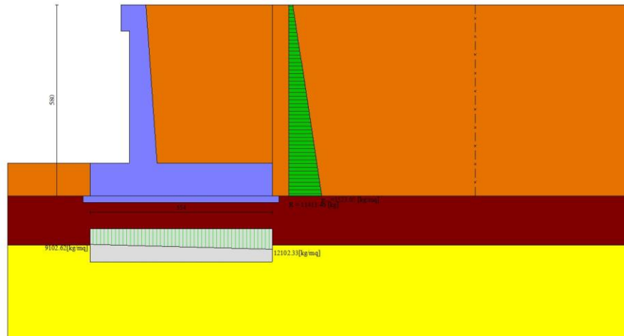
Fig. 15 - Diagramma delle pressioni (combinazione statica) (Combinazione n° 1)
