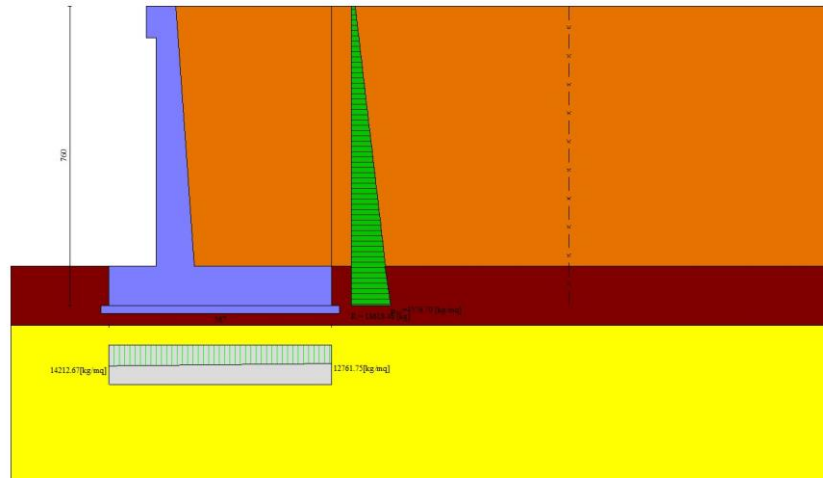
Fig. 15 - Diagramma delle pressioni (combinazione statica) (Combinazione n° 1)
