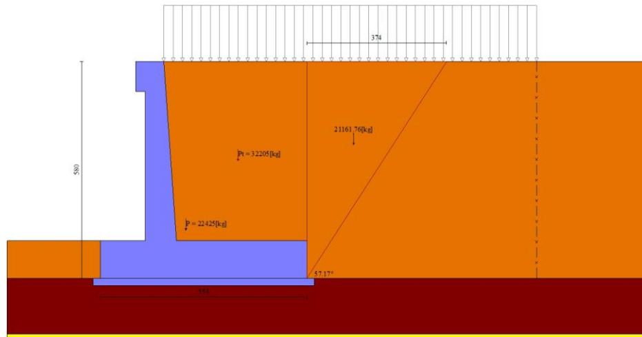
Fig. 6 - Cuneo di spinta (combinazione statica) (Combinazione n° 1)
