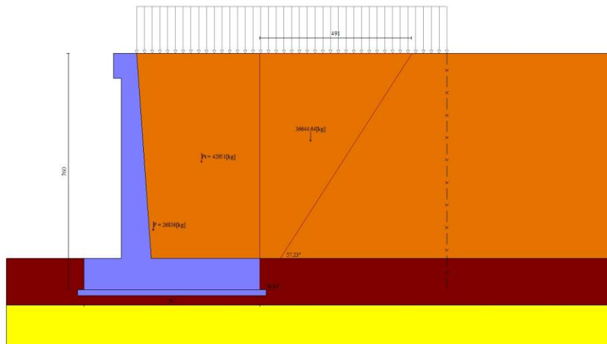
Fig. 14 - Cuneo di spinta (combinazione statica) (Combinazione n° 1)
