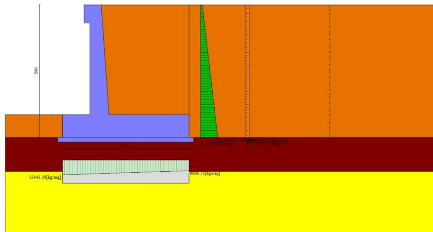
Fig. 9 - Diagramma delle pressioni (combinazione sismica) (Combinazione n° 2)
