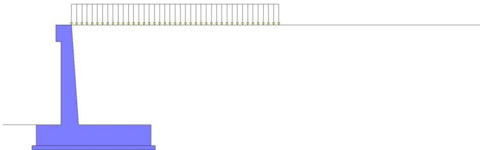
Fig. 5 - Carichi sul terreno
