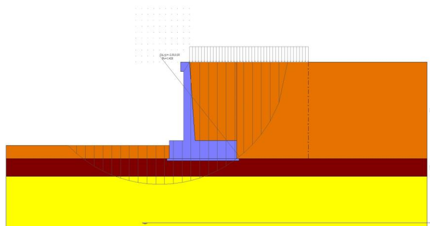
Fig. 13 - Stabilità fronte di scavo - Cerchio critico (Combinazione n° 7)
