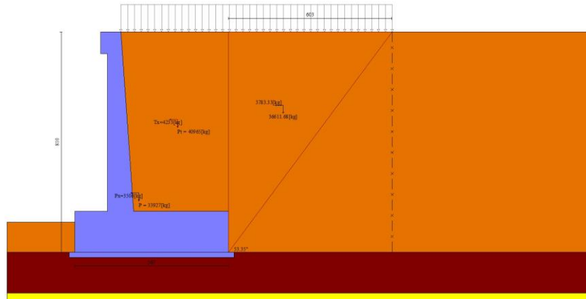
Fig. 5 - Cuneo di spinta (combinazione sismica) (Combinazione n° 2)
