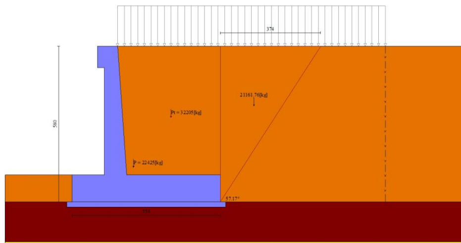
Fig. 14 - Cuneo di spinta (combinazione statica) (Combinazione n° 1)
