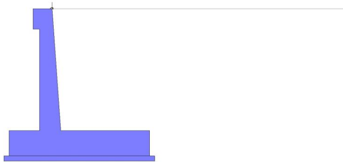
Fig. 3 - Carichi sul muro
