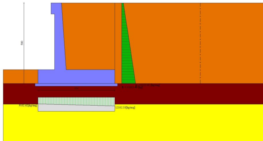
Fig. 7 - Diagramma delle pressioni (combinazione statica) (Combinazione n° 1)
