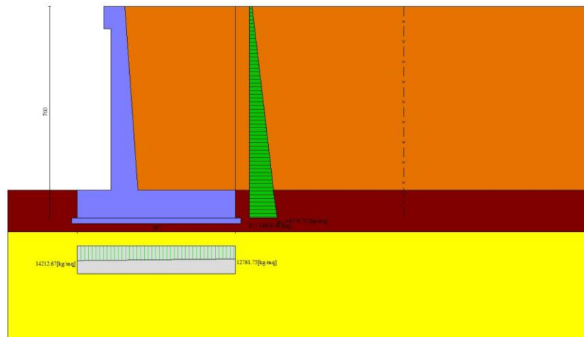
Fig. 7 - Diagramma delle pressioni (combinazione statica) (Combinazione n° 1)
