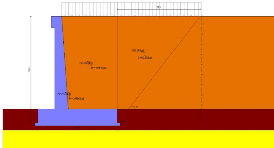
Fig. 8 - Cuneo di spinta (combinazione sismica) (Combinazione n° 2)
