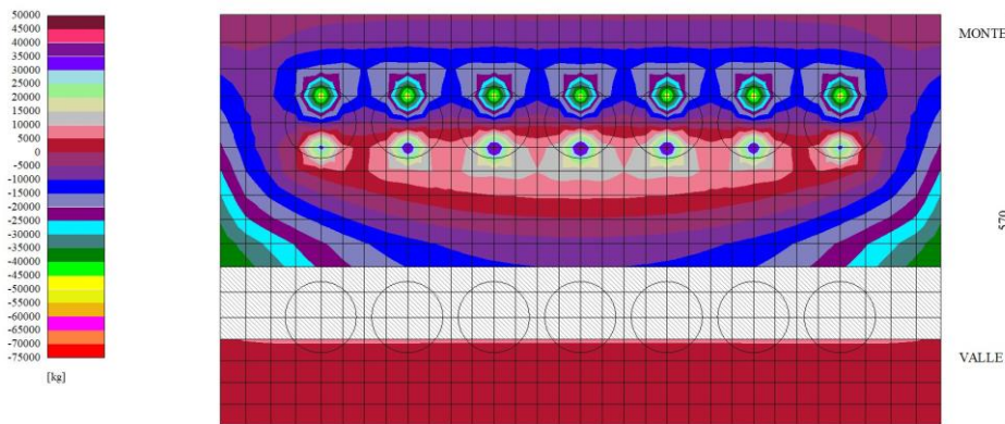
Fig. 34 - Piastra fondazione - Taglio TyMAX (Combinazione n° 4)
