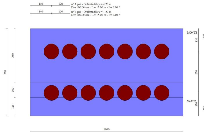
Fig. 2 - Pianta pali
