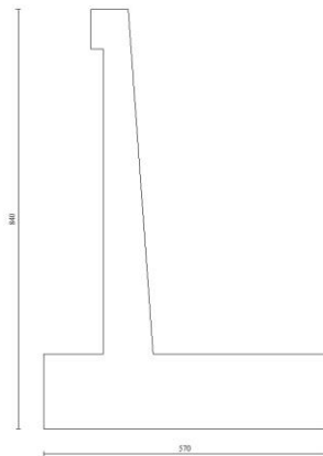
Fig. 38 - Paramento (Inviluppo)
