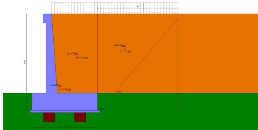
Fig. 27 - Cuneo di spinta (combinazione sismica) (Combinazione n° 2)
