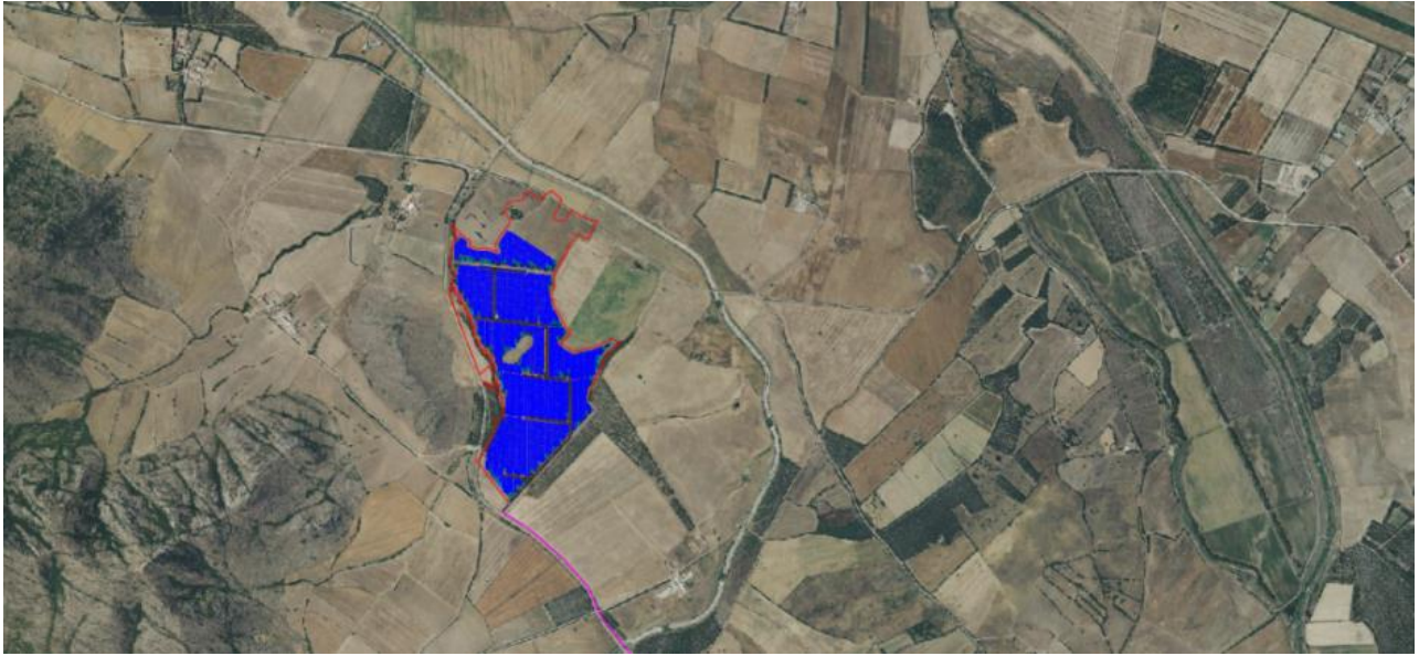
Planimetria delle linee a 36 kV (cavidotti interrati) per il collegamento delle Cabine di Raccolta di Area alla Cabina di Raccolta Generale (C-00). Per ulteriori dettagli si rimanda alle relative tavole di progetto.
