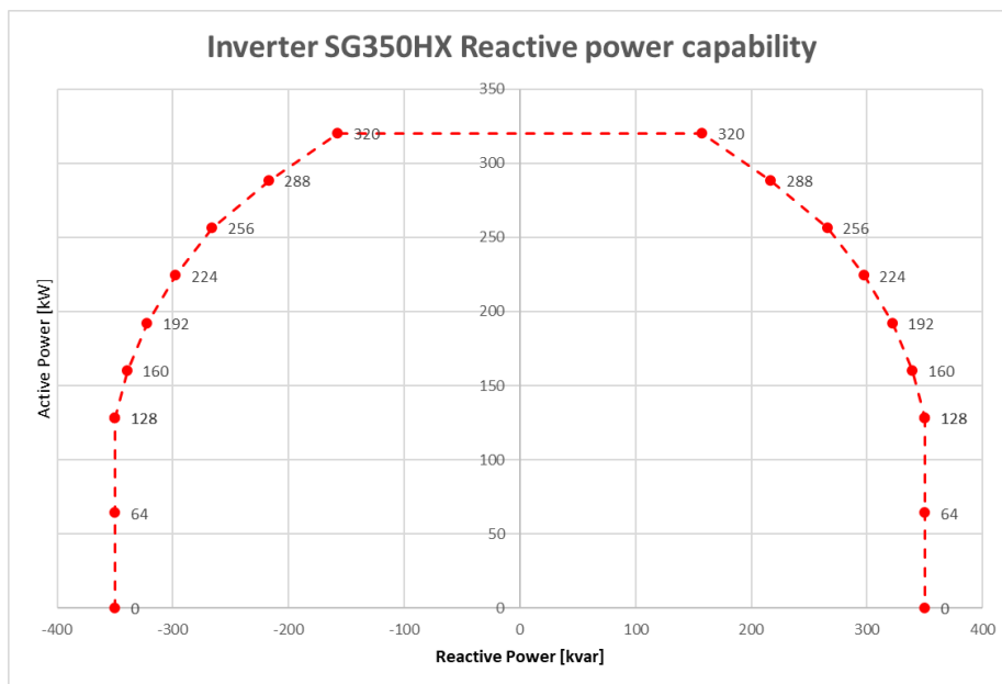
Fig. 2 – Curva di capability P,Q dell’inverter Sungrow SG350HX
