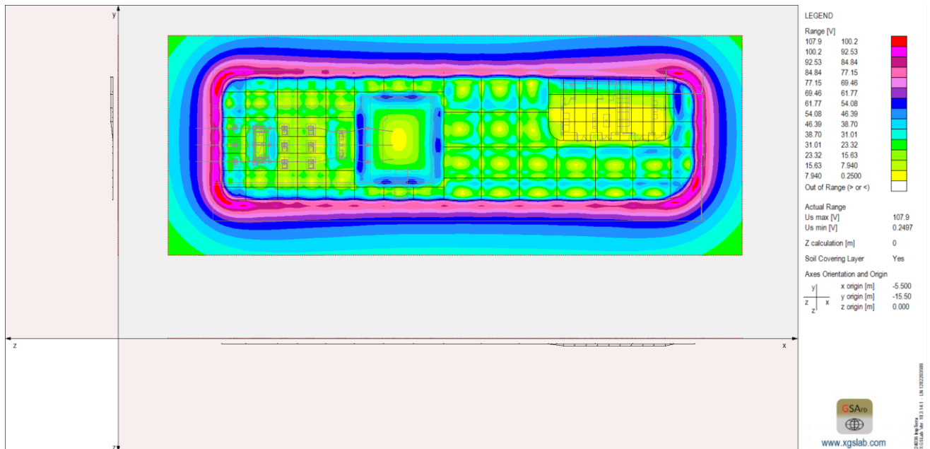
Fig. 12 - Distribuzione delle tensioni di passo (rappresentazione 2D)
