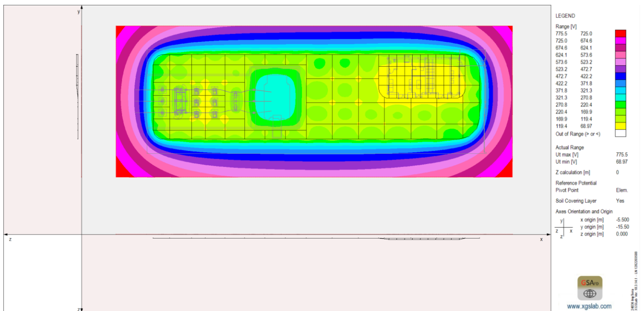
Fig. 11 - Distribuzione delle tensioni di contatto (rappresentazione 2D)
