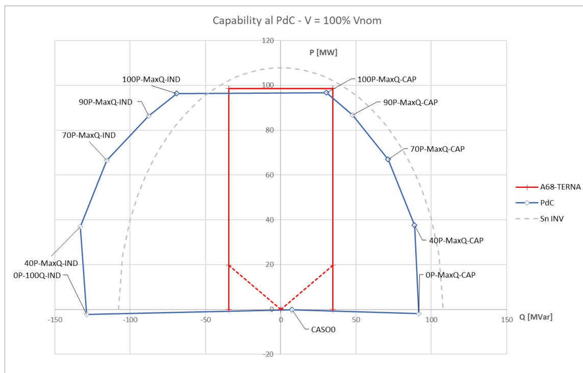
Fig. 3 – Curva di capability al PdC dell’impianto (blu), confrontata con quella richiesta dall’Allegato A.68 al CdR (rossa)
