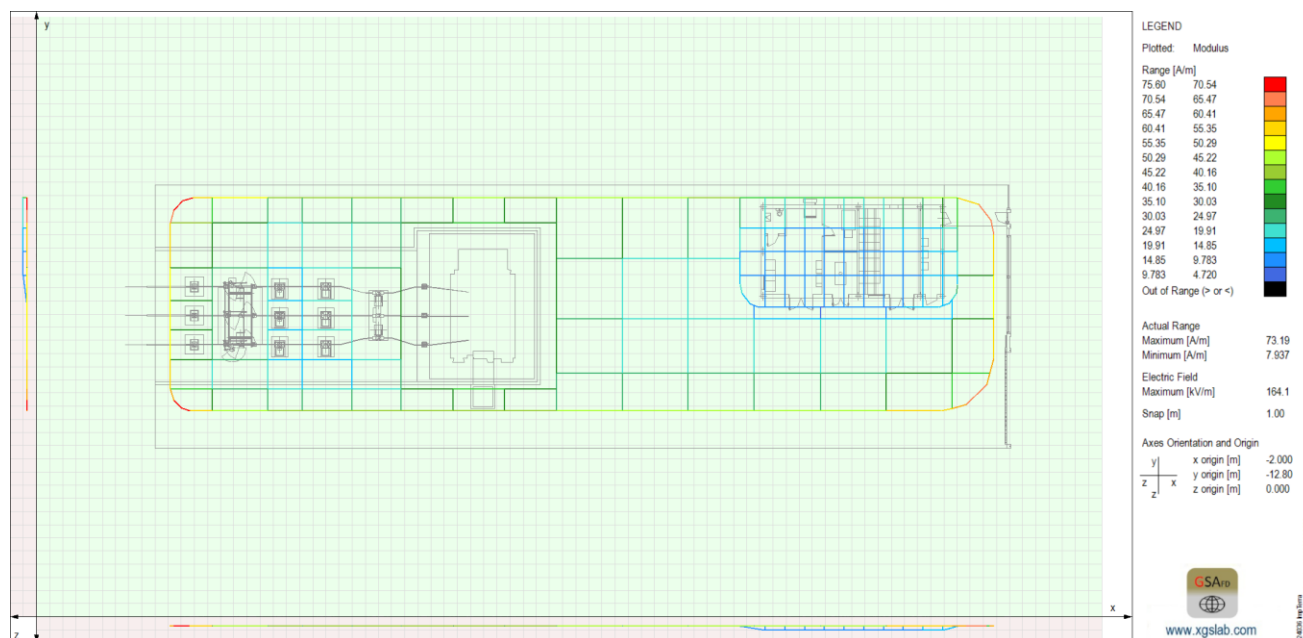
Fig. 8 - Distribuzione della densità di corrente dispersa
