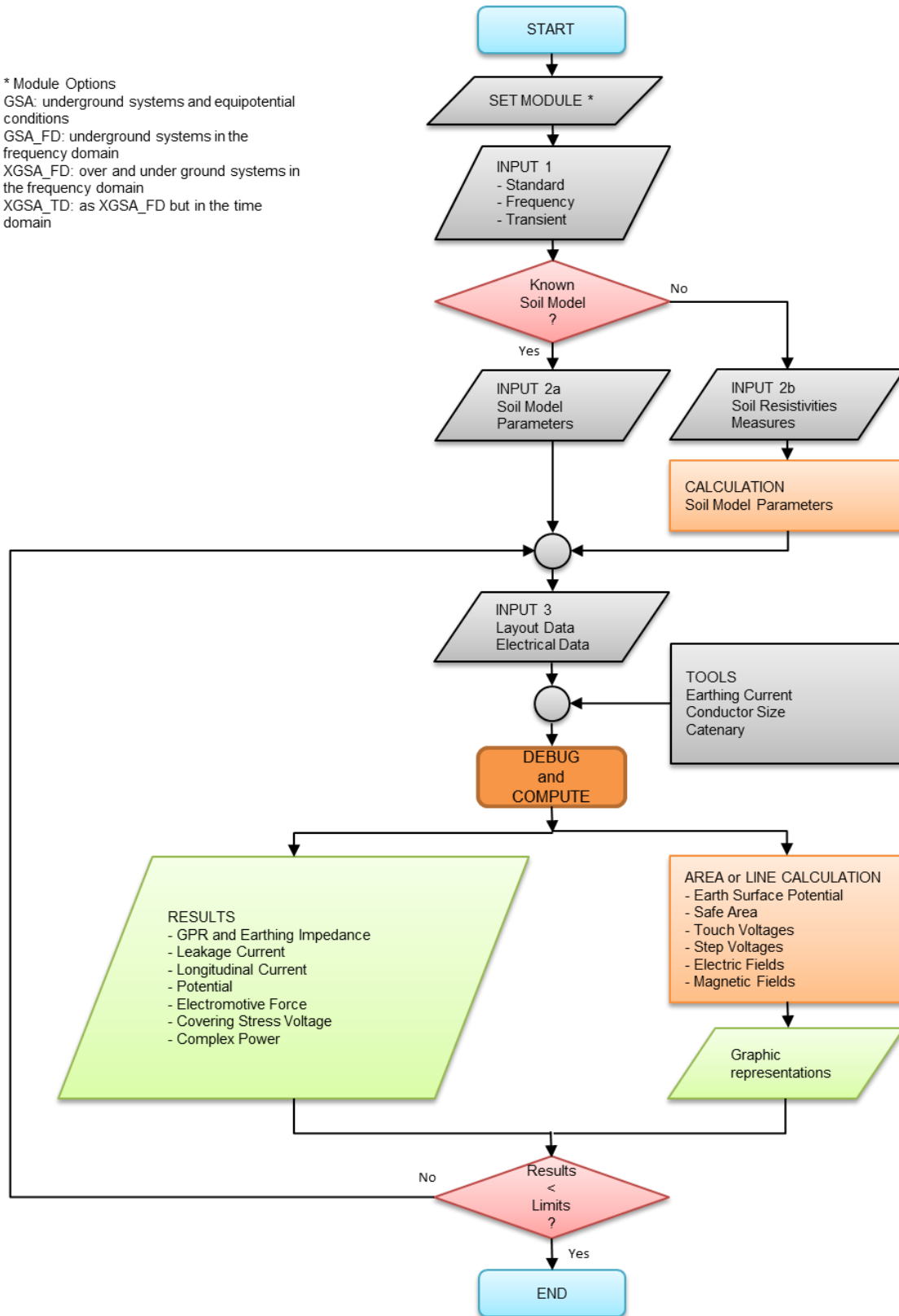
Fig. 4 - Diagramma di flusso di XGSLabDATI
