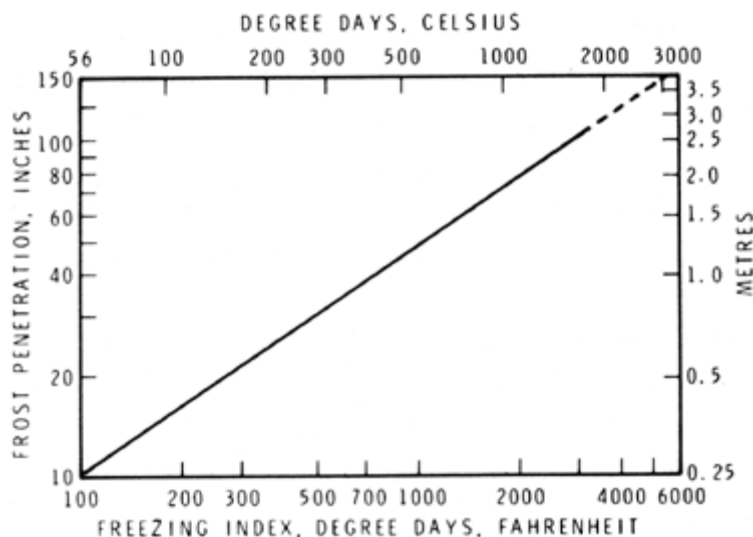
Fig. 6 - Relazione tra indice di congelamento e massima profondità di congelamento del terreno
