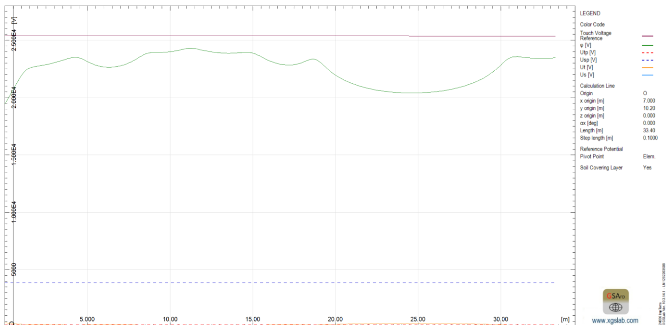
Fig. 14 - Tensioni di contatto e di passo lungo la direttrice di calcolo considerando lo strato superficiale
