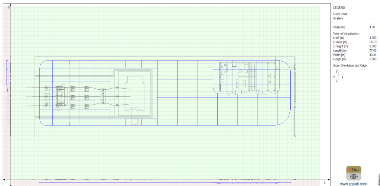
Fig. 7 - Layout del sistema dispersente
