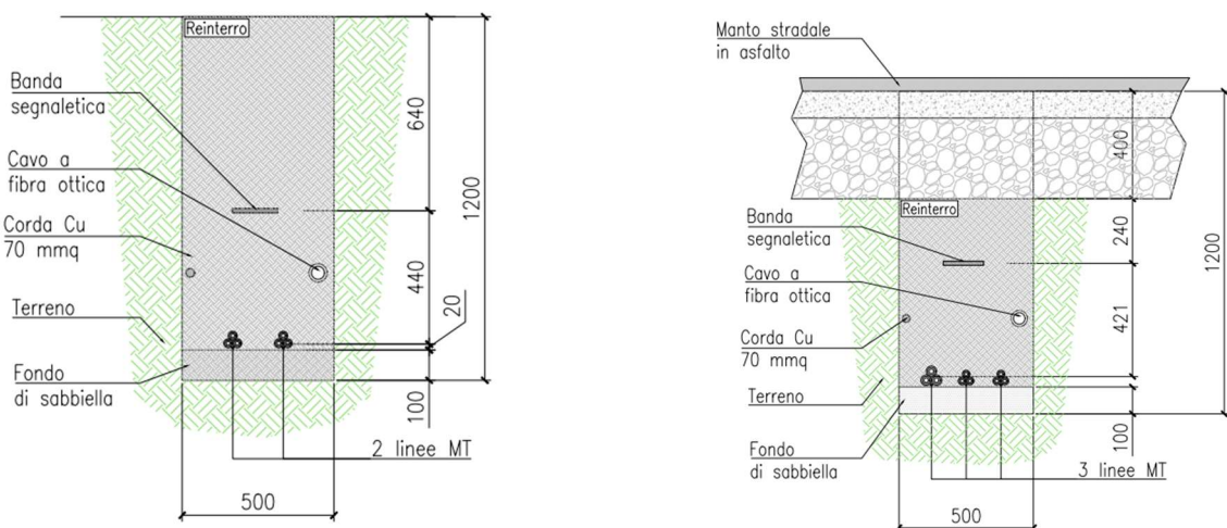
Figure 8 – Sezioni posa cavidotto 'SECUZIONE DEI MOVIMENTI TERRA
