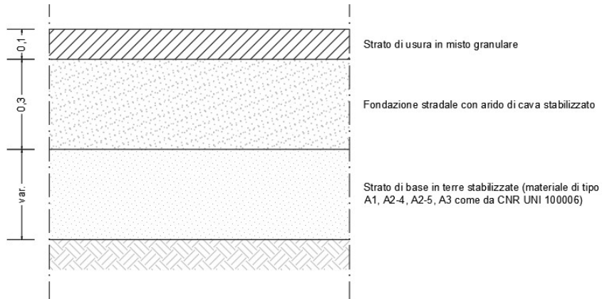
Figure 4 - Stratigrafia stradale
