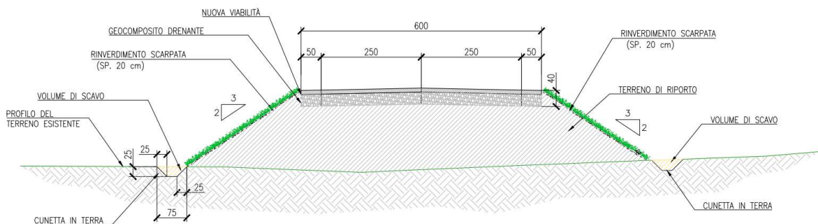
Figure 3- Tipologica sezione stradale
