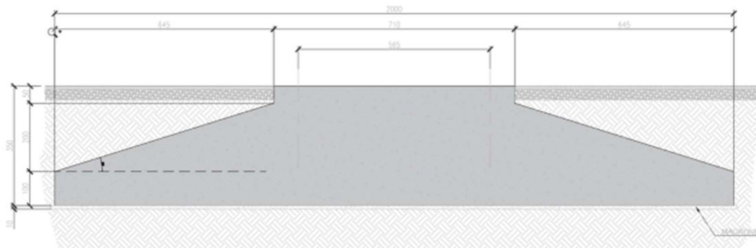
Figure 7 – Fondazione superficiale
