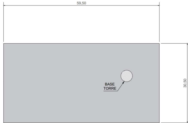
Figure 5 - Layout piazzole rispettivamente in fase di cantiere ed in fase di esercizio
