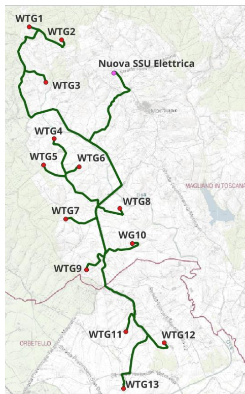
Figura 3: Ubicazione del cavidotto e della SSU
