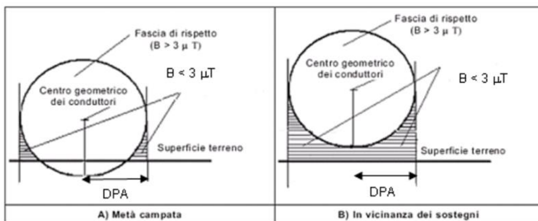
Figura 1: Schema Fasce rispetto e DPA in corrispondenza di metà campata e in vicinanza dei sostegni.
