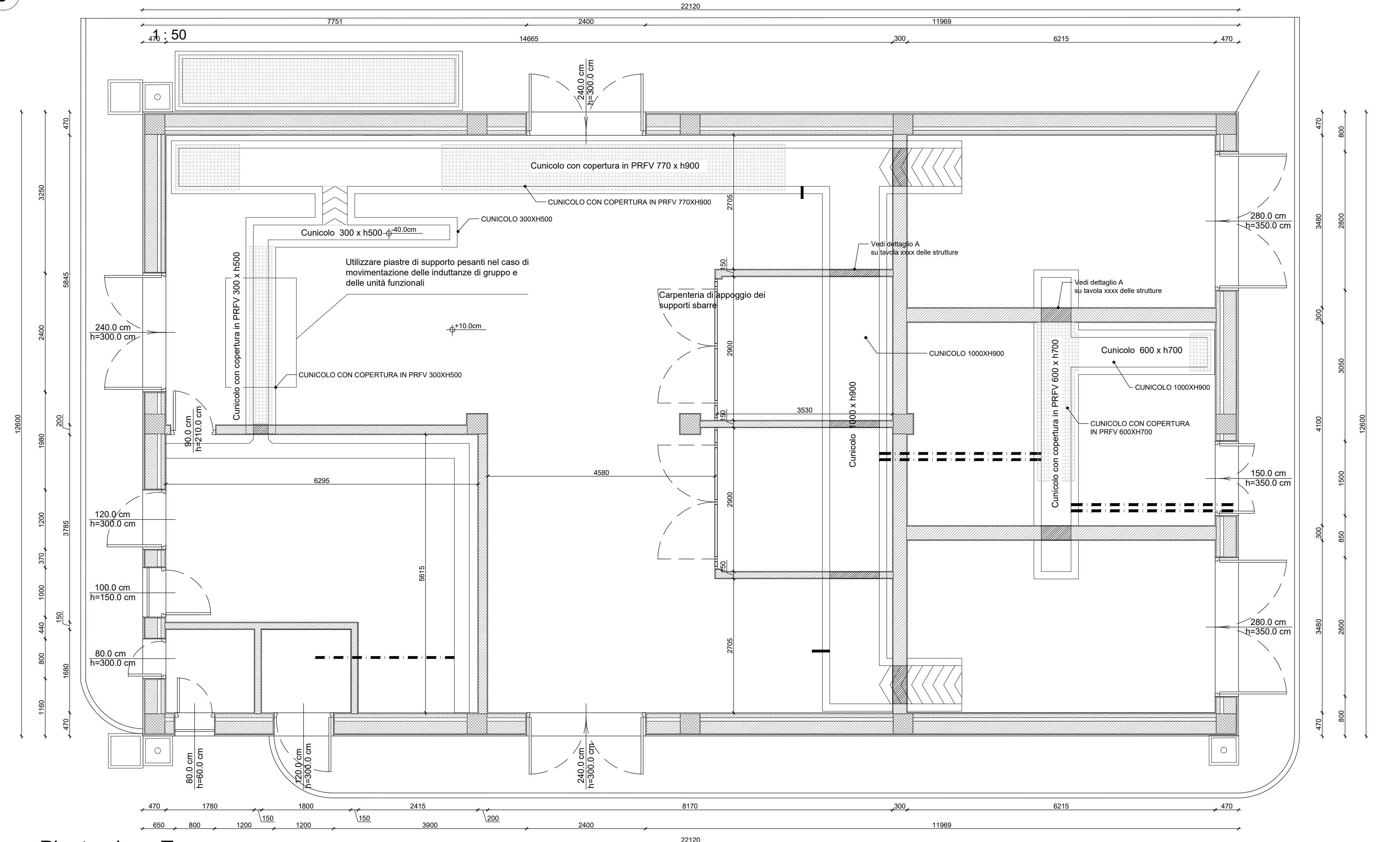
1 Pianta piano Terra 1 : 50
