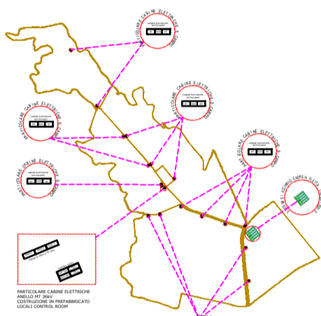
AREE IMPIANTO FOTOVOLTAICO MAPPA VIABILITA' INTERNA E DISTRIBUZIONE CABINE ELETTRICHE
