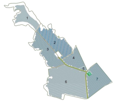
VISTA COMPLESSIVA SUPERFICI IMPIANTO FOTOVOLTAICO IN PROGETTO
