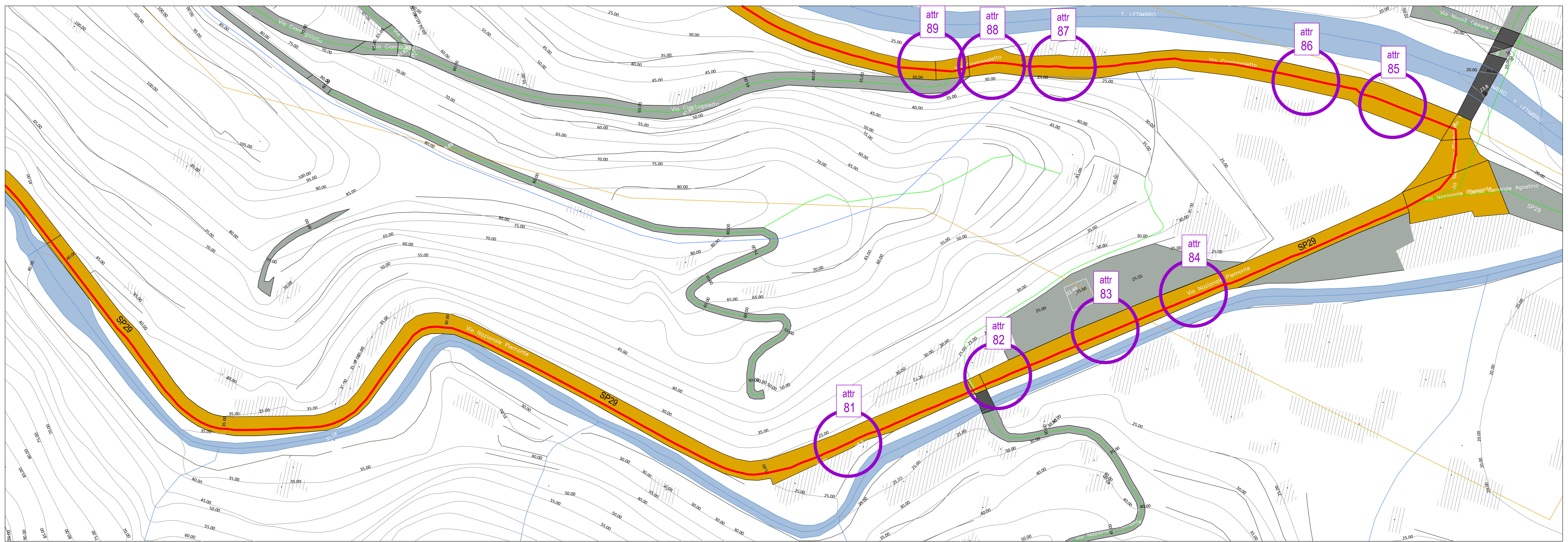
PLANIMETRIA DI INTERVENTO 17 base CTR - scala 1:1000
