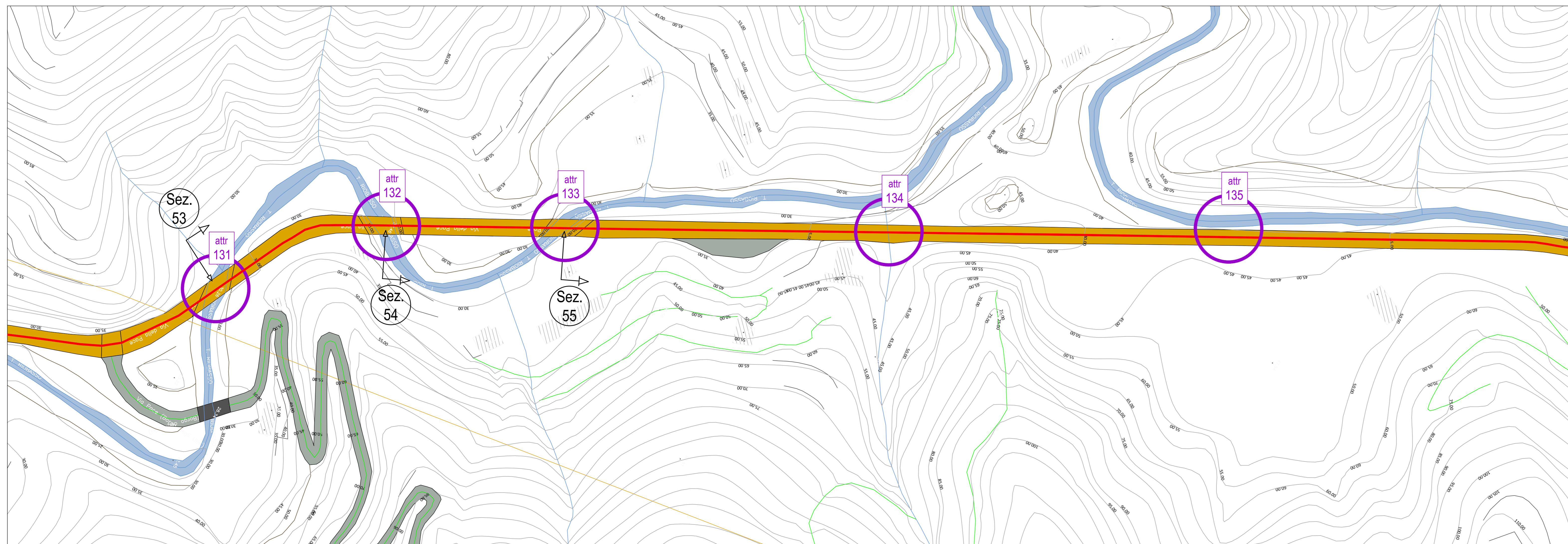
PLANIMETRIA DI INTERVENTO 28 base CTR - scala 1:1000
