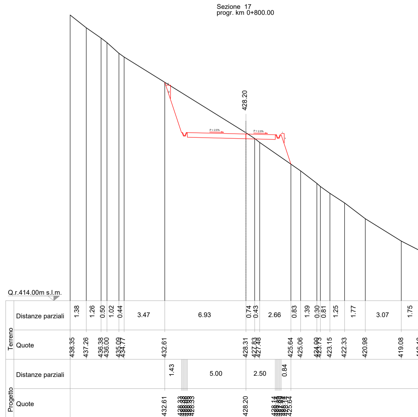
Sezione 17 prog. km 0+800.00
