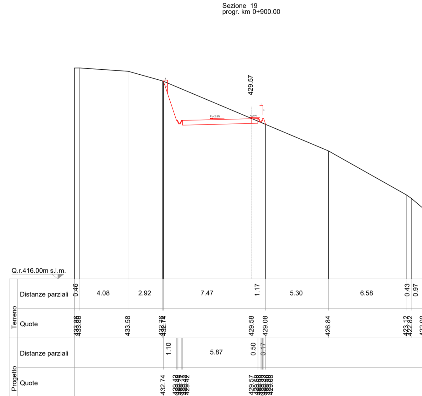
Sezione 19 prog. km 0+900.00
