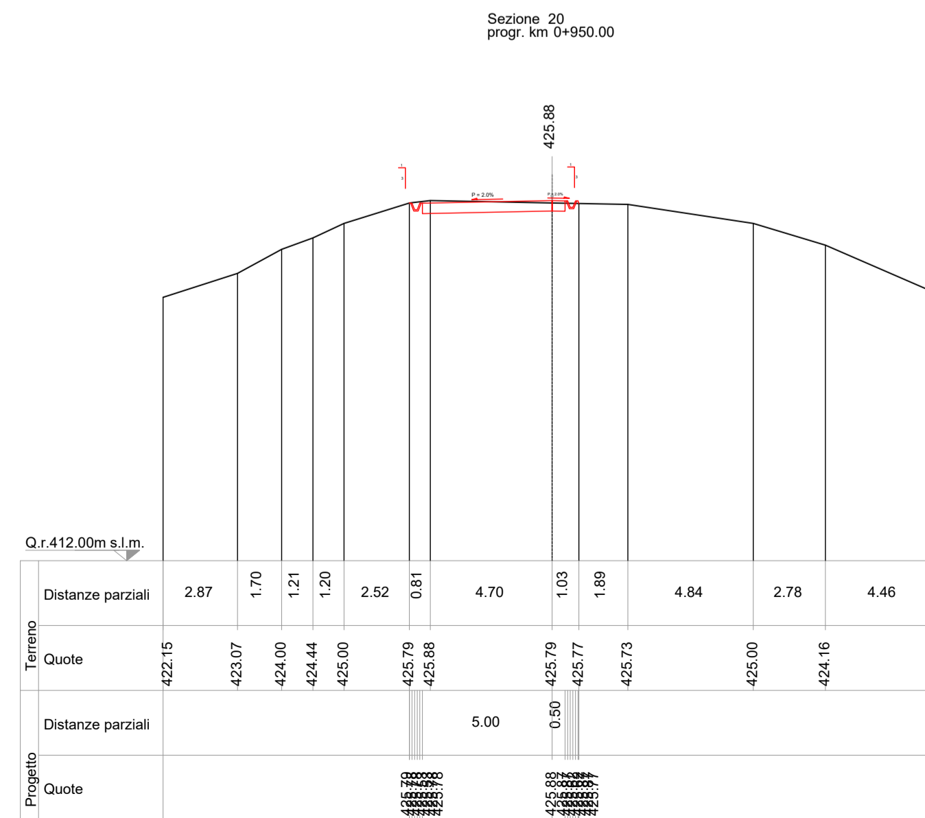
Sezione 20 prog. km 0+950.00
