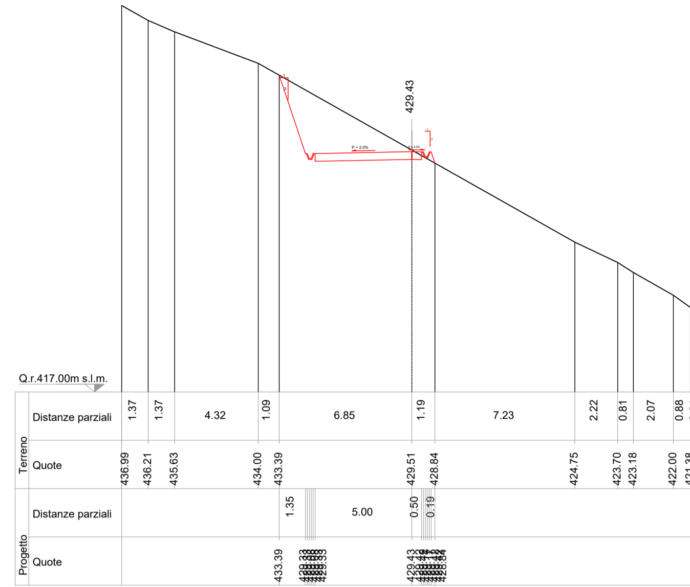
Sezione 18 prog. km 0+850.00
