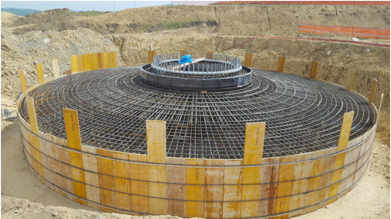
Figura 4 | Strutture di fondazione degli aerogeneratori
