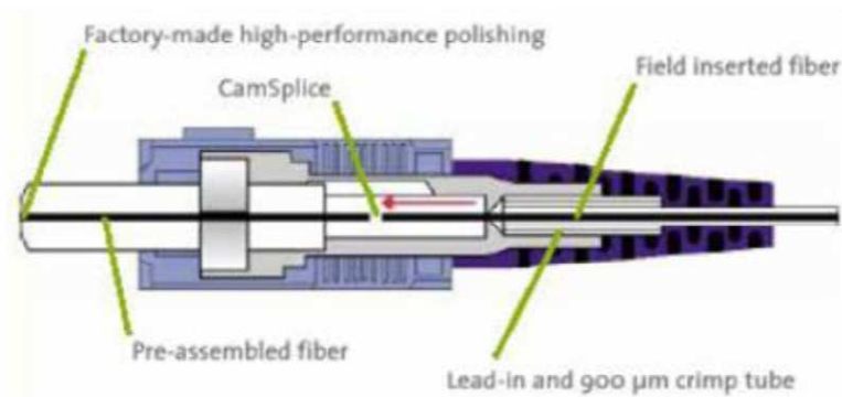
Figura 7 | Connettore ST
